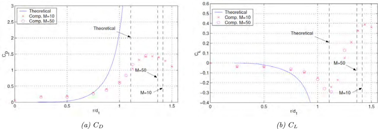
FIGURE 9.10 – Comparaison des coefficients de traînée et de portance obtenus par la méthode Sedov-Laurence (-) avec les résultats numériques AMROC pour la sphère en gaz parfait ( \gamma = 1.4 ), à M = 10 ( \times ) et M = 50 ( \circ ). Figure extraite de [127].
