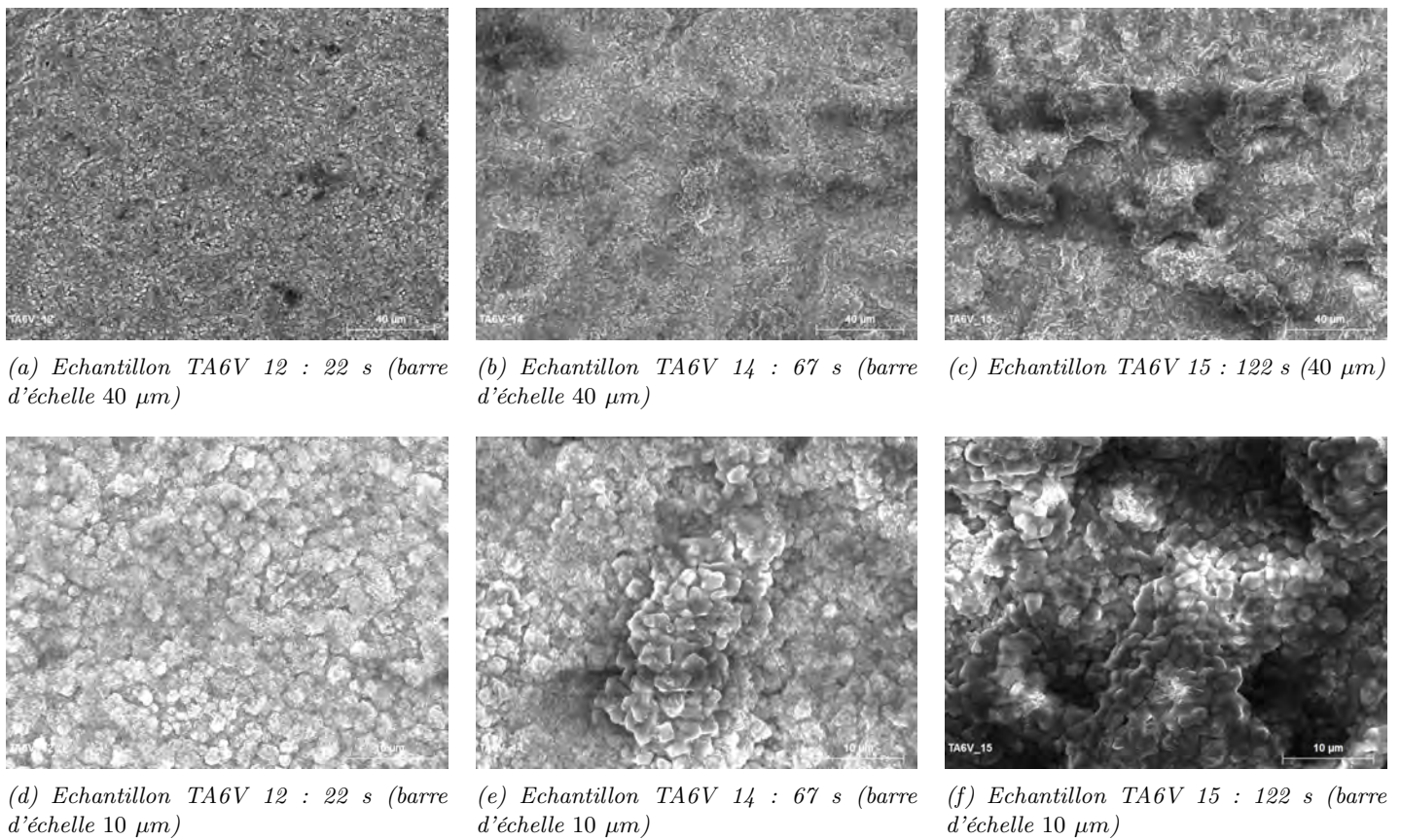
FIGURE 7.17 – Micrographies MEB des surfaces des échantillons oxydés sous plasma d'air à une température d'environ 1700 K pour différents temps d'exposition.
