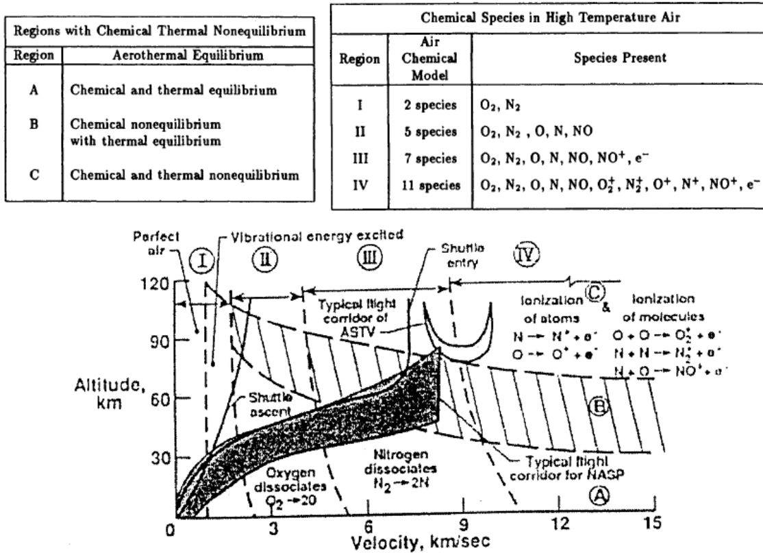
FIGURE 2.20 – Caractérisation thermo-chimique d'un écoulement d'air autour d'une sphère de 30.5 cm de rayon, d'après [19].
