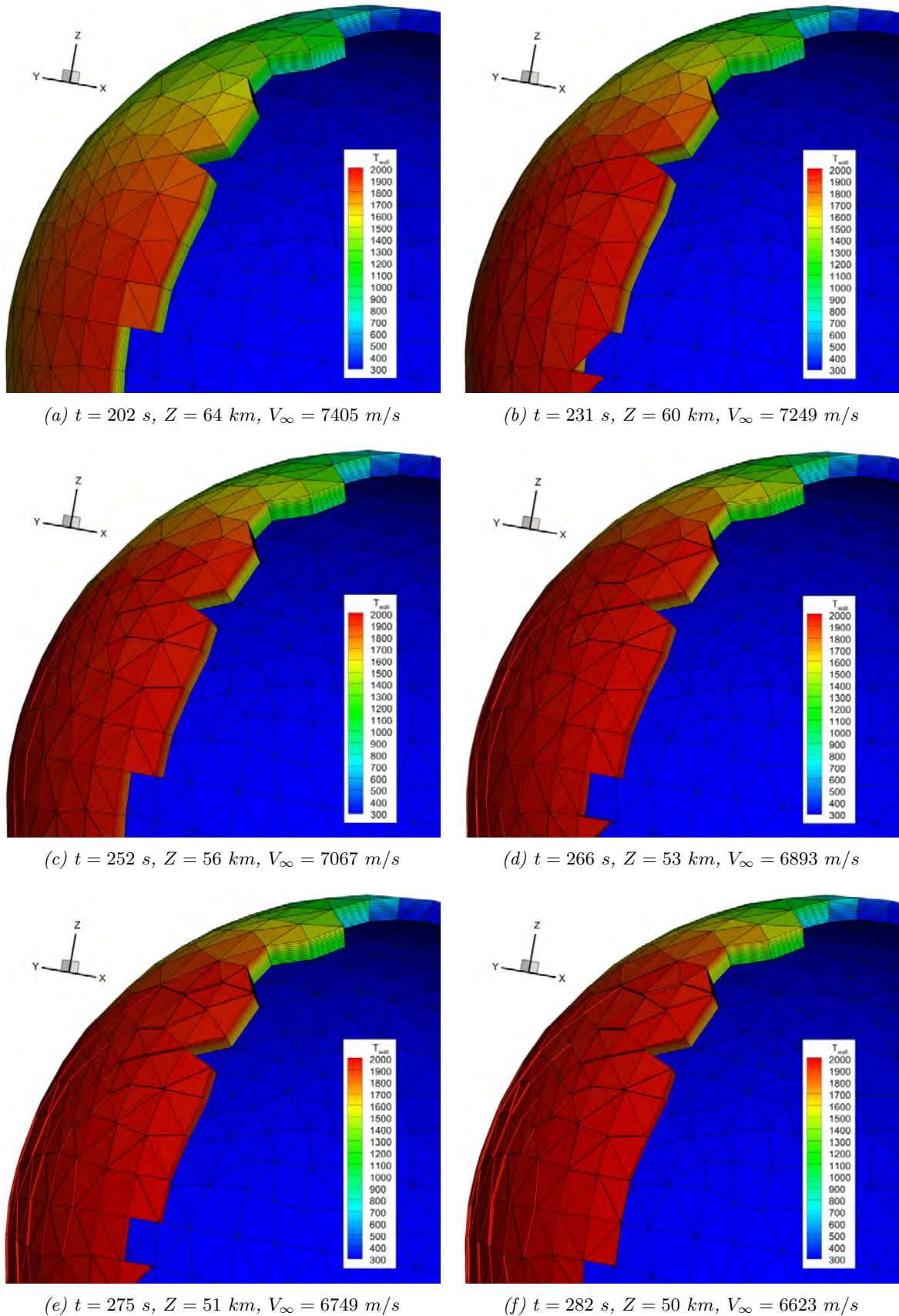
FIGURE 10.10 – Dégradation thermique de la paroi relevée en différents instants de la trajectoire (Cas 3).
