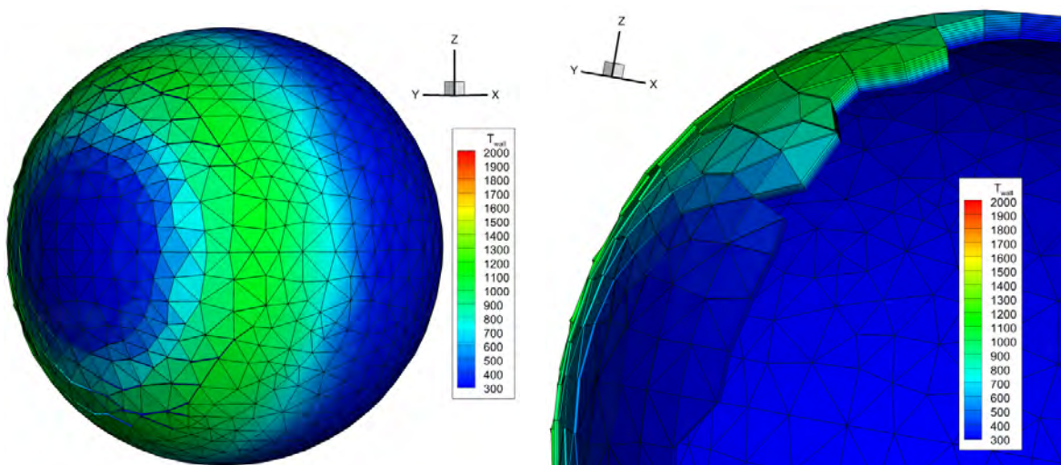
(e) t = 390 \text{ s} , Z = 16 \text{ km} , V_\infty = 665 \text{ m/s} , distribution surfacique de température
