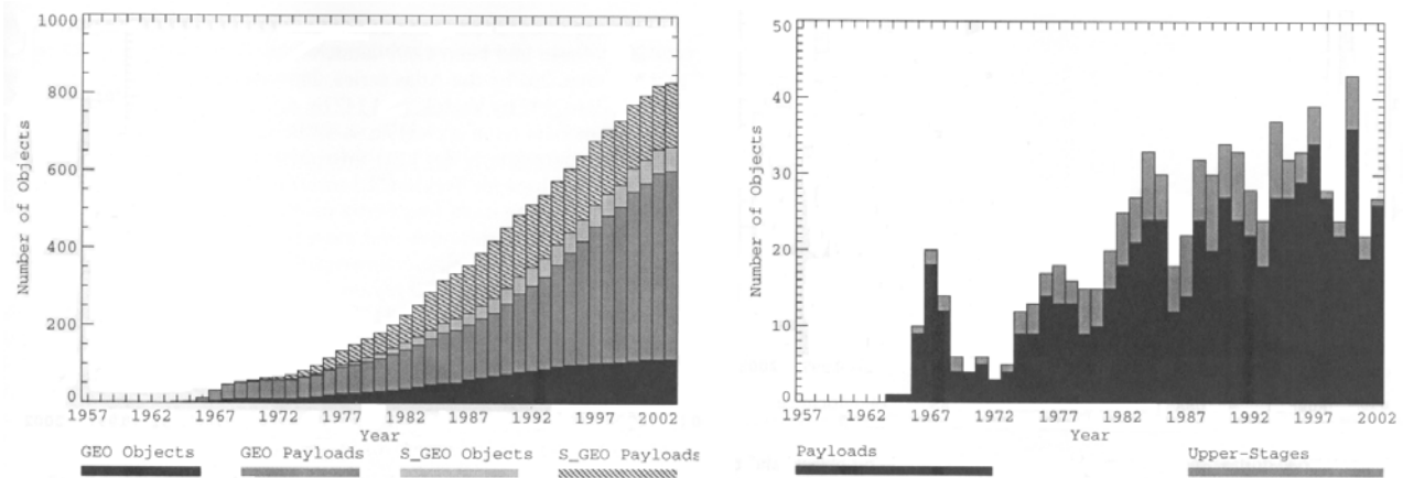
(a) Évolution annuelle du nombre d'objets, catalogués et traçables, en GEO et super-GEO suivant leur origine (Charge utile ou étage supérieur de lanceurs), (source : [110]).
