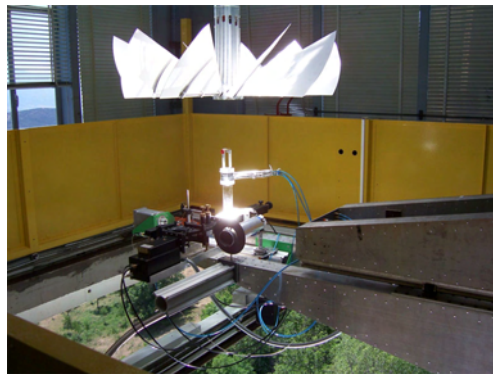
(a) Dispositif expérimental MESOX, (Source : CNRS/PROMES).
