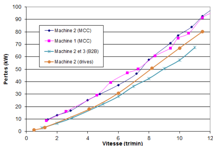
Figure 5.29 Comparaison des pertes à vide en fonction des essais
