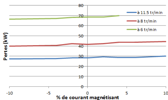
Figure 5.30 Variation des pertes en fonction du courant magnétisant (exprimé en pourcentage du courant nominal)
