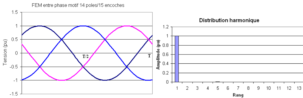
Figure 3.18 FEMs et analyse spectrale d'une machine à 15 encoches/14 pôles
