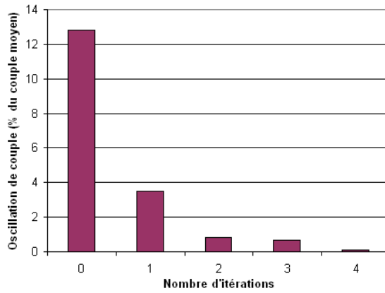
Figure 4.27 Évolution des ondulations de couple en fonction du nombre d'itérations
