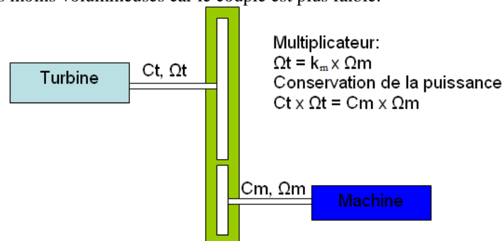
Figure 1.20 Principe du multiplicateur de vitesse
