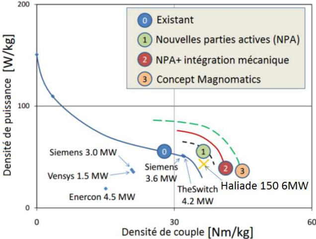
Figure 5.48 Comparaison des densités de couple des génératrices éoliennes [Mat11]
