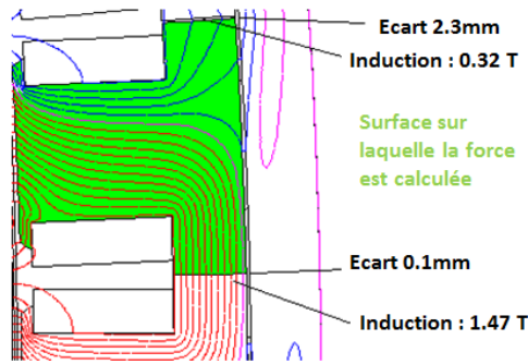
Figure 5.8 Lignes de champ dans un plot
