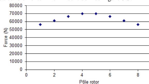
Figure 5.5 Effort normal vu par chaque pôle du motif à instant donné (Cas couple nominal)
