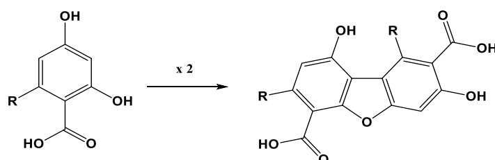
Figure 23 : Biogenèse des dibenzofuranes par couplage de deux unités de type acide orsellinique.
