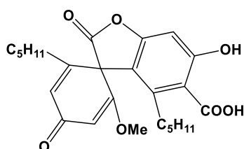
Figure 21 : Exemple de depsones, l'acide picrolichénique.
