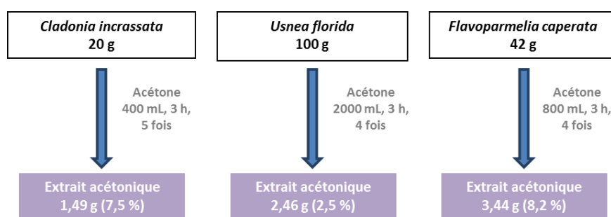
Figure 76 : Schéma d'extraction des lichens. Masses des extraits obtenus (g) et pourcentages d'extraction (%).
