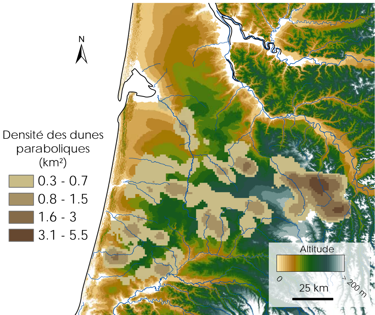
Fig. III.44 : Carte de densité des dunes paraboliques des Landes de Gascogne. N_{\text{tot}} = 2636
