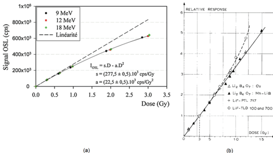
FIGURE 1.18 – Linéarité des a) dosimètres OSL ( Al_2O_3 ); b) dosimètres TLD (LiF et Li_2B_4O_7 ) en fonction de la dose [89, 91].
