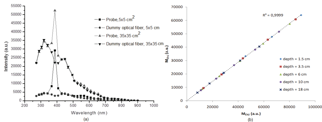
FIGURE 1.25 – a) Spectre du signal de luminescence pour une fibre nue et pour une sonde GaN b) ratio des contributions du signal de luminescence d'une fibre nue dans les canaux CH1 et CH2 respectivement [7].
