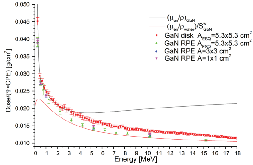
FIGURE 2.15 – Dose dans le transducteur GaN normalisée par la fluence énergétique et par le facteur d'équilibre électronique CPE^w(A, E) .
