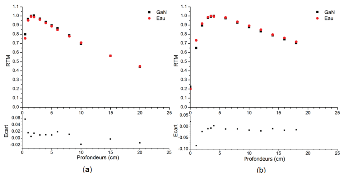
FIGURE 2.4 – RTM mesurés par radioluminescence du GaN et par une chambre d'ionisation pour des faisceaux a) de 6 MV dans un champ carré de 3 \times 3 \text{ cm}^2 et b) de 18 MV dans un champ carré de 5 \times 5 \text{ cm}^2 .
