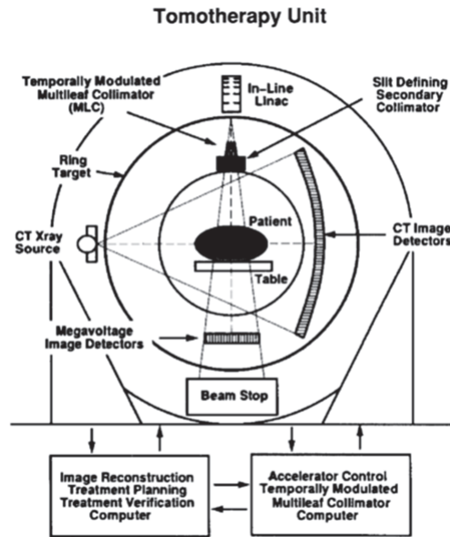
FIGURE 1.6 – Schéma de principe d'une unité de tomothérapie hélicoïdale [27].
