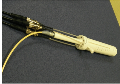
FIGURE 4.26 – Applicateur gynécologique instrumenté avec 4 sondes GaN développé dans le cadre de la thèse de Pierrick Guiral.
