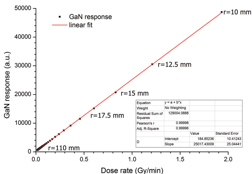
FIGURE 4.5 – Dépendance de la réponse dosimétrique du GaN au débit de dose mesurée pour une source 192 Ir HDR.
