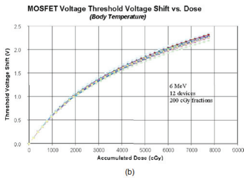
FIGURE 1.22 – linéarité de réponse de la réponse dosimétrique en radiothérapie externe (photon 6 MV) a) du dosimètre GaN ; b) du dosimètre MOSFET ; et c) du dosimètre temps réel \text{Al}_2\text{O}_3 : \text{C} [89].
