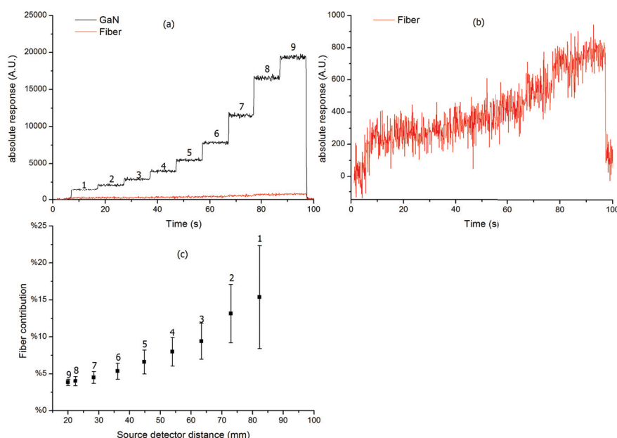
FIGURE 4.6 – a) Réponses d’une sonde GaN et d’une fibre nue en fonction du temps pour 9 positions d’exposition planifiées ; b) zoom sur la réponse de la fibre nue ; c) Contribution de la fibre dans le signal de luminescence de la sonde GaN.
