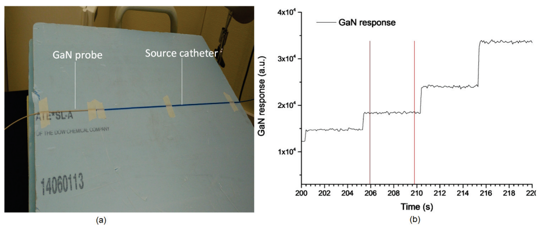
FIGURE 4.4 – a) Configuration de la caractérisation de la dépendance du débit de dose ; b) Exemple du signal acquis au cours de la mesure.
