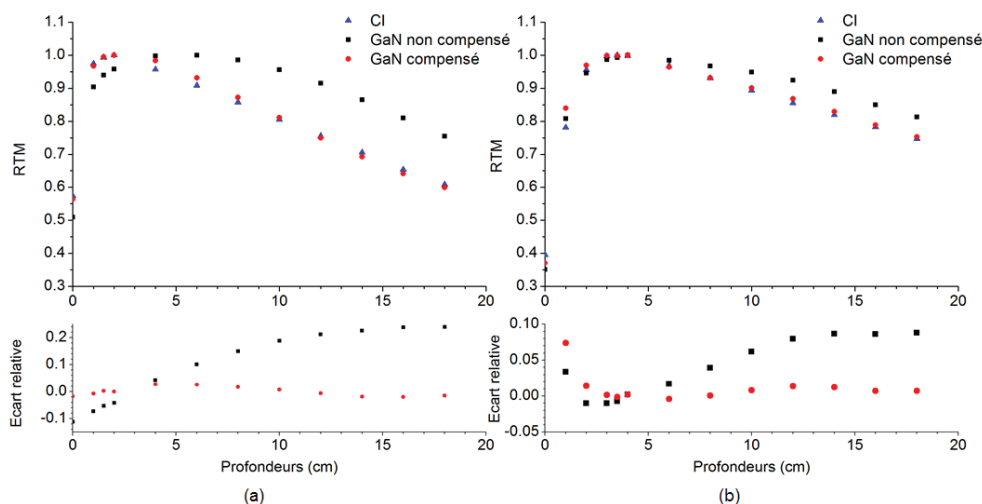
FIGURE 2.7 – Mesures de RTM avec le transducteur GaN avant et après compensation pour des faisceaux a) de 6 MV et b) de 18 MV dans un champ carré de 17 \times 17 \text{ cm}^2 . Les écarts relatifs sont donnés par rapport aux mesures de référence obtenues avec la chambre d’ionisation.
