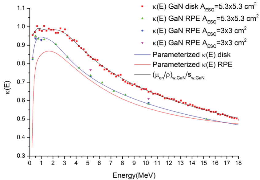
FIGURE 2.16 – facteur \kappa(E) en fonction de l'énergie des photons incidents pour deux tailles de cavité GaN, un cylindre ( h = 0,1 \text{ cm} r = 0,125 \text{ cm} ) et un lingot parallélépipédique ( 0,03 \times 0,03 \times 0,1 \text{ cm}^3 ) et pour différentes tailles du champ (pour les champs circulaires, la légende fait apparaître les champs carrés équivalents).
