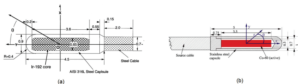
FIGURE 4.13 – Vue en coupe d'une source HDR a) ^{192}\text{Ir} Micro Selectron [205]; b) ^{60}\text{Co} 0.A86 [207].
