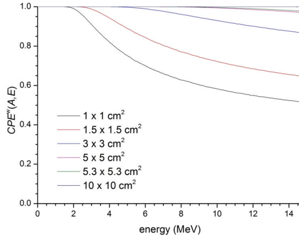
FIGURE 2.14 – CPE^{\text{w}}(A, E) calculé pour des différentes tailles du champ, avec un faisceau de photon mono-énergétique [156].
