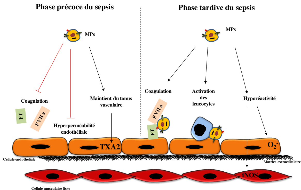
Figure 14: Rôle des MPs dans le sepsis. D'après Reid et al., 2012. FT, facteur tissulaire; FVIIa, facteur tissulaire VIIa; TXA2, thromboxane A2; O_2^- , anion superoxyde; iNOS, NO synthase inductible.
