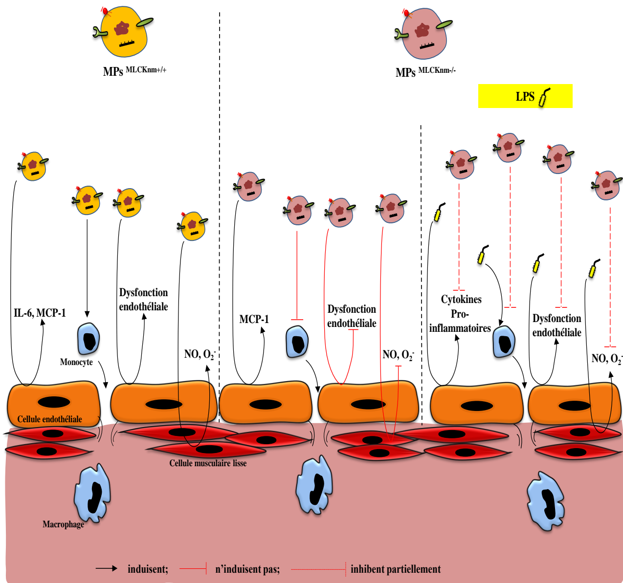
Figure 16: Schéma récapitulatif des principaux résultats de la deuxième partie de l'étude. MPs^{MLCKnm+/+} : MPs circulantes issues des souris sauvages; MPs^{MLCKnm-/-} : MPs circulantes issues des souris KO MLCKnm. IL-6: interleukine 6; MCP-1: protéine chimiokine des monocytes 1; NO: monoxyde d'azote; O_2^- : anion superoxyde. Les MPs^{MLCKnm+/+} induisent la production par les cellules endothéliales du IL-6 et MCP-1. Les MPs^{MLCKnm-/-} induisent la production que du MCP-1. Les MPs^{MLCKnm+/+} et non pas les MPs^{MLCKnm-/-} , induisent l'infiltration des macrophages, une dysfonction endothéliale ainsi qu'une production de NO et O_2^- . En présence du LPS, les MPs^{MLCKnm-/-} protègent partiellement contre les effets du LPS.
