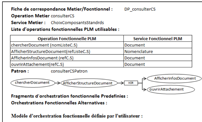
Figure 65 : Fiche de correspondance métier/fonctionnel de l'opération ConsulterCS
