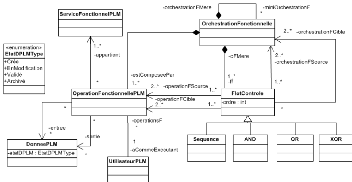
Figure 37 : Méta-modèle d'orchestration fonctionnelle
