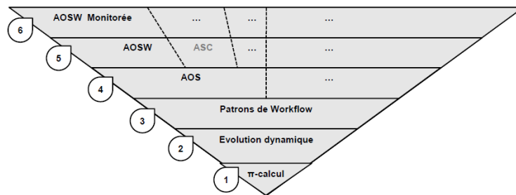
Figure 7 : Les différentes couches du langage PXL [Verjus 11]
