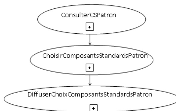
Figure 68 : Orchestration fonctionnelle ChoixdeComposantsStandard_OF
