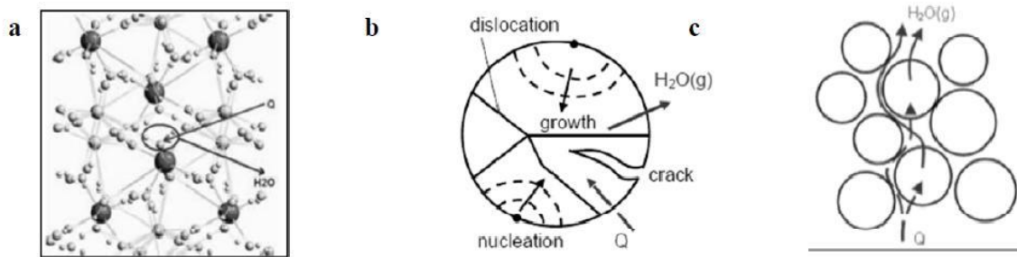
Figure 24 : Différentes échelles de déroulement des phénomènes, a) l'échelle du cristal, b) l'échelle du grain, c) l'échelle du lit réactif.
