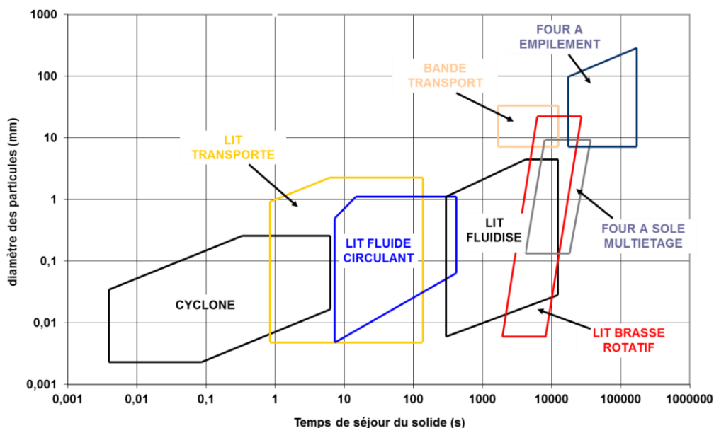
Figure 19 : Plages d'utilisation des différents types de réacteurs solide-gaz [Villermux 1979], [Pardo 2013].
