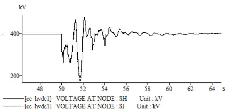
(b) Réponses en tension côtés SH et SI (HVDC 2)
