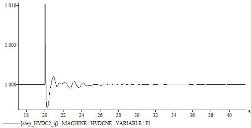
(a) Réponse de la puissance active côté NE (HVDC 1)
