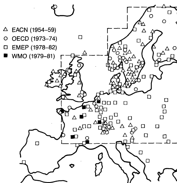
Figure 23 : Principaux réseaux européens de surveillance de la pollution atmosphérique de fond, et en particulier des concentrations de SO 2 dans les eaux de pluies, entre 1954 et le début des années 1980 [Popovics et al. , 1987, “Fig. 1. Networks of different monitoring programs of background pollution”, p. 48]
