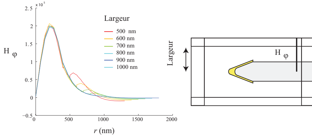
FIGURE D.2 – Profil du champ dans la fibre pour différentes largeurs de fenêtre. La couche PML a pour épaisseur 400 nm. Le rayon de la fibre nue est de R_0 = 400 nm.
