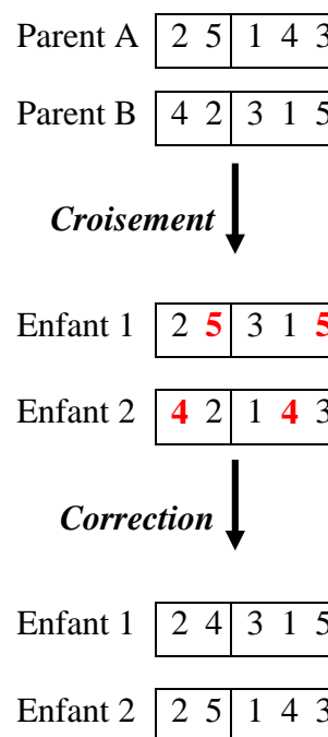
Figure 7.3 : Exemple d'une opération de croisement
