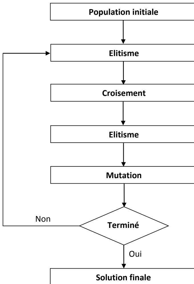
Figure 7.5 : Fonctionnement de l'algorithme génétique
