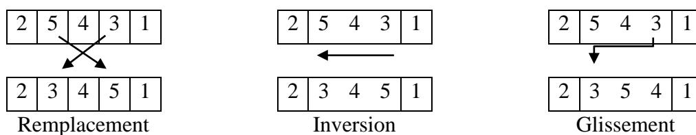
Figure 7.4 : Trois opérations de mutation
