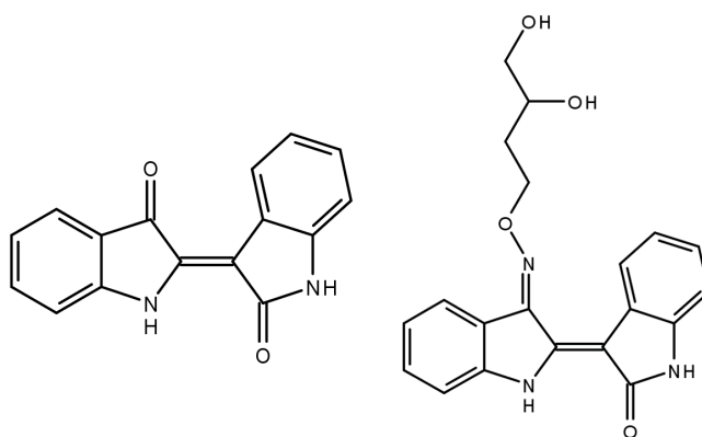
Figure 12 : Structure chimique de l'indirubine (gauche) et du composé E804 (droite).
