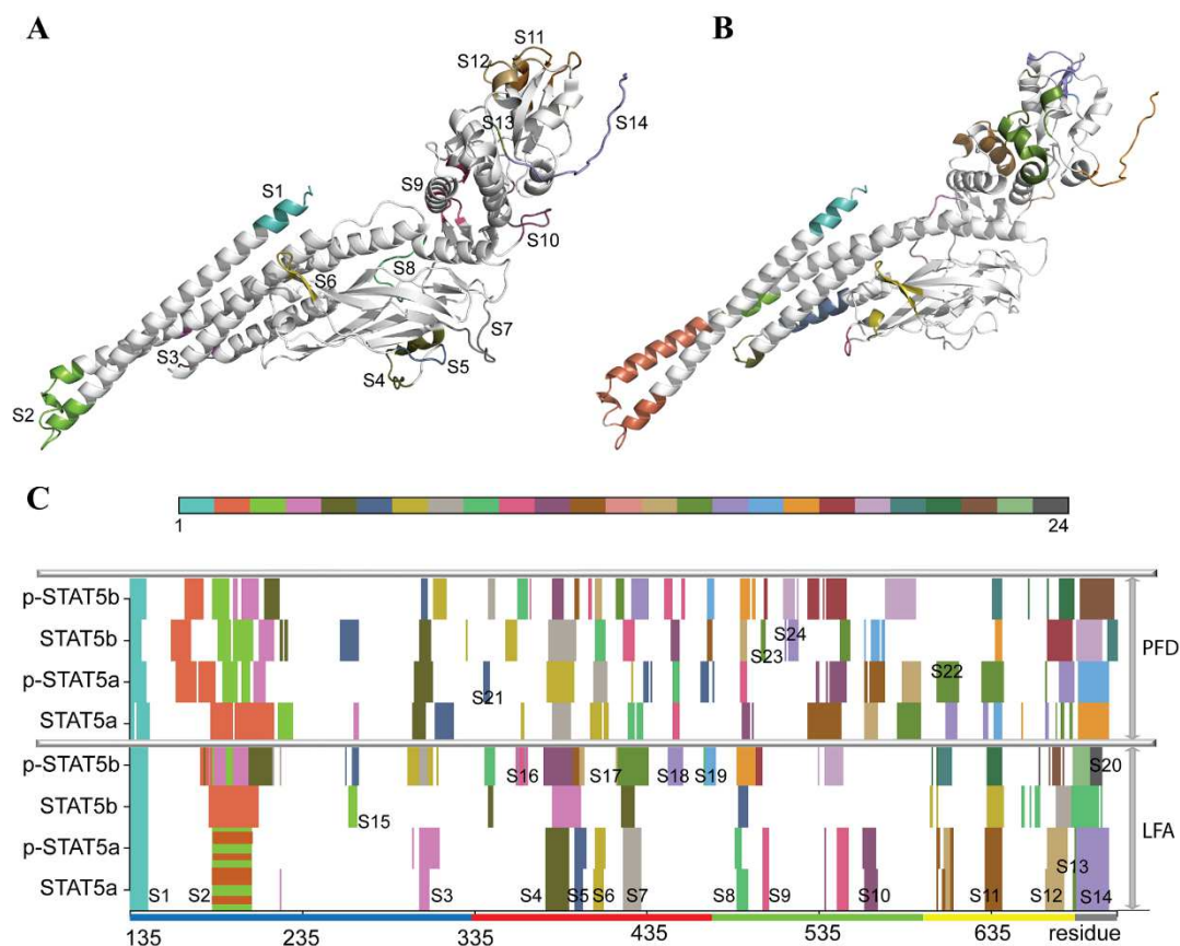
Figure 44: Position des Segments Dynamiques Indépendants identifiés dans les protéines STAT5s. (haut) Représentation tridimensionnelle de la position des IDSs identifiés par les algorithmes LFA (A) et PFD (B). Les IDSs sont indiqués par la S_i , où i = 1 \dots 24 . (bas, C) Représentation graphique de la position des IDSs pour chaque système, par les deux méthodes. Chaque couleur représente un IDS ; les IDSs superposables sont hachurés.
