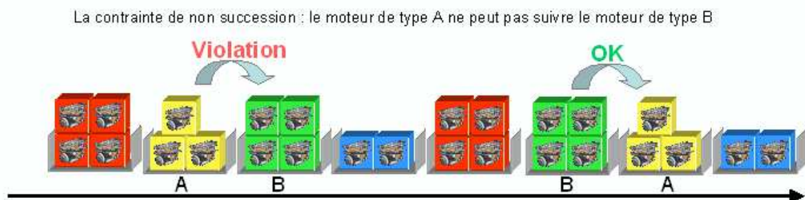
Figure II- 10:La contrainte de non succession
