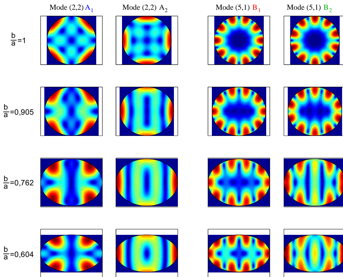
FIGURE 2.6 – Déformées modales.
