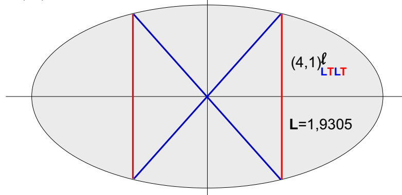
FIGURE 2.11 – Orbites périodiques n = 4 , m = 1 avec mouvement de libration pour un disque elliptique b/a = 0,5227 a) de pression pure ou cisaillement pur , b) avec conversion de mode TLTL, c) avec conversion de mode LTLT.
