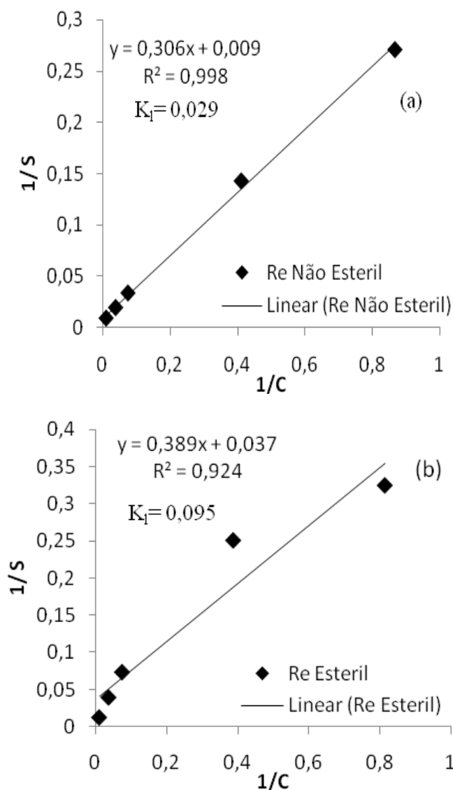
Figura 11 - Isotherma de sorção do sulfametoxazol (SMX) no solo Recife não estéril (c) e estéril (d).
