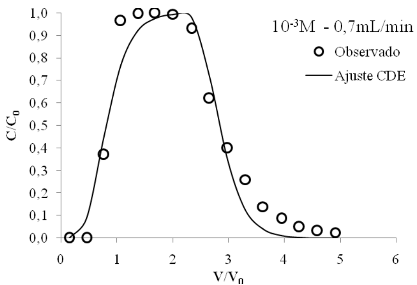
Figura 29 - Curvas médias de eluição do SMX ajustadas pelo modelo CDE, em colunas de solo Macon na concentração de 10 -3 M nas vazões de 0,2; 0,45 e 0,7 mL/min.
