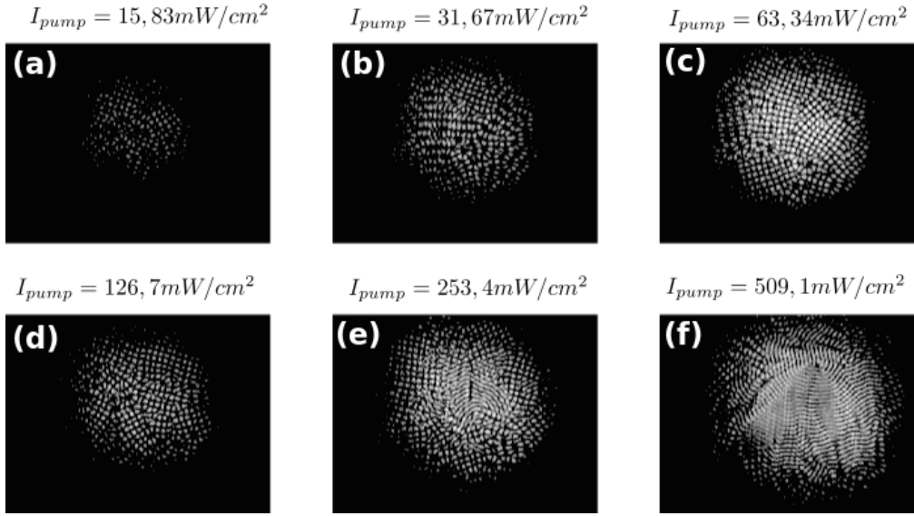
FIGURE 2.30 – Evolution des instabilités (dans le canal \perp ) en fonction de l'intensité de la pompe. Le désaccord du faisceau est \delta = -7,76 \Gamma et t_{pump} = 200 \mu s .
