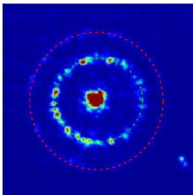
FIGURE 2.12 – Exemple d'image au champ lointain de la section transversale de la pompe après passage à travers le centre du nuage. Le petit cercle (en pointillés vert) représente le mode fondamental , et le plus grand (en pointillés rouges) le 1 er mode supérieur .
