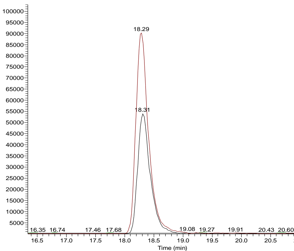
Figure V-3-b-2 : Chromatogrammes de détection par spectrométrie de masse du 5'-désoxyadénosyle après éluion sur colonne HPLC C18. En rouge : masse détectée de 253 g.mol -1 (AdoD), en noir : masse détectée de 252 g.mol -1 (AdoH). Les unités en abscisse correspondent au temps d'éluion sur la colonne HPLC.
