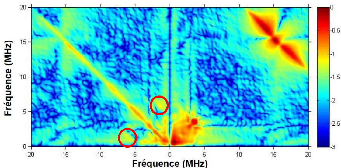
Figure I-4-d-2 : Spectre RPE-HYSCORE du mutant RimO-RS. L'échantillon analysé contient 80 \mu\text{L} à 425 \mu\text{M} d'holoprotéine réduite. La réduction est réalisée par incubation avec 10 équivalents de dithionite pendant 30 minutes. Les conditions d'enregistrements de ce spectre sont : Température = 8 K / Champ magnétique = 3580 G / Fréquence = 9,71 GHz / Transformée de Fourier 2D.
