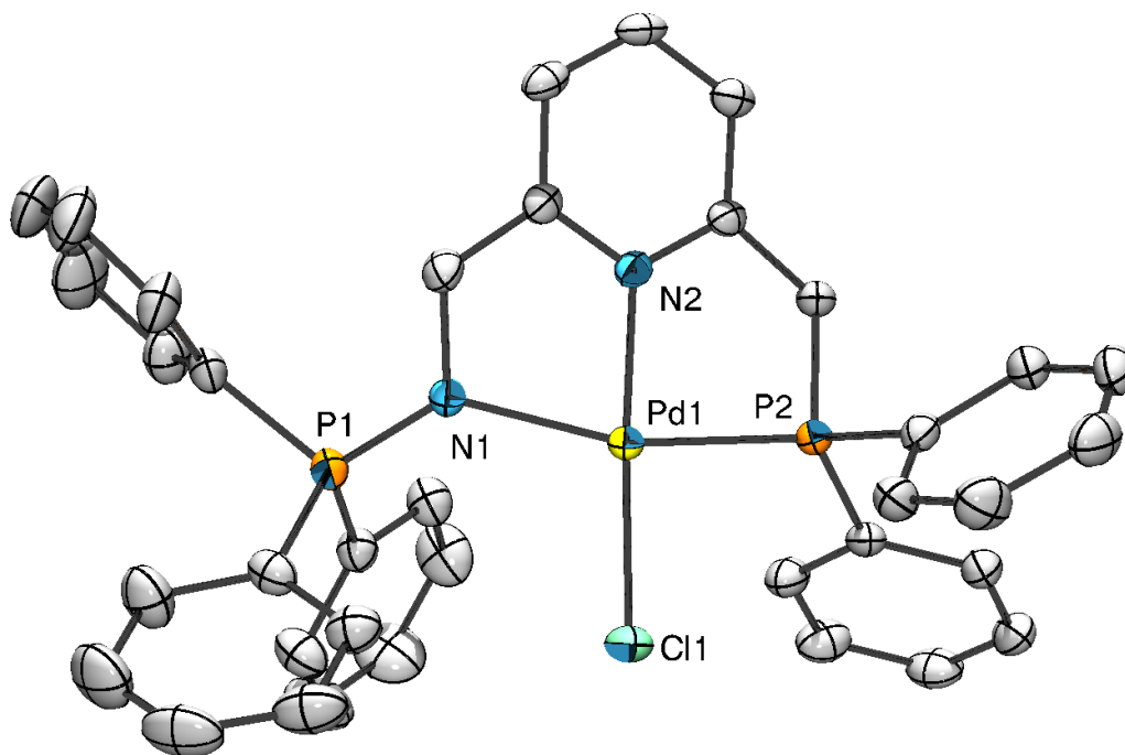
Figure 64 - ORTEP de [L 1 PdCl]Cl – Les atomes d'hydrogènes, une molécule de benzonitrile et le contre-ion chlorure ont été omis pour plus de clarté. Longueurs de liaisons (Å) et angles (°) sélectionnés : N1-P1 1,603(2), N1-Pd1 2,110(2), P2-Pd1 2,2112(7), N2-Pd1 1,998(2), Cl1-Pd1 2,2953(7) ; N1-Pd1-P2 164,23(6), N2-Pd1-Cl1 175,95(6), N1-Pd1-N2 80,2(1), P2-Pd1-N2 84,04(6), N1-Pd1-Cl1 99,9(2), P2-Pd1-Cl1 93,19(3).
