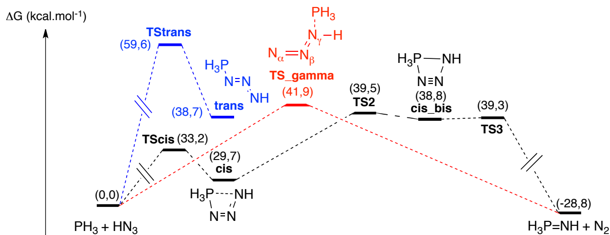
Schéma 14 - Profil énergétique de la réaction entre PH 3 et HN 3
