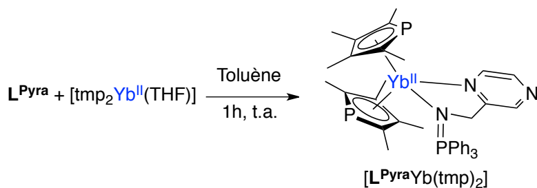
Schéma 155 - Synthèse de [L^{Pyra}Yb(tmp)_2]
