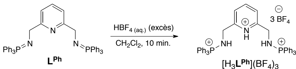
Schéma 86 - Protonation de L^{Ph}
