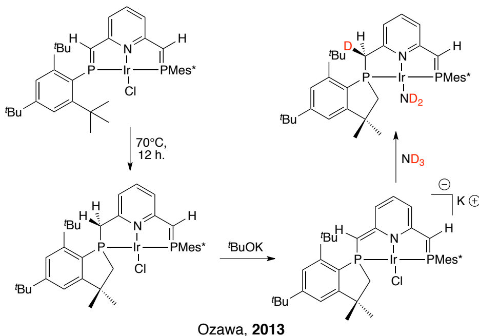
Schéma 63 - Isomérisation et coopération métal-ligand d'un pinceur phosphaalcène
