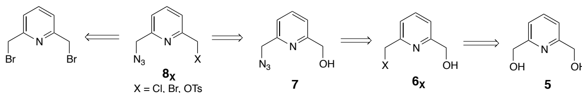
Schéma 171 – Rétrosynthèses possibles pour l'intermédiaire clé \mathbf{8}_X
