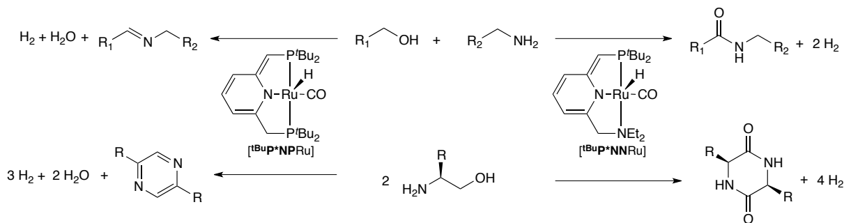
Schéma 57 - Divergence de réactivité en fonction de l'hémilabilité du ligand pincer
