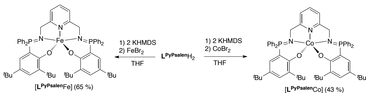
Schéma 226 - Synthèse de complexes de cobalt et de fer du ligand L^{PyPsalen}
