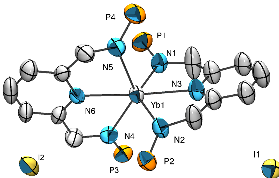
Figure 39 - ORTEP de [\text{L}^{\text{Et}}\text{)}_2\text{Yb]}_2\text{I}_2 – Les substituants éthyles des atomes de phosphore et les atomes d'hydrogènes ont été omis pour plus de clarté. Longueurs de liaisons (Å) et angles ( ^\circ ) sélectionnés : N1-P1 1,59(1), N2-P2 1,61(1), N4-P3 1,61(1), N5-P4 1,58(1), N1-Yb1 2,52(1), N2-Yb1 2,51(1), N3-Yb1 2,49(1), N4-Yb1 2,47(1), N5-Yb1 2,52(1), N6-Yb1 2,49(1) ; N4-Yb1-N5 133.3(3), N4-Yb1-N6 66.2(3), N5-Yb1-N6 67.3(3), N4-Yb1-N3 105.9(3), N5-Yb1-N3 120.6(3), N6-Yb1-N3 167.6(3), N4-Yb1-N2 102.9(3), N5-Yb1-N2 99.3(3), N6-Yb1-N2 123.8(3), N3-Yb1-N2 66.3(3), N4-Yb1-N1 96.7(4), N5-Yb1-N1 96.9(3), N6-Yb1-N1 102.8(3), N3-Yb1-N1 67.8(3).
