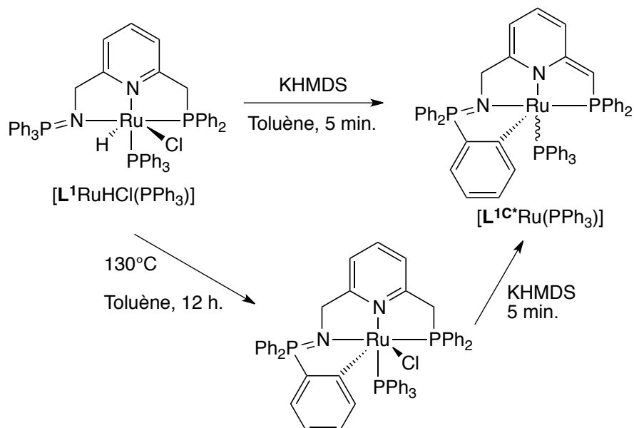
Schéma 208 - Accélération de la cycloméallation par déaromatation
