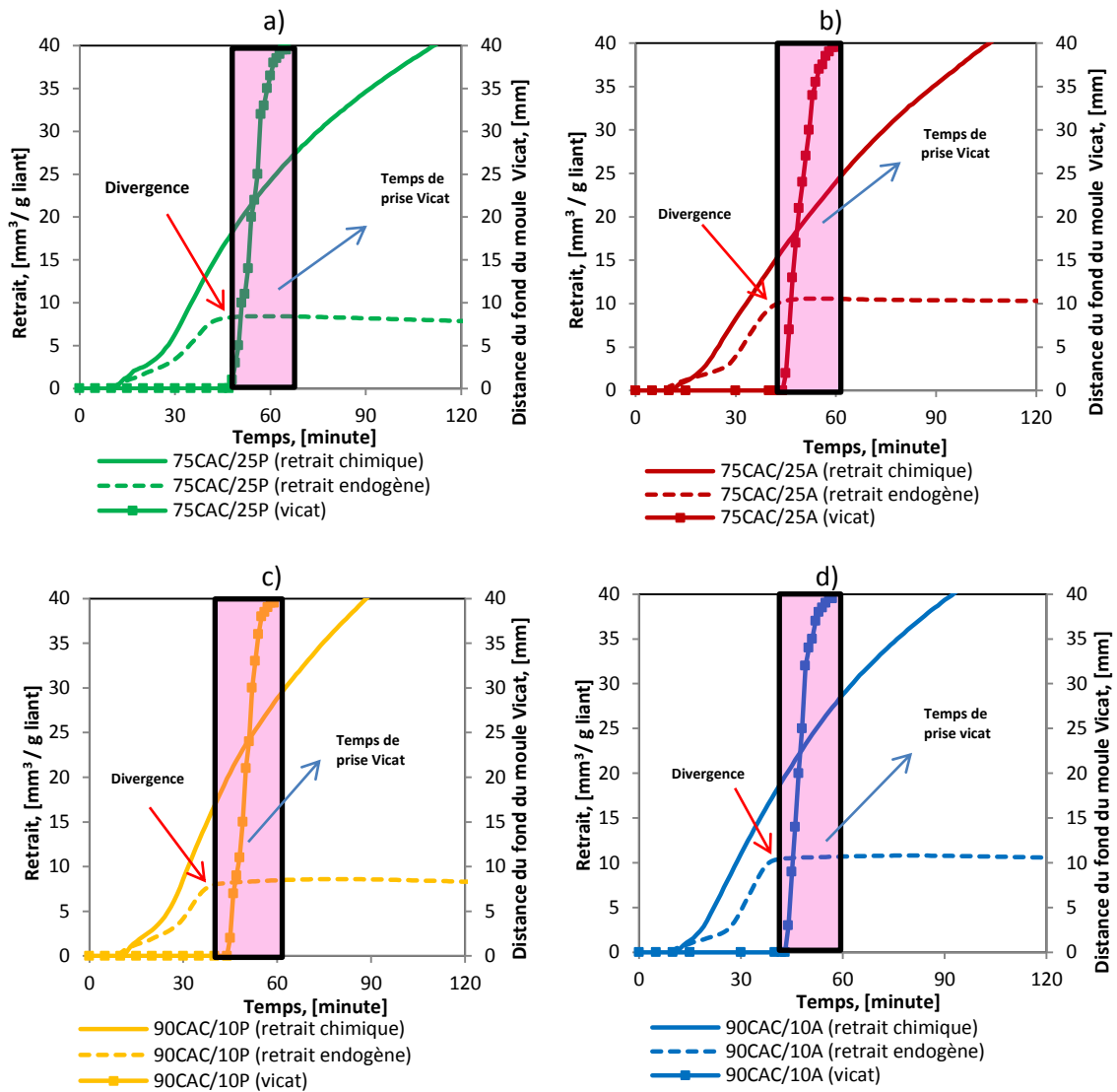
Figure 3.12 Comparaison entre cinétique de retrait chimique, retrait endogène et temps de prise a – Composition 75CAC/25P b - Composition 75CAC/25A c - Composition 90CAC/10P d - Composition 90CAC/10A
