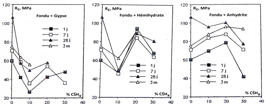
Figure 1.15. Influence de la nature du sulfate de calcium et de son dosage sur les résistances en compression pour les mélanges Fondu + sulfate de calcium (Bayoux et al. 1990).
