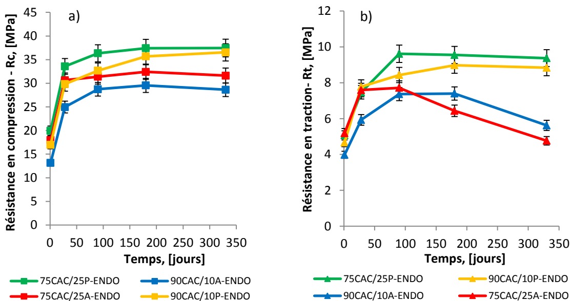
Figure 4.14 Evolution de la résistance des mortiers en condition endogène a) Résistance en compression b) Résistance en traction
