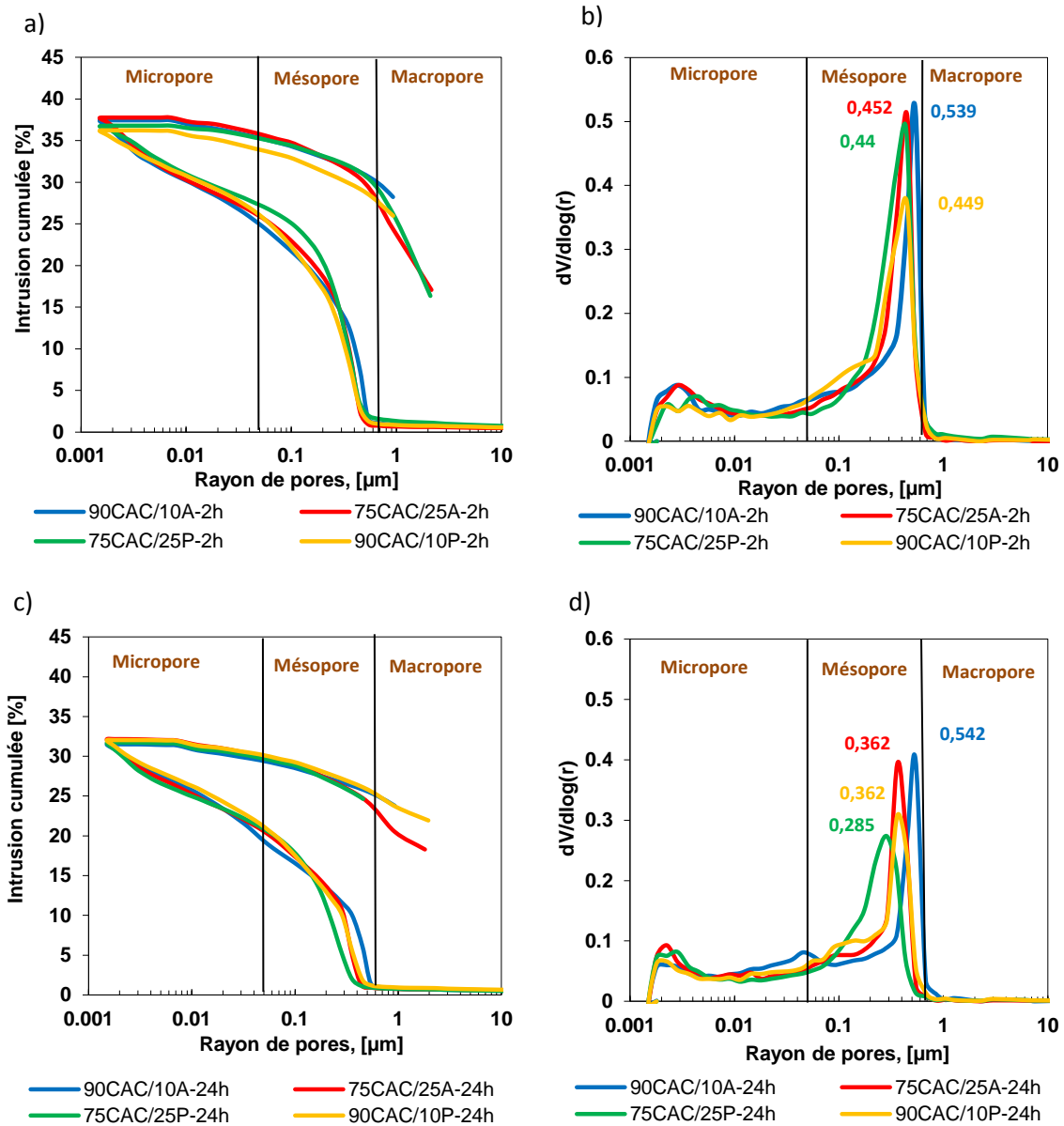
Figure 3.32 : Distribution cumulée des pores à 2h et à 24h.
