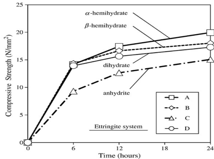
Figure 1.14 Evolution de la résistance des mortiers ettringitiques (64,5% CAC - 22,6% \overline{CSH}_x - 12,9% CEM) avec différents natures du sulfate de calcium (Kouji Onishi et al. 2010).
