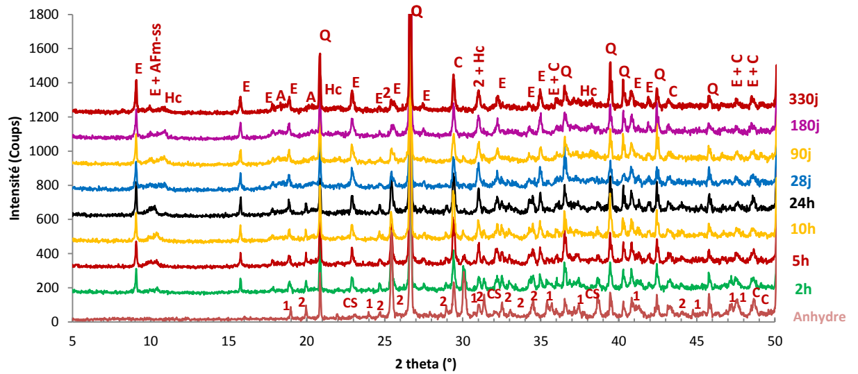
Figure A.2. Diffractogrammes de la composition 75CAC/25A jusqu'à 330j.
