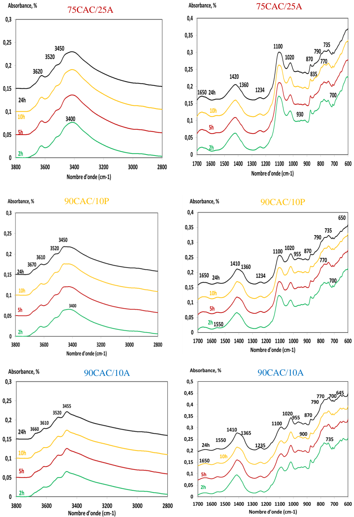
Figure 3.29 Evolution des signaux infrarouge de 2h à 24h
