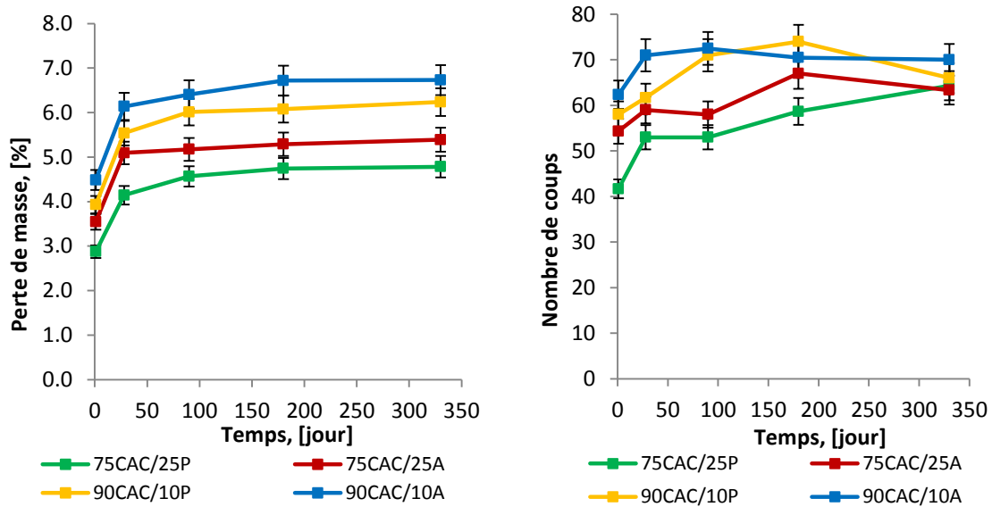
Figure 4.5 Evolution de l'AH 3 des 4 compositions a) Evolution de l'AH 3 par DTA-TG au pic de 270 à 350 o C b) Evolution de l'AH 3 par DRX au pic 2θ= 18.4, 20.3 o
