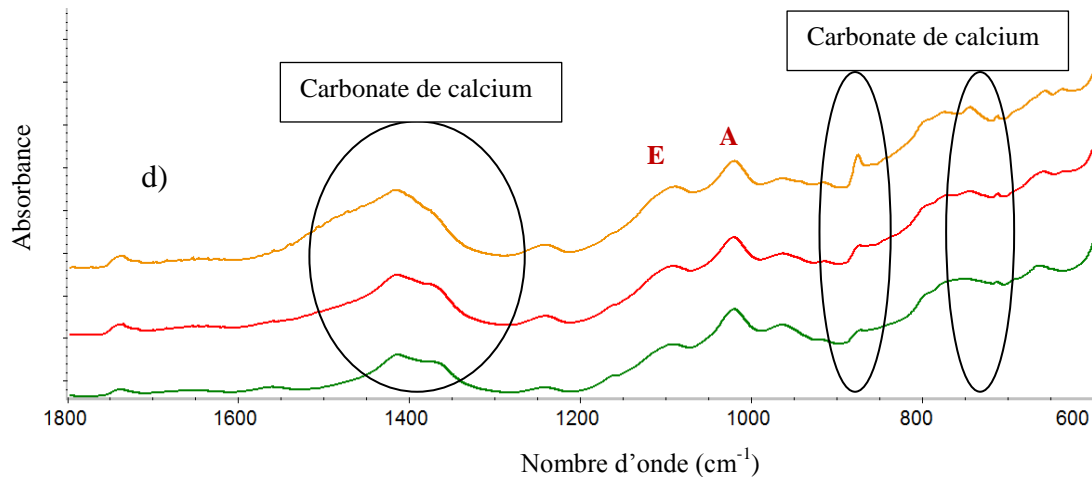
Figure 4.22 Comparaison des résultats IR de l'échantillon en endogène avec l'échantillon au séchage
