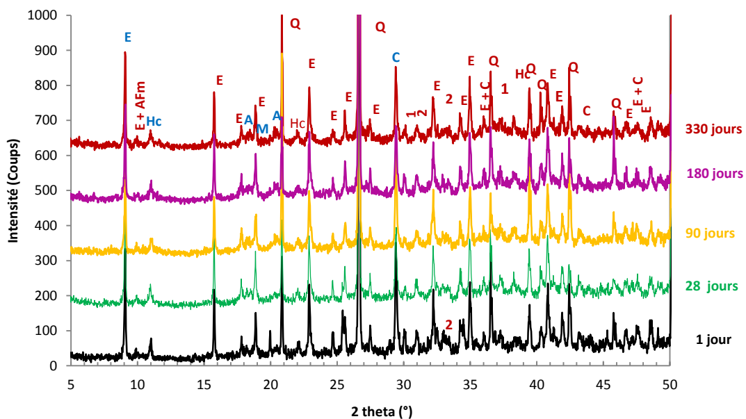
Figure 4.1: Diffractogrammes de la composition 75CAC/25P de 1j à 330j.
