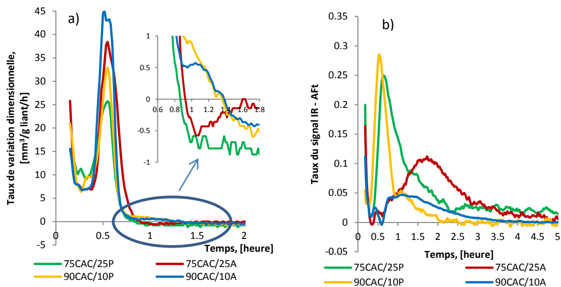
Figure 3.36 Vitesse de la déformation endogène volumique en fonction du temps a) Courbe de l'évolution de déformation endogène volumique b) Vitesse du signal IR de l'ettringite en fonction du temps
