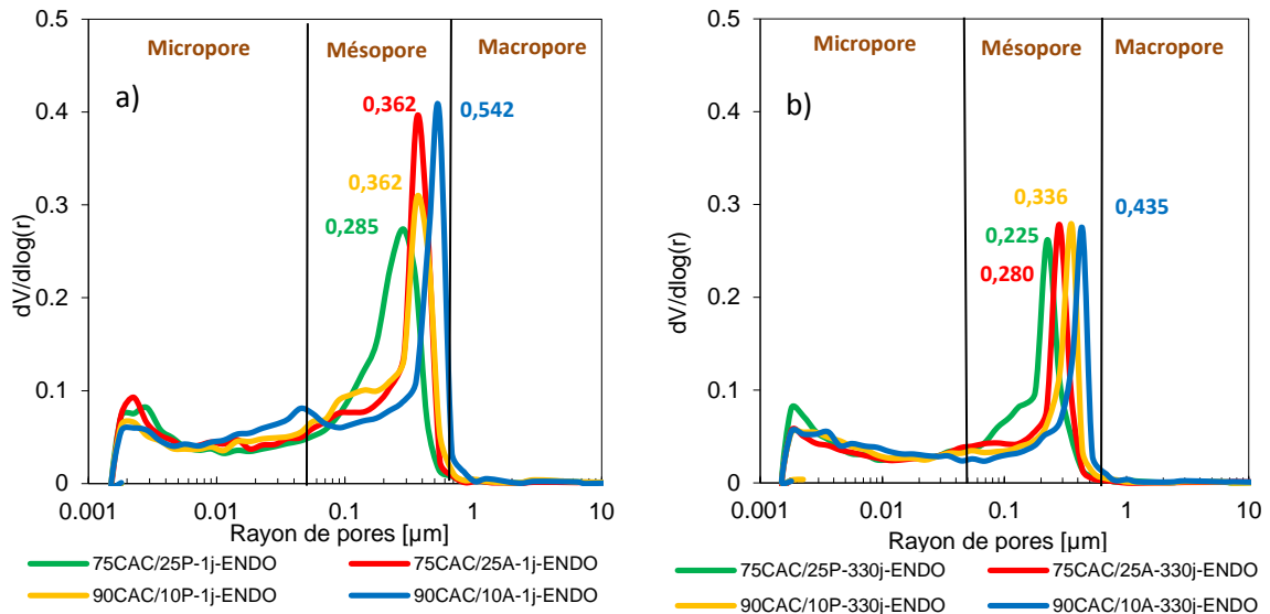
Figure 4.12 Comparaison de la distribution poreuse des 4 compositions a) 1 jour et b) 330 jours
