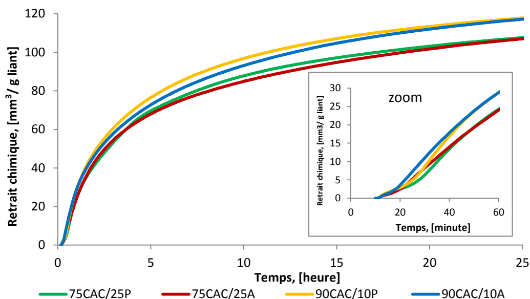
Figure 3.3: Influence de la nature et du dosage du sulfate de calcium sur le retrait chimique jusqu'à 24h (début des mesures à 10 minutes).
