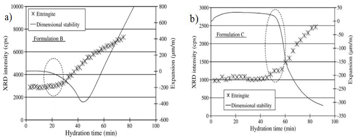
Figure 1.12 Evolution de l'ettringite et du gonflement à très jeune âge des compositions ettringitiques (Kouji Onishi et al. 2010)
