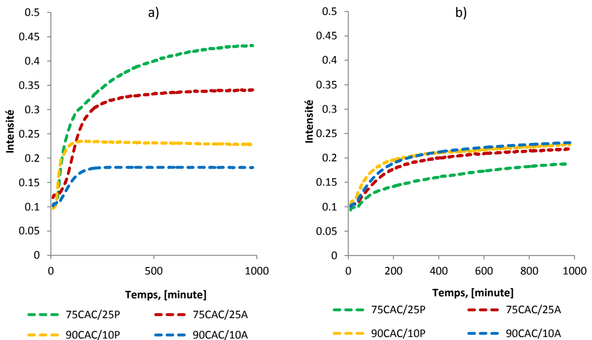
Figure 3.17 Evolution de l'intensité du signal IR de l'ettringite et de l' AH_3 a) Evolution de l'ettringite à la bande 1100\text{cm}^{-1} b) Evolution de l' AH_3 à la bande 1020\text{cm}^{-1}
