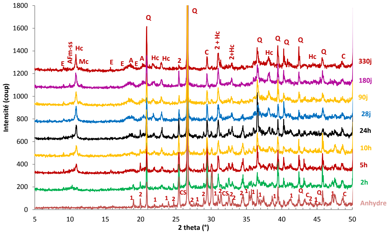
Figure A.4. Diffractogrammes de la composition 90CAC/10A jusqu'à 330j.
