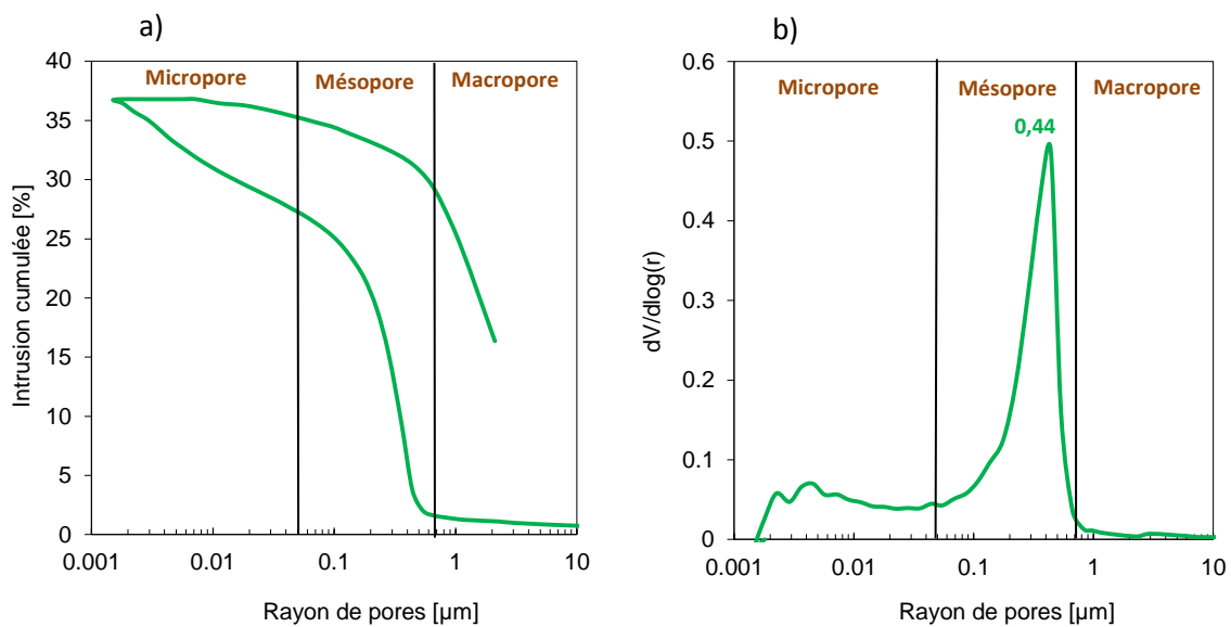
Figure 2.9 Distribution de la porosité d'un mortier contenant 75CAC/25P a) Distribution poreuse cumulée b) Distribution poreuse
