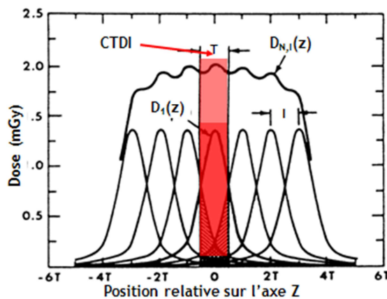
Profil de dose pour plusieurs coupes
