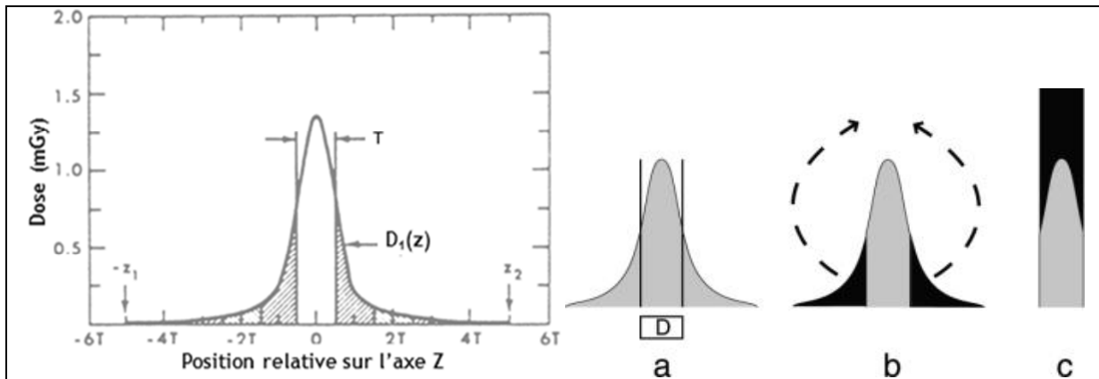
Profil de dose pour une coupe
