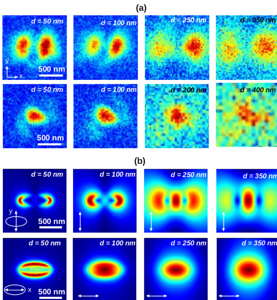
Figure 5.10: Cartes d'intensité en transmission mesurées (a) et calculées (b) avec deux polarisations orientées suivant l'axe majeur et l'axe mineur de l'ellipse pour différentes distances d .
