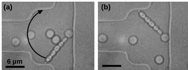
Figure 1.8: Valve constituée de microparticules assemblées par photopolymérisation. La valve est contrôlée par la pince optique et dirige les microparticules vers le haut (a) ou vers le bas (b). [17]
