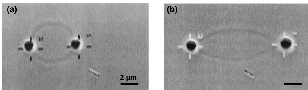
Figure 1.9: Images d'un globule rouge avant (a) et après étirement (b) par la séparation de deux billes diélectriques d'1 µm de diamètre piégées optiquement. [21]
