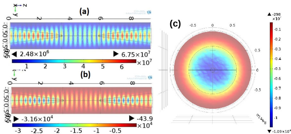
Figure 4.22: Simulation de deux pointes placées en face à face et séparées de 2,5 \mu\text{m} . Carte du champ électrique (a) et énergie potentielle dans la direction axiale (b) et transverse (c) pour une particule de YAG 300.
