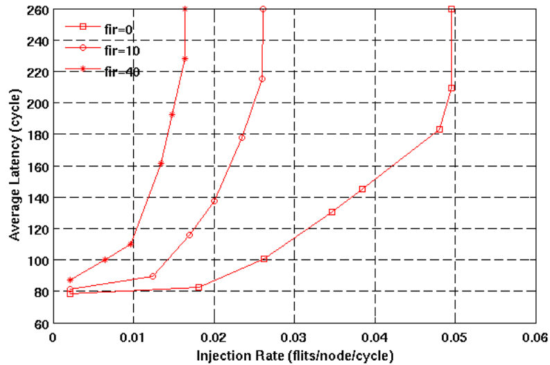
Fig. A.2.c. Latence moyenne de CAFTA avec différents ratio d'injection de faute (faute de routeurs) sous le trafic « Bit complement» pour un NoC 16x16 en tore 2D
