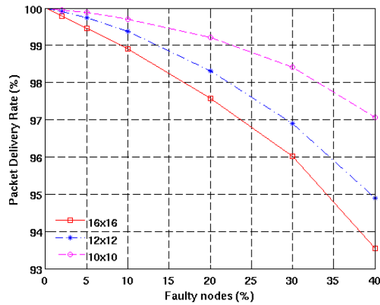
Figure 4.10 Taux de paquets délivrés avec succès pour différentes tailles de réseau et différents taux d'injection de fautes (faute de nœud) sous le trafic (a) « Uniform Random », (b) « Transpose », (c) « Bit complement », pour un NoC 2D Mesh
