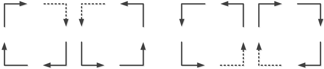
Figure 1.2 Routage South-Last (à gauche) / North-Last (à droite)
