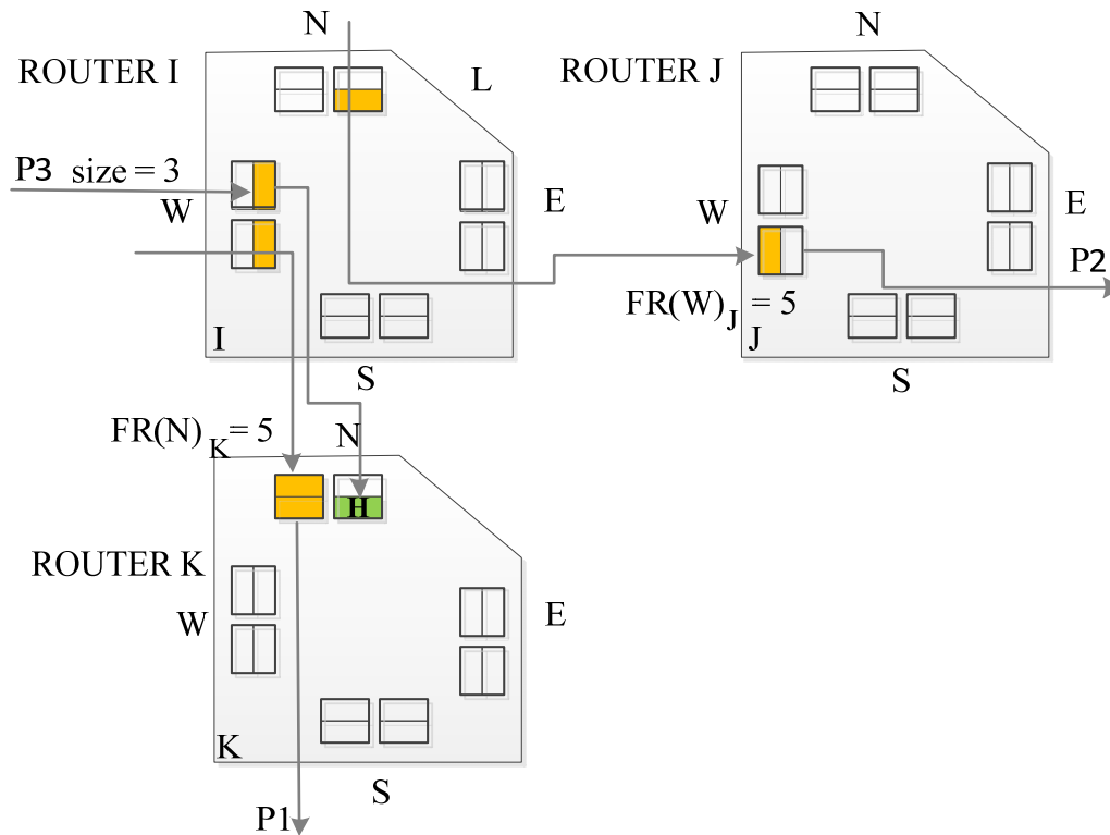
(c) Mise à jour de la valeur de FR dans le cas du choix basé sur « Flit Remain ».
