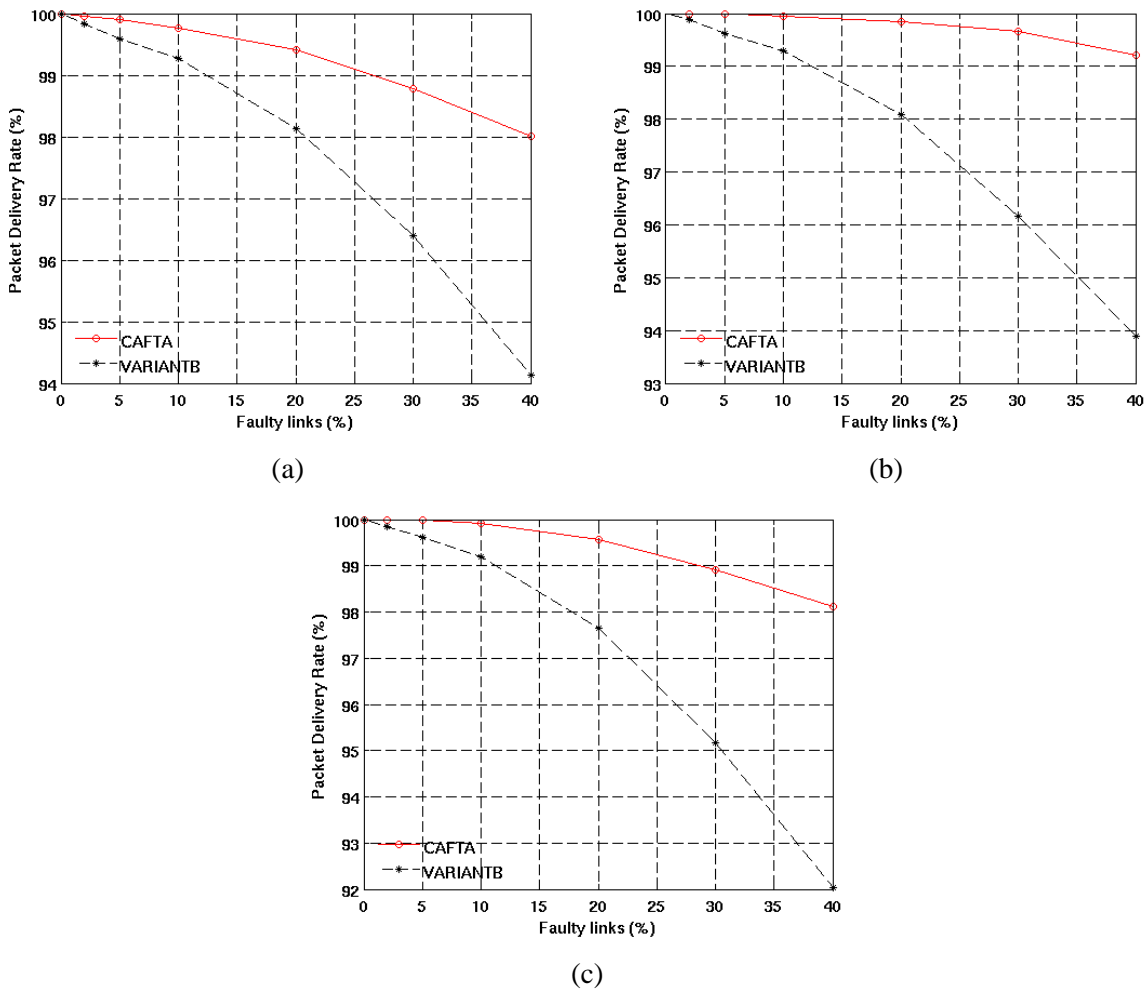
Figure 4.6 Taux de réussite avec différents ratios d'injection de faute (faute de liens) sous le trafic : (a) « Uniform Random », (b) « Transpose », (c) « Bit complement », pour un NoC en maille 16x16
