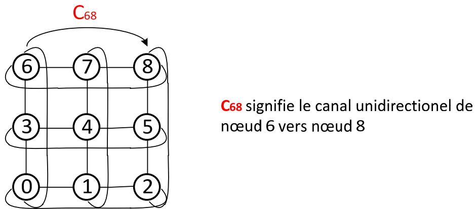
Figure 3.7 Un exemple de 3x3 Tore 2D
