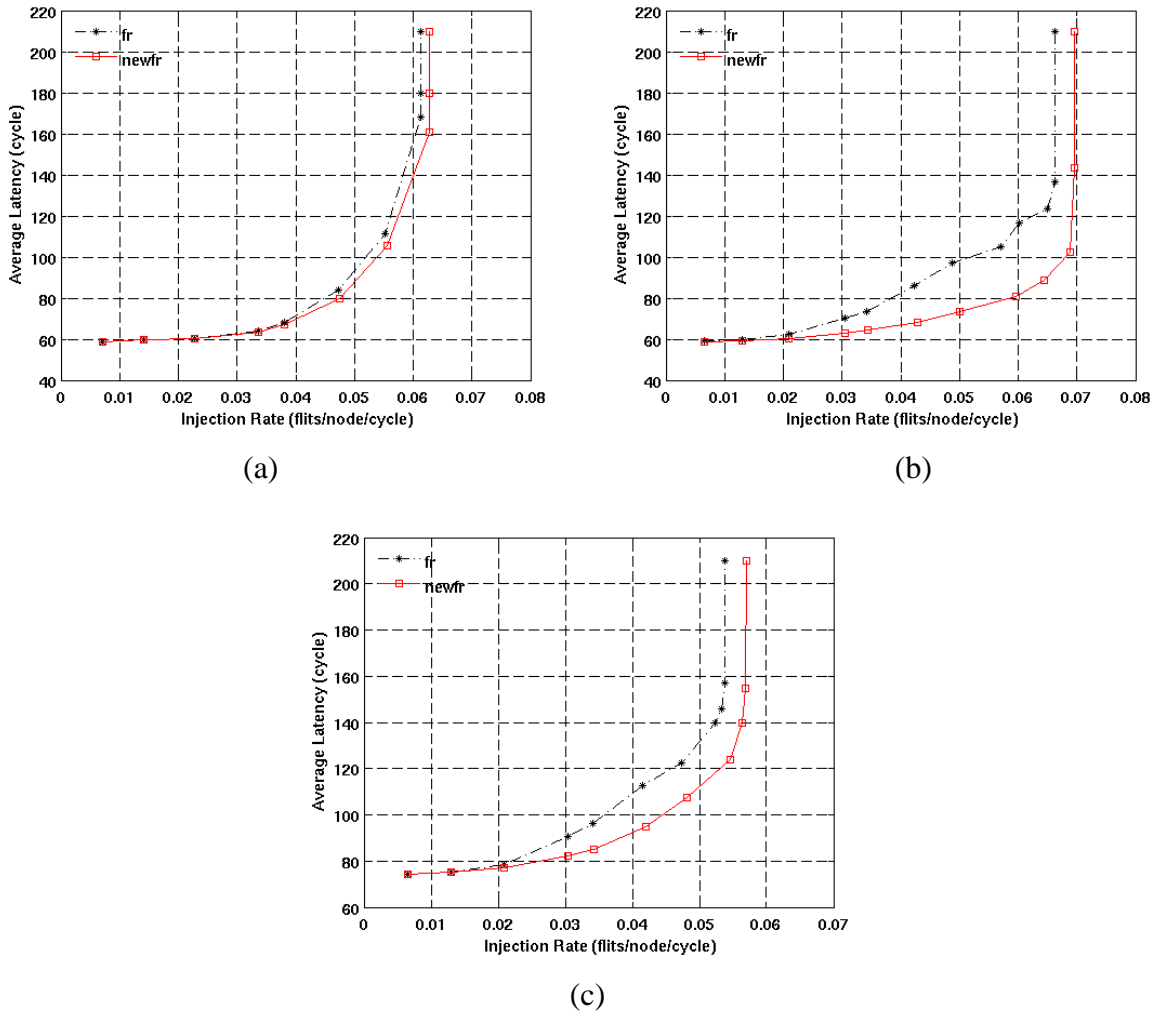
Figure 4.12 Latence moyenne avec différentes métriques de congestion sous le trafic (a) « Uniform Random », (b) « Transpose» et (c) pour un NoC 16x16 sans injection de fautes
