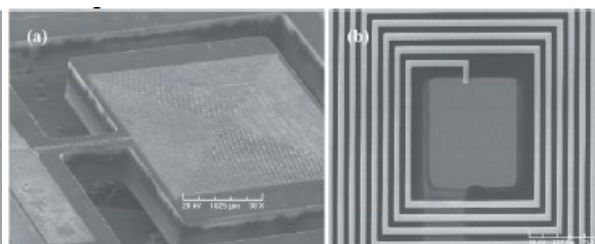
Figure 1-8 Deux architectures de bobines [KKTB07].
