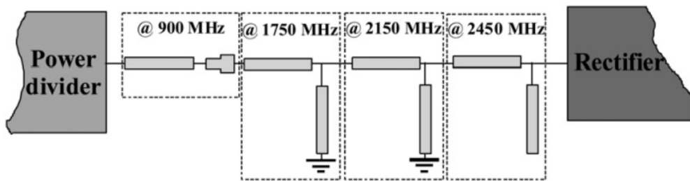
Figure 2-5 Réseau d'adaptation conçu par [MCPR13].
