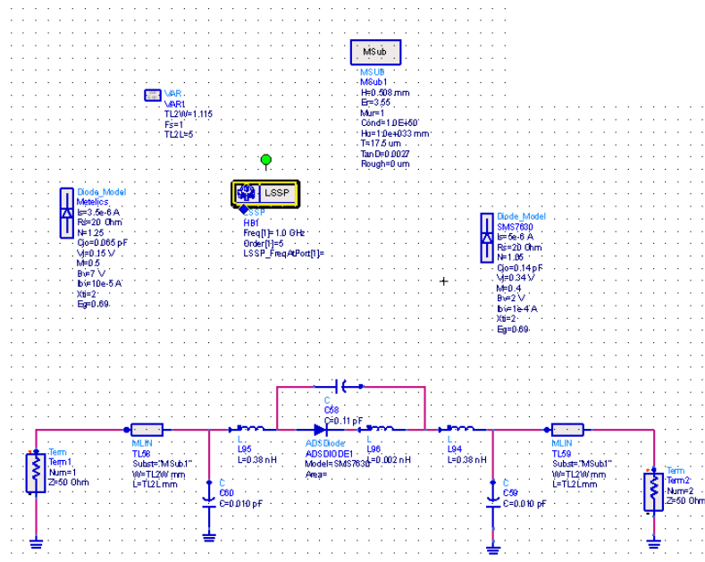
Figure 1-0-6 Simulation pour calculer les paramètres S de la diode Schottky
