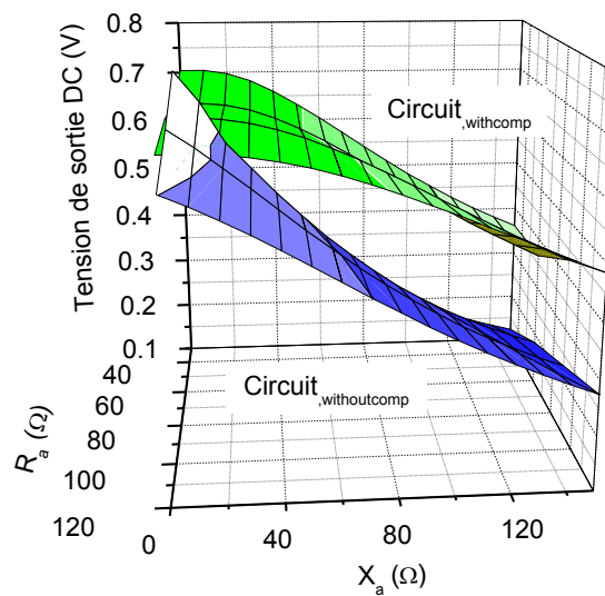
Figure 4-24 Tension de sortie DC simulée en fonction de R_a et X_a pour F_{req} = 950 MHz, R_L = 11 k \Omega .
