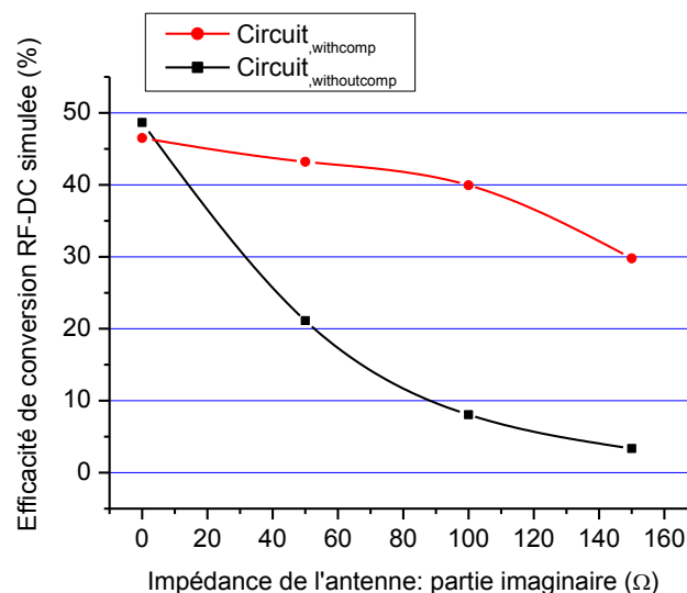
Figure 4-25 Efficacité de conversion de la rectenna simulée en fonction de la partie imaginaire de l'impédance de l'antenne pour F_{req} = 950 MHz, R_L = 11 k \Omega .
