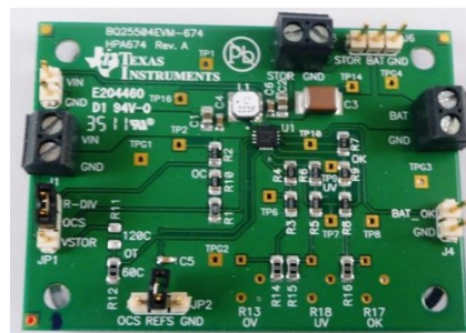
Figure 3-45 Photo de la carte d'évaluation du convertisseur BQ25504.
