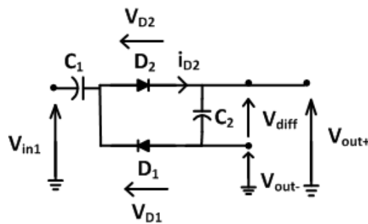
Figure 3-31 Architecture du redresseur proposé.
