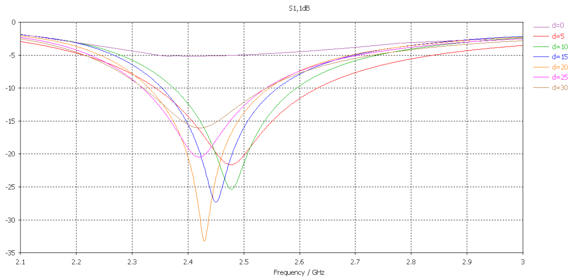
Figure 4-8 Coefficient de réflexion de l'antenne en fonction de la fréquence pour plusieurs distances d [0 ; 30] mm.
