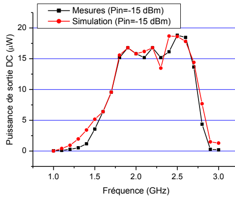
Figure 3-15 Puissance de sortie simulée et mesurée pour une puissance incidente de -15 dBm.
