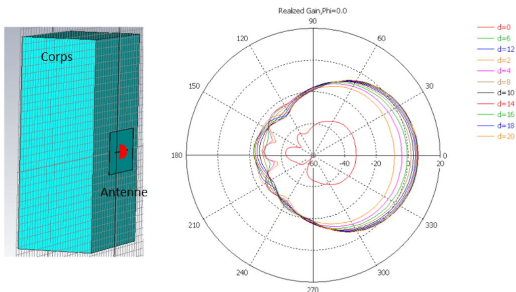
Figure 4-5 Gain réalisé de l'antenne en fonction de la distance entre l'antenne et le corps.
