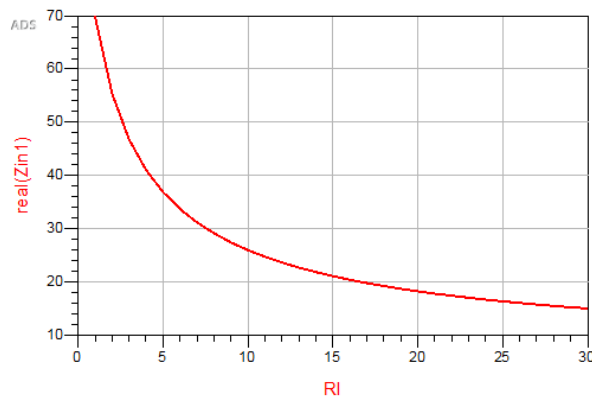
Figure 2-34 Impédance (partie réelle) vue de l'entrée du redresseur en fonction de la charge R_L en kΩ.
