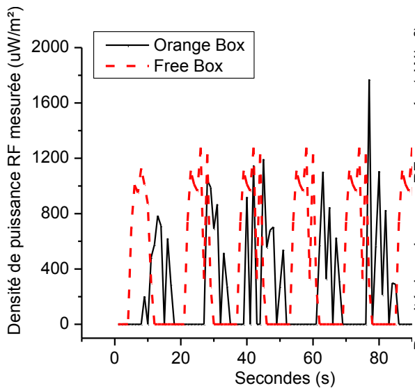
Figure 2-13 Densité de puissance RF mesurée pour deux routeurs Wi-Fi.
