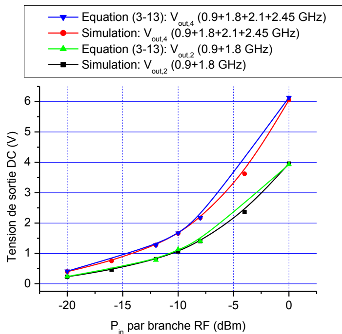
Figure 3-34 Tension de sortie simulée en fonction de la puissance incidente pour chaque fréquence comparée à la tension calculée à partir du modèle mathématique (3-13) pour R_L=11\text{ k}\Omega .
