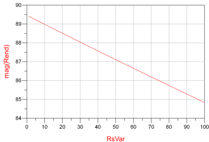
Figure 1-0-3 Efficacité de conversion en fonction de R_s .
