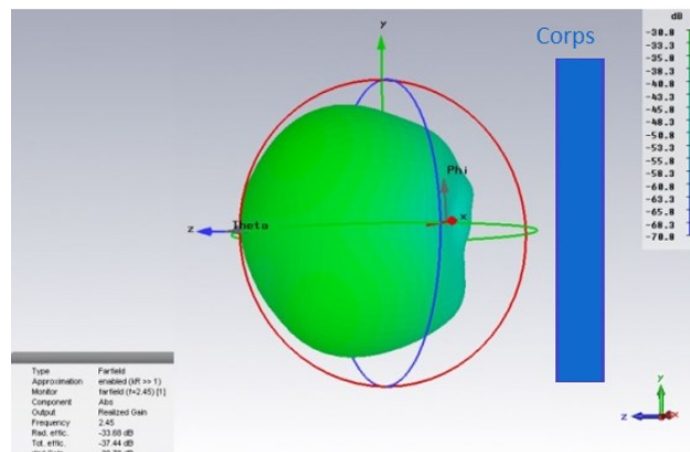
Figure 4-4 Gain réalisé de l'antenne lorsque l'antenne est collée sur le corps ( d= 0 ).
