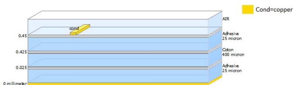
Figure 0-1 Composition de la structure modélisée sous ADS.
