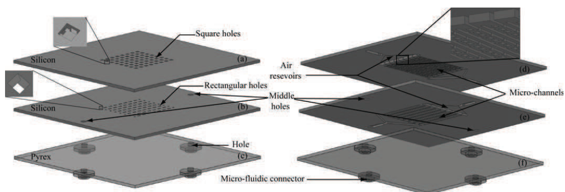
FIGURE 5.6 – Le prototype de micro-convoyeur développé par Zeggari et al. [75] est constitué de trois couches.
