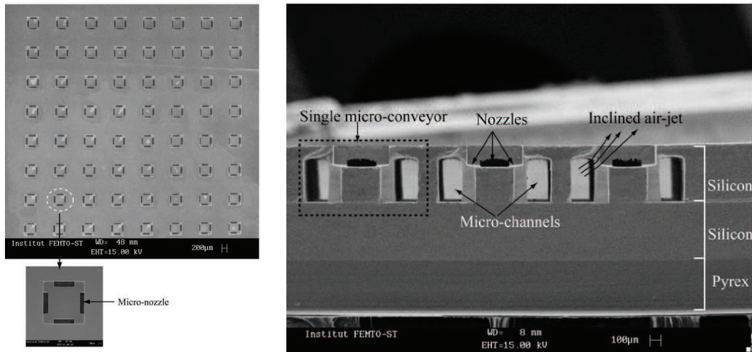
FIGURE 5.7 – Images MEB (microscope à balayage électronique) du micro-conveyeur développé par Zeggari et al. [75].
