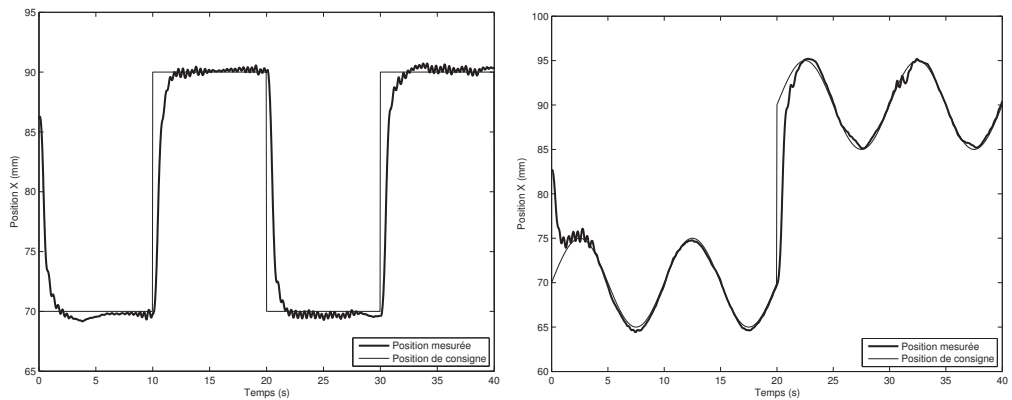
(c) Réponse expérimentale du système à une succession d'échelons.
