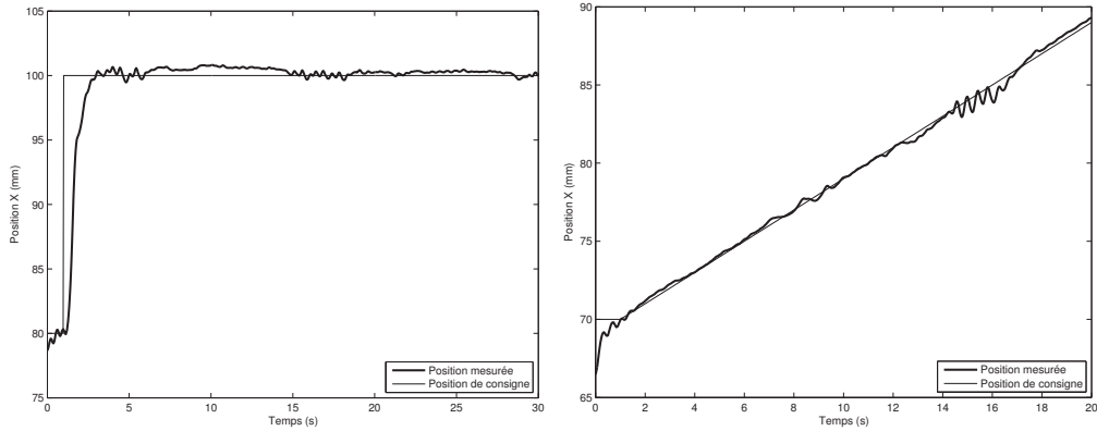
(a) Réponse expérimentale du système à un échelon d'amplitude 20 mm.
