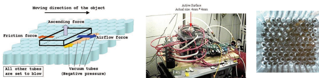
FIGURE 2.20 – Le système développé par Ku et al. [41] génère des jets d'air de différentes pression permettant de déplacer et de faire léviter des objets.
