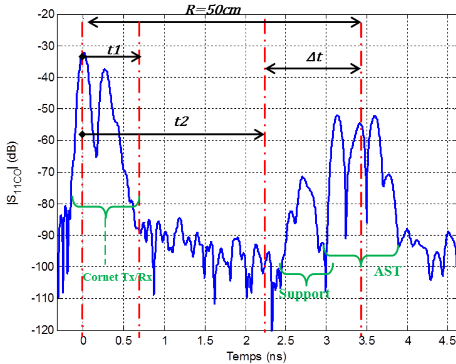
Figure 2. Résultat de la mesure de la réflexion temporelle.
