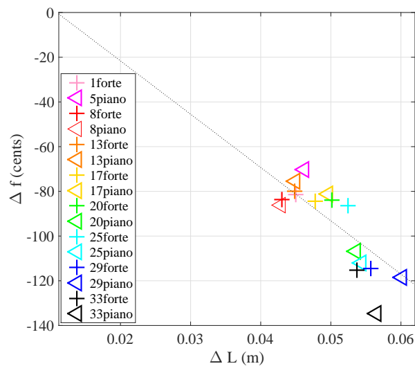
FIGURE 2.18 – Figure représentant des écarts entre la fréquence de résonance de la flûte sans flûtiste et pour différentes positions des lèvres \Delta f_0 (en cents) en fonction de \Delta L .
