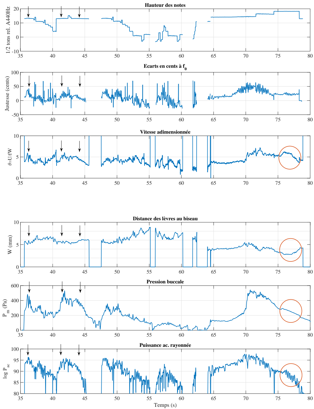
FIGURE 8.43 – Jeu de Syrix par le musicien 2, sont représentés : la hauteur des notes jouées, l'écart de celles-ci à un diapason basé sur le La à 440Hz, en cents, la vitesse de jet adimensionnée \theta , la pression buccale P_m , la distance des lèvres au biseau W et la puissance acoustique rayonnée. Les Si \flat du second registre sont repérés par des flèches, et le Mi \flat de la dernière phrase par une ellipse.
