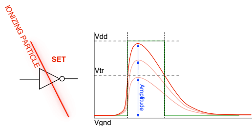
Figure 1.5: Blocage Électrique
