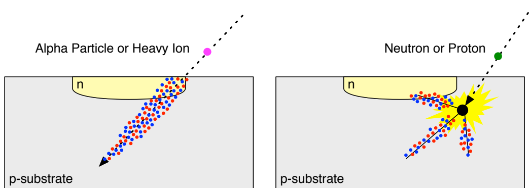
Figure 1.4: Méthodes d'interactions de particules : Ionisation Directe et Indirecte
