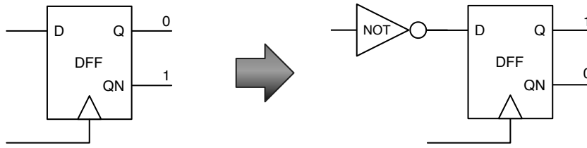
Figure 1.13: Optimisation par l'inversion d'état
