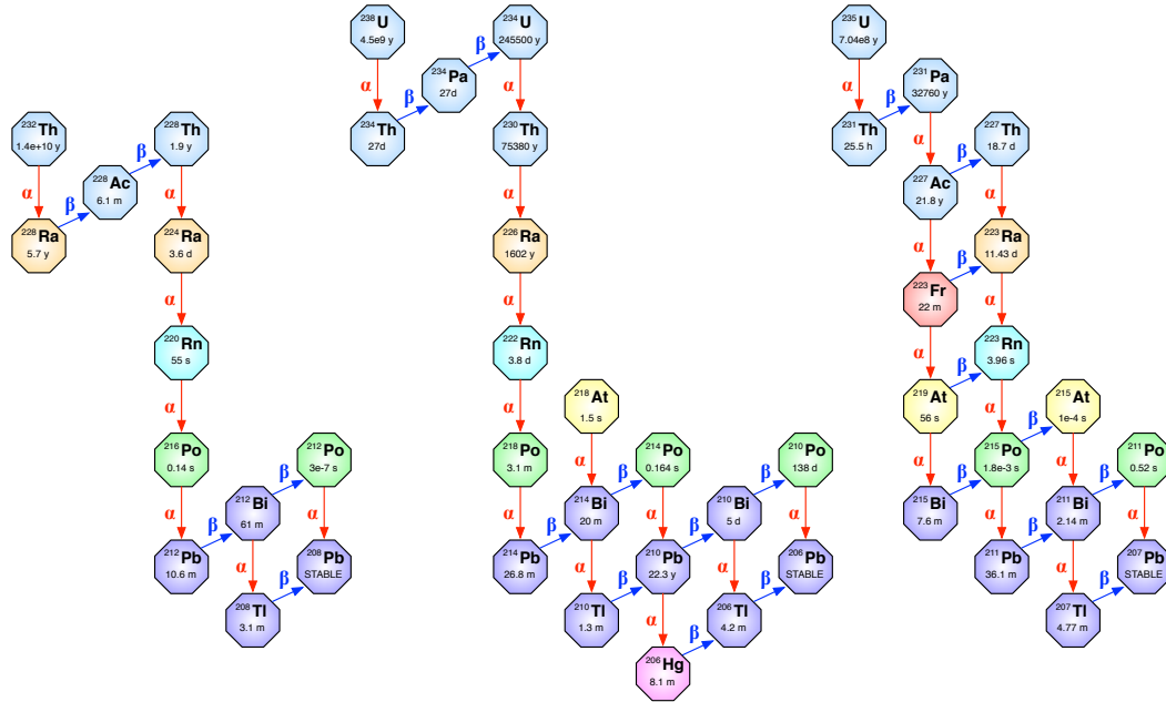
Figure 1.3: Les désintégrations radioactives
