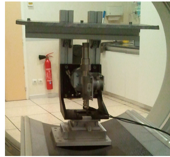
(b) Photo du dispositif dans l'anneau du scanner
