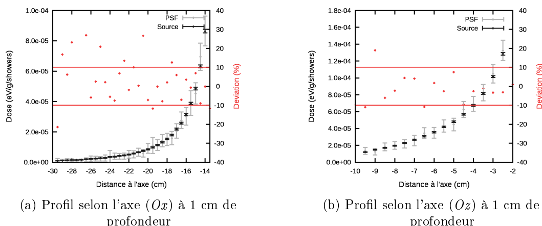
FIGURE 3.27 – Profils de dose dans la cuve à eau à l'extérieur du champ pour une tension de 120 kV, un SFOV de 32 cm et une collimation de 4.2 cm
