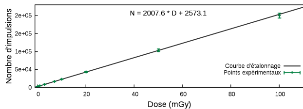
(d) Césium
