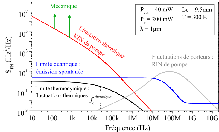
FIGURE 2.9 – Représentation des différentes limitations de la densité spectrale de bruit de fréquence dans le VeCSEL.
