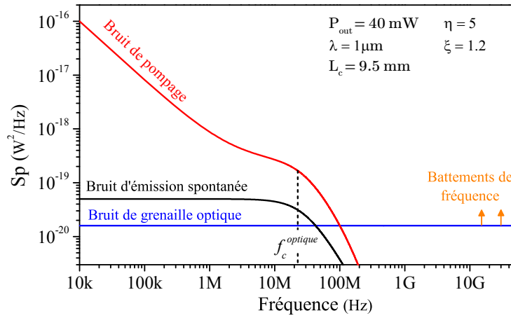
FIGURE 2.7 – Représentation des différentes limitations en bruit d'intensité pour un VeCSEL. Pour la limitation par le bruit de pompe, on a considéré le bruit typique d'une diode de pompe monomode.
