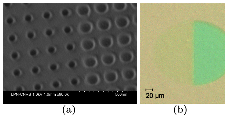
FIGURE 2.25 – a) Image au microscope MEB du cristal photonique pour ff = 0.3 et ff = 0.6 . — b) Image au microscope optique montrant l'effet des deux zones de test à cause de la différence d'indice effectif.
