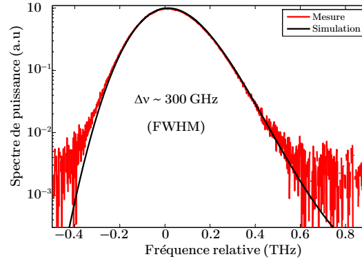
FIGURE 4.3 – Spectre optique du VeCSEL sans mode émettant autour de 1.07\mu\text{m} : la largeur à mi-hauteur et de \sim 300 GHz ( \sim 1.15 ).
