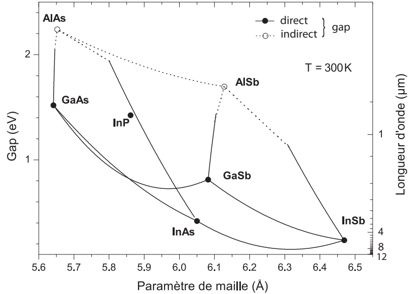
FIGURE 1.5 – Diagramme d'énergie de bande interdite en fonction du paramètre de maille pour les matériaux III-V.
