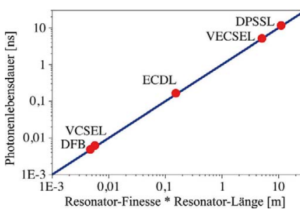
Bild 2: Photonlebensdauer verschiedener Lasertechnologien: Mikroresonator-VCSEL, 300 µm DFB, 1 cm ECDL, 1 cm VeCSEL und 1 m Festkörperlaser (z.B. TiSa)
