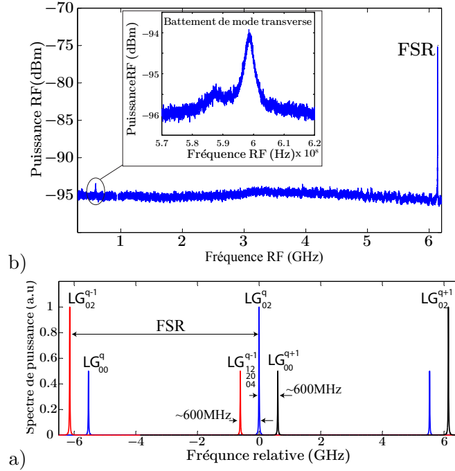
FIGURE 3.5 – a) Mesure du spectre radio fréquence de bruit d'intensité de VeCSEL à 1 \mu\text{m} , émettant sur le mode transverse LG_{02} dégénéré, sur une gamme de fréquences allant jusqu'au premier harmonique des battements des modes longitudinaux. En zoom, le signal de battement dû aux modes transverses faibles (résolution 20 kHz). — b) Spectre théorique de la cavité froide du VeCSEL.
