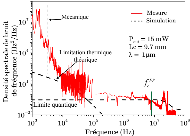
FIGURE 2.10 – Densité spectrale de bruit de fréquence du VeCSEL à 1\mu\text{m} . Les limitations théoriques de différentes origines sont indiquées. La limite théorique de bruit blanc a été calculée pour un facteur \alpha_h = 4 .
