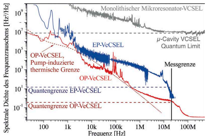
Bild 6: Spektrum des Frequenzrauschens für 10 mW EP-VeCSEL, 2 W OP-VeCSEL und 2 mW μ-Resonator-VCSEL
