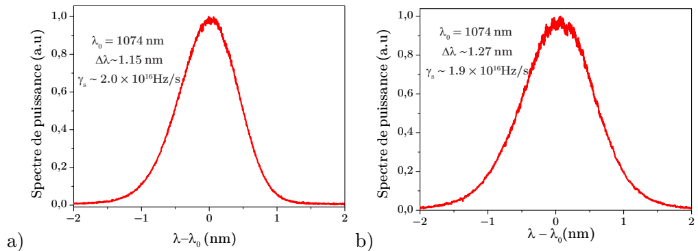
FIGURE 4.15 – Spectre optique de VeCSEL sans mode. –a) En configuration de cavité linéaire. –b) En configuration de cavité en anneau uni-directionnelle. Le spectre du laser est \sim 10\% plus large; cette largeur est équivalente à \sim 330 \text{ GHz} à \lambda = 1.074 \text{ nm} .
