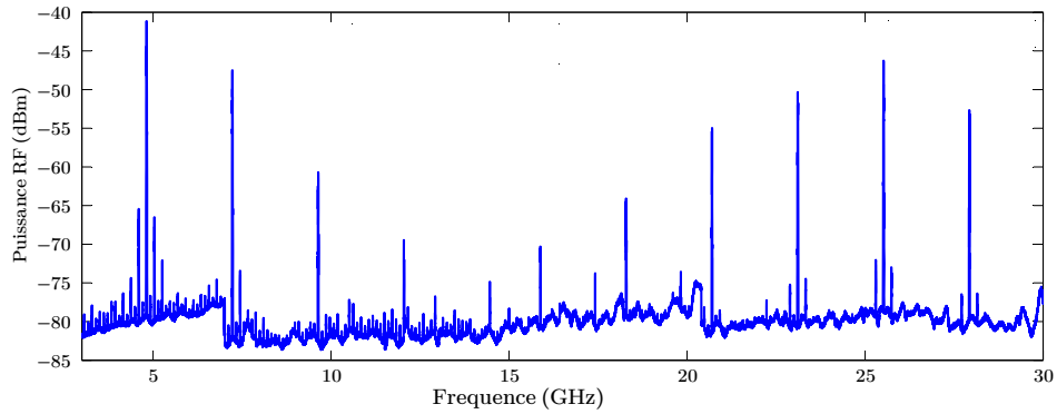
FIGURE 5.6 – Spectre RF du VeCSEL injecté par source mono-fréquence. La configuration de la cavité satisfait 1 \times f_s = 2 \times f_c avec f_c = 110\text{MHz} . Le spectre RF ne correspond pas à un fonctionnement impulsionnel à 220MHz.
