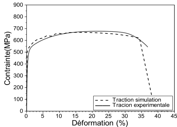
FIGURE 6.10 – Comparaison des propriétés mécaniques en traction monotone : courbe expérimentale et courbe approximée par le modèle Hansel Spittel après ajustement des paramètres.
