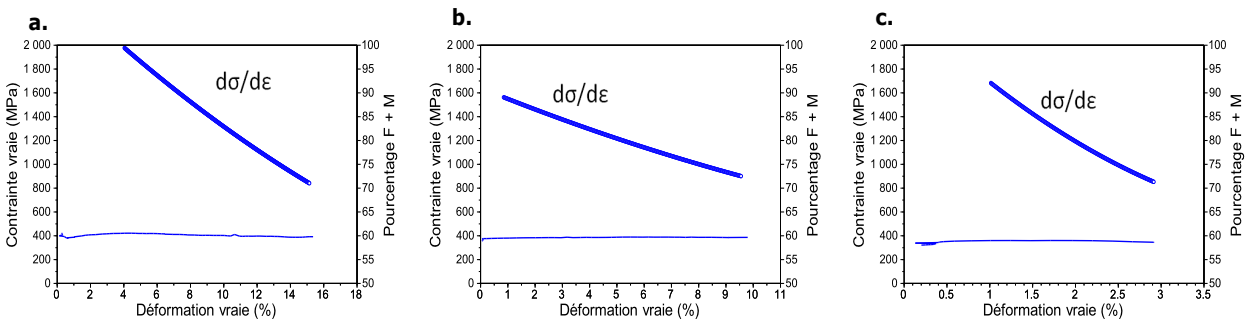
FIGURE 3.8 – Évolution du taux d'érouissage et du pourcentage de ferrite + martensite en fonction de la déformation pour l'alliage A a. sans pré-déformation, b. pré-déformé à 10 % et c. pré-déformé à 20 %.
