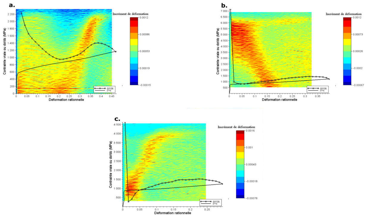
FIGURE 3.15 – Évolution de l'incrément de déformation et du taux d'écroutissage en fonction de la déformation pour l'alliage B a. non pré-déformé, b. après 10 % de pré-déformation et c. après 20 % de pré-déformation.
