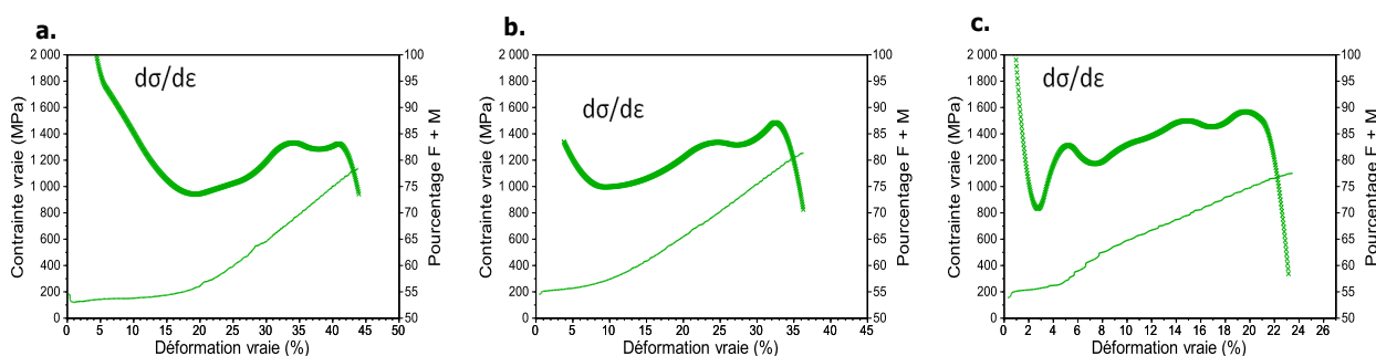
FIGURE 3.10 – Évolution du taux d'écroissage et du pourcentage de ferrite + martensite en fonction de la déformation pour l'alliage C a. sans pré-déformation, b. pré-déformé à 10 % et c. pré-déformé à 20 %
