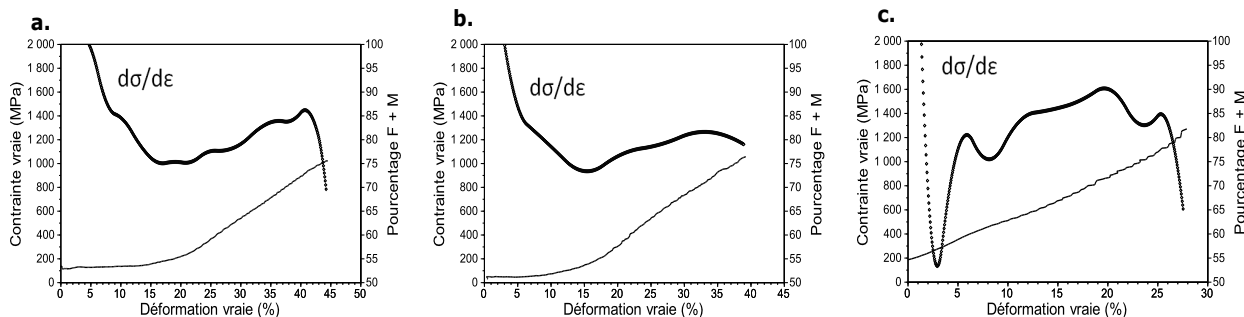
FIGURE 3.9 – Évolution du taux d'écroissage et du pourcentage de ferrite + martensite en fonction de la déformation pour l'alliage B a. sans pré-déformation, b. pré-déformé à 10 % et c. pré-déformé à 20 %
