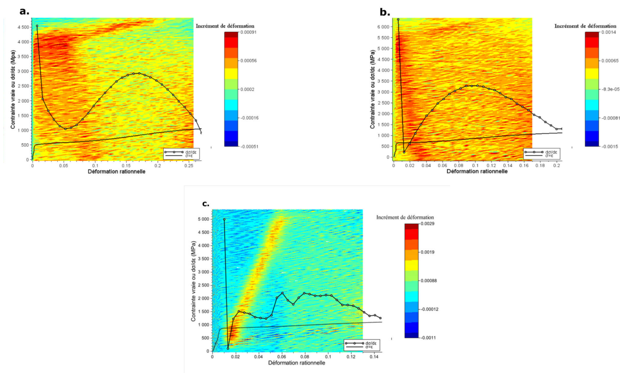
FIGURE 3.17 – Évolution de l'incrément de déformation et du taux d'érouissage en fonction de la déformation pour l'alliage D a. non pré-déformé, b. après 10 % de pré-déformation et c. après 20 % de pré-déformation.
