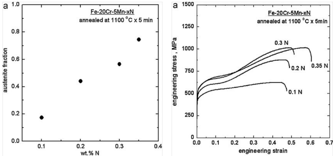
FIGURE 1.6 – Fraction de phase austénitique et courbes conventionnelles de traction pour différents teneurs en azote [CJHP12a]. Étude réalisée sur un acier inoxydable duplex.
