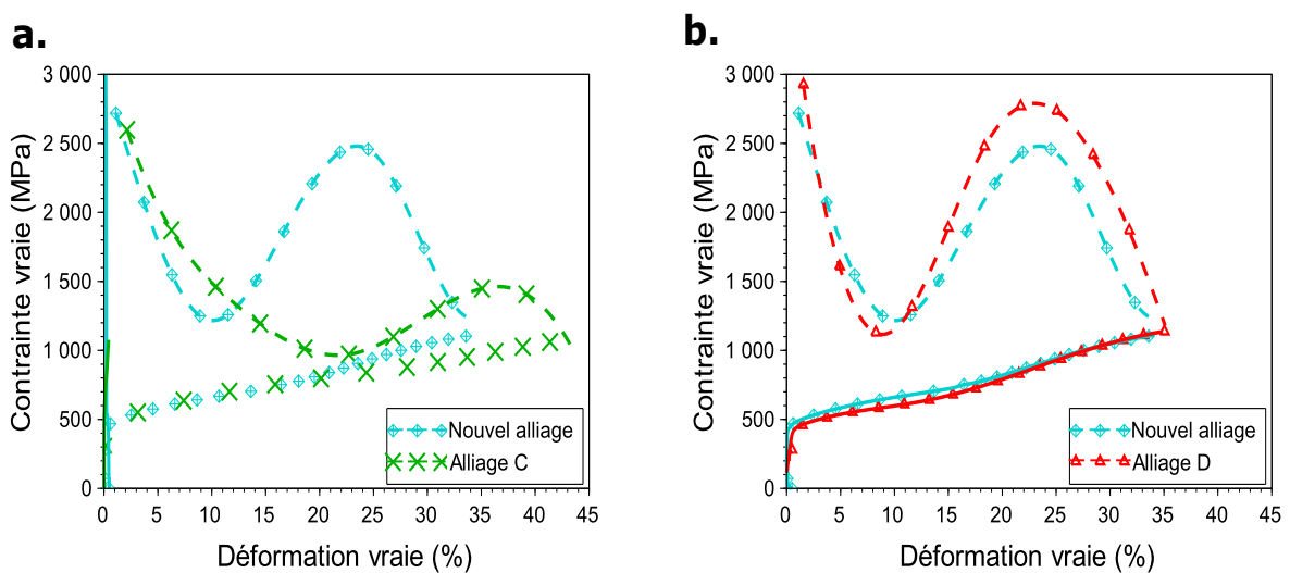
FIGURE 6.7 – Comparaison de l'évolution du taux d'écroissage entre le nouvel alliage et a. l'alliage C et b. l'alliage D.
