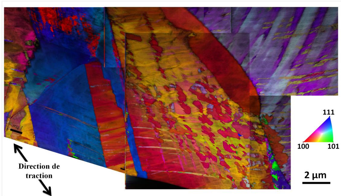
FIGURE 4.11 – Cartographie ACOM d'orientations cristallographiques de la zone analysée après une déformation de 20 %.
