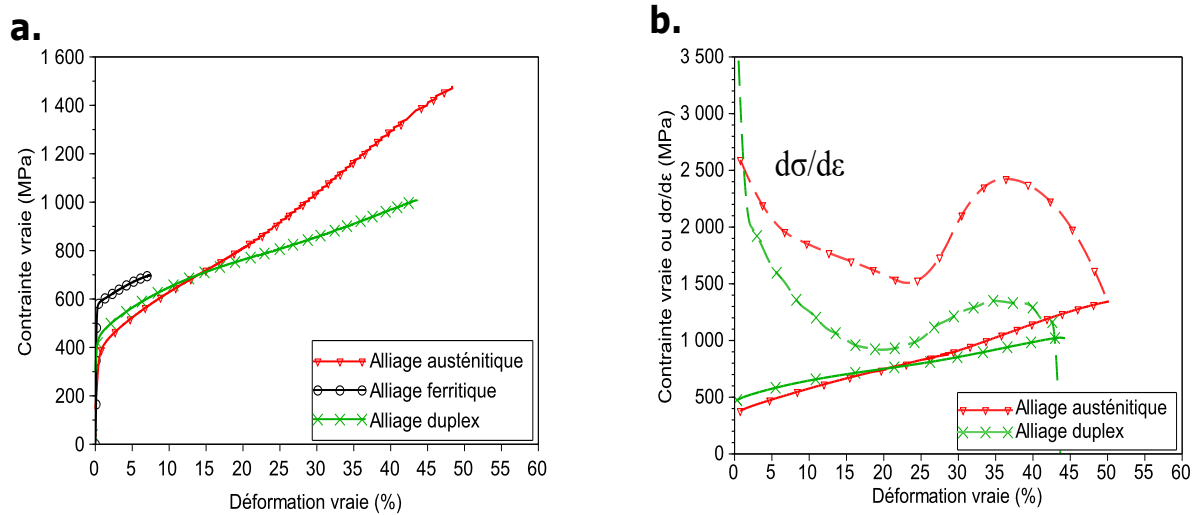
FIGURE 4.5 – a. Courbe de traction rationnelle pour les nuances austénitique, ferritique et duplex après traitement thermomécanique. b. Courbe de traction rationnelle et évolution du taux d'érouissage pour les nuances austénitique et duplex.
