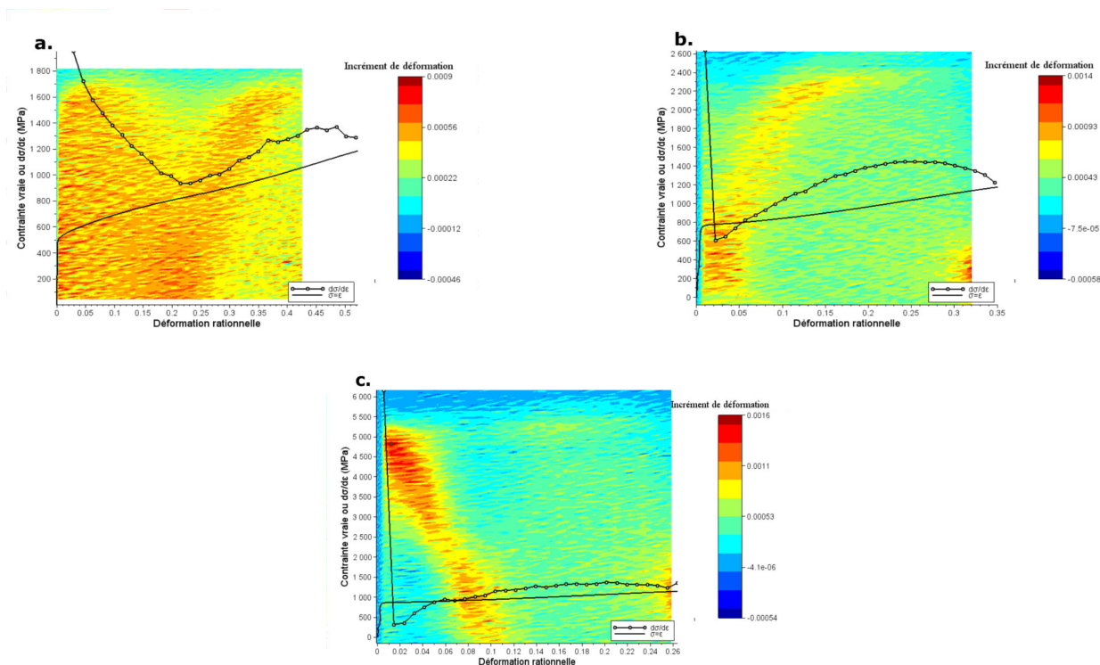
FIGURE 3.16 – Évolution de l'incrément de déformation et du taux d'érouissage en fonction de la déformation pour l'alliage C a. non pré-déformé, b. après 10 % de pré-déformation et c. après 20 % de pré-déformation.
