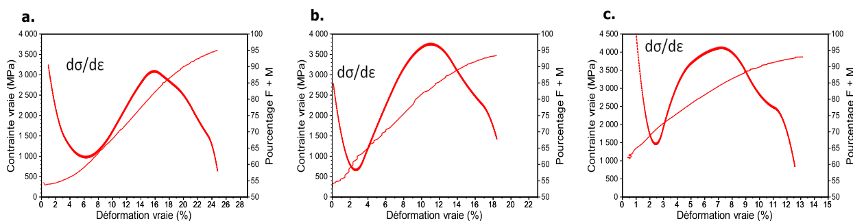
FIGURE 3.11 – Évolution du taux d'écroissage et du pourcentage de ferrite + martensite en fonction de la déformation pour l'alliage D a. sans pré-déformation, b. pré-déformé à 10 % et c. pré-déformé à 20 %
