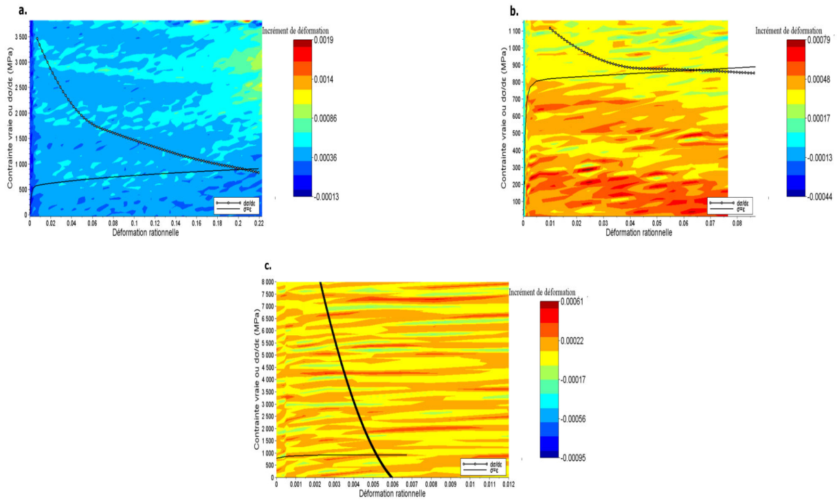
FIGURE 3.14 – Évolution de l'incrément de déformation et du taux d'écroutissage en fonction de la déformation pour l'alliage A a. non pré-déformé, b. après 10 % de pré-déformation et c. après 20 % de pré-déformation.
