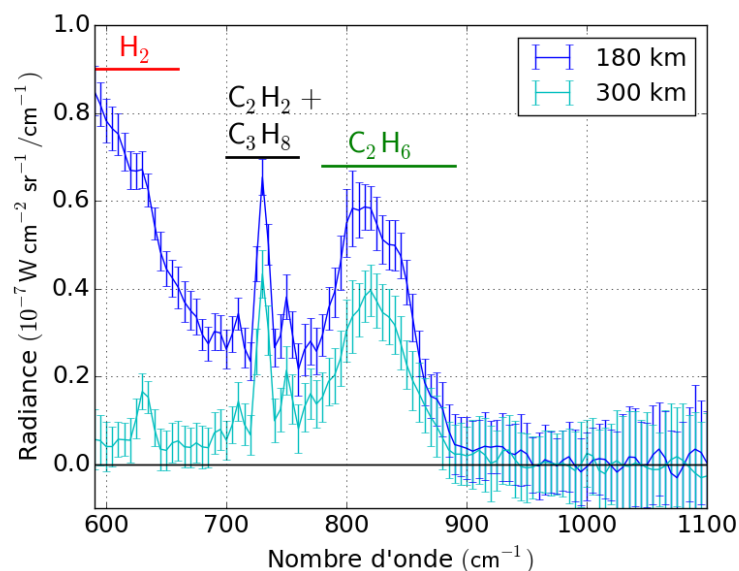
FIGURE 2.6 – Exemples de spectres CIRS obtenus après co-addition mesurés à 30°N ( L_S = 12^\circ ) par FP3, acquis respectivement aux altitudes 180 km (8.4 hPa) et 300 km (0.7 hPa). Les deux spectres ont une résolution spectrale de 7.5 \text{ cm}^{-1} .
