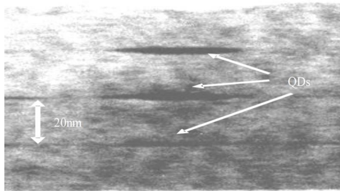
Figure 2.17. Image TEM des bâtonnets quantiques au niveau de la couche active: Courtesy of G. Patriarche, CNRS LPN
