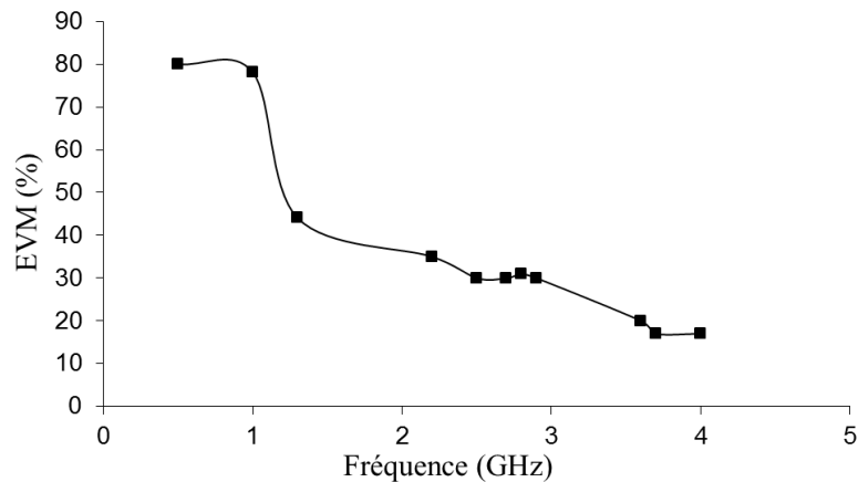
Figure 2.39. EVM en fonction de la fréquence de modulation (directe)
