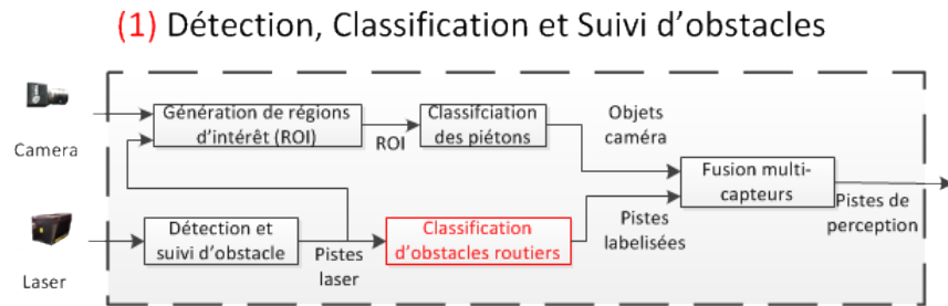
FIGURE 3.6: Architecture du système de perception des usagers vulnérables
