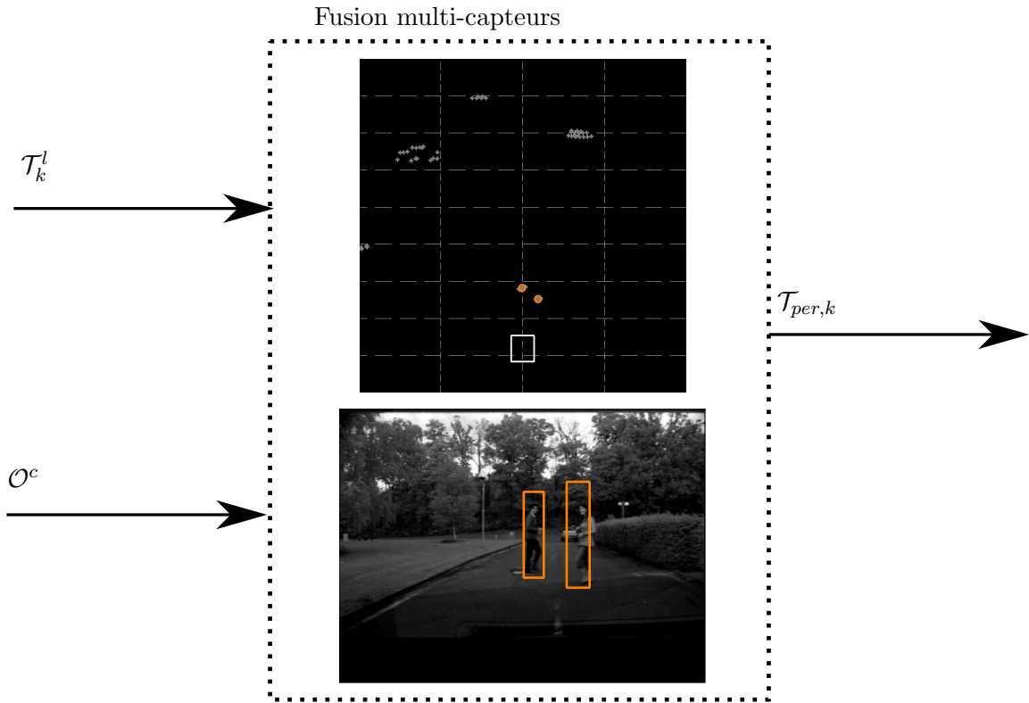
FIGURE 3.11: Fusion multi-capteurs
