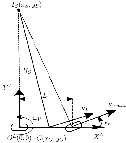
FIGURE 4.4: Modèle bicyclette
