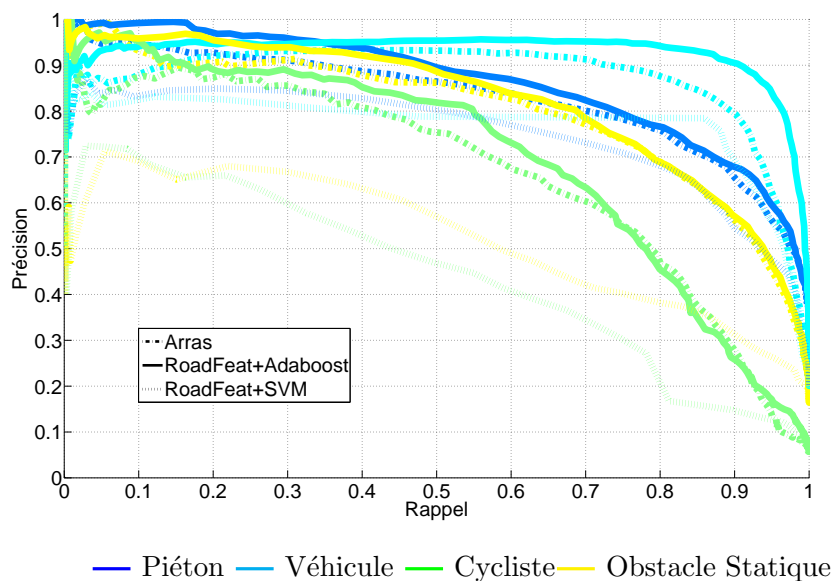
FIGURE 6.6: Précision-Rappel
