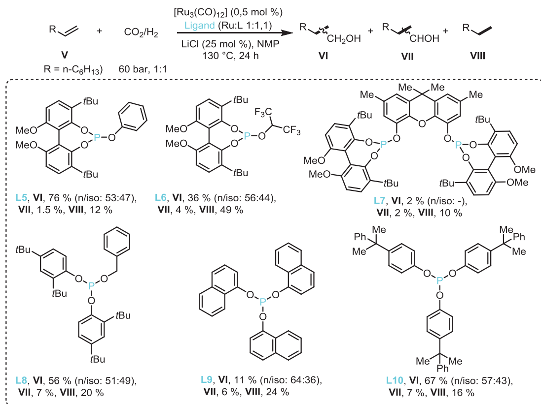
Schéma 168 : Évaluation des ligands phosphites dans la réaction d'hydroformylation du 1-octène avec le \text{CO}_2 .
