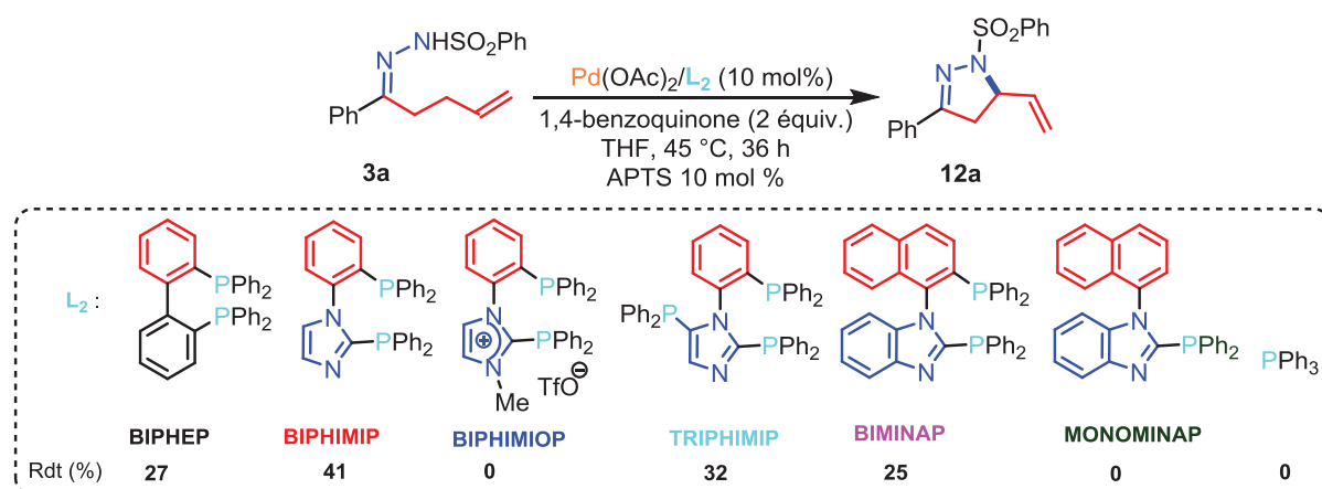
Schéma 88 : Différents ligands phosphorés testés en N-allylation intramoléculaire CH-oxydante catalysée par le palladium en présence d'APTS et de l'hydrazone 3a cristallisée.
