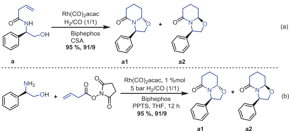
Schéma 137 : Réactions domino “cyclohydrocarbonylation/cyclisation” (a) et réaction domino multi-composant (b).
