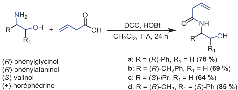
Schéma 136 : Synthèse d'amides linéaires par couplage peptidique à partir d'amino-alcools.
