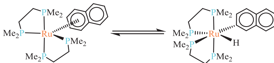
Schéma 3 : Synthèse d'un complexe aryl-ruthénium par activation d'une liaison C(sp 2 )-H.
