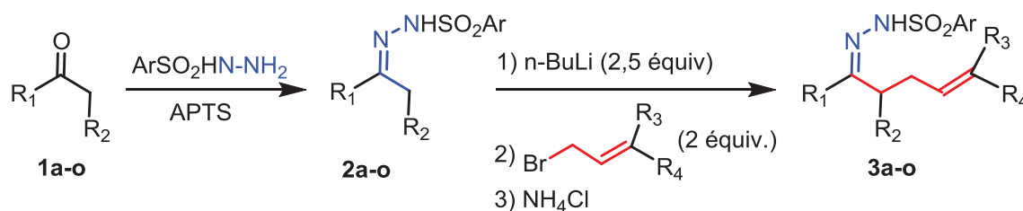
Schéma 66 : Synthèse d'hydrazones C-homoallyliques 3a-o .
