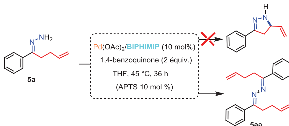
Schéma 97 : Tentatives de cyclisation de l'hydrazone C-homoallylique 5a en 5-vinyl-2-pyrazoline (conditions "acides").
