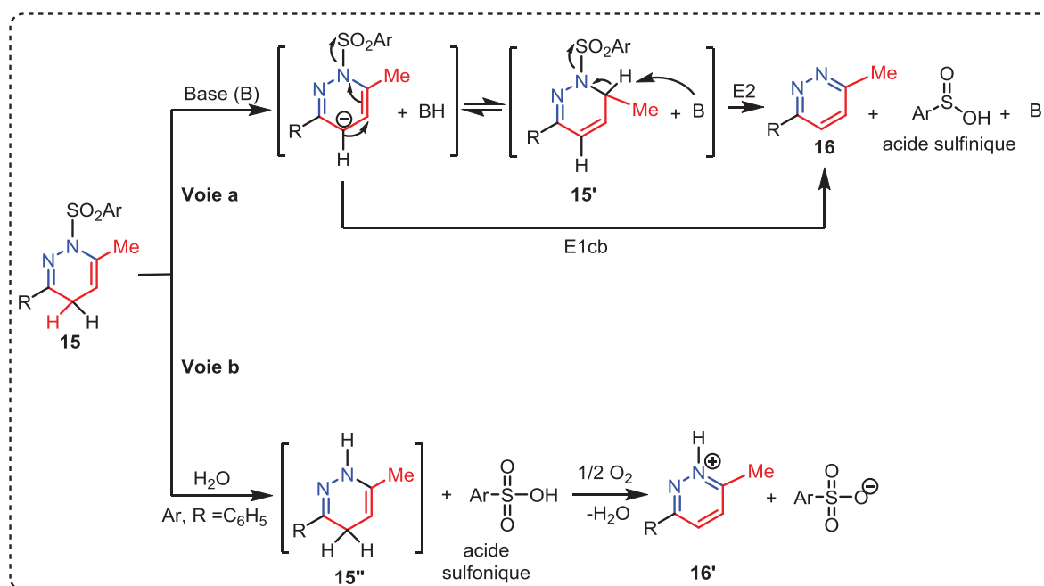
Schéma 129 : Propositions de mécanisme pour la formation des pyridazines 16 à partir des 1,4-dihydropyridazines 15 : a) suivant un processus d'élimination; b) suivant le processus d'hydrolyse et d'oxydation.
