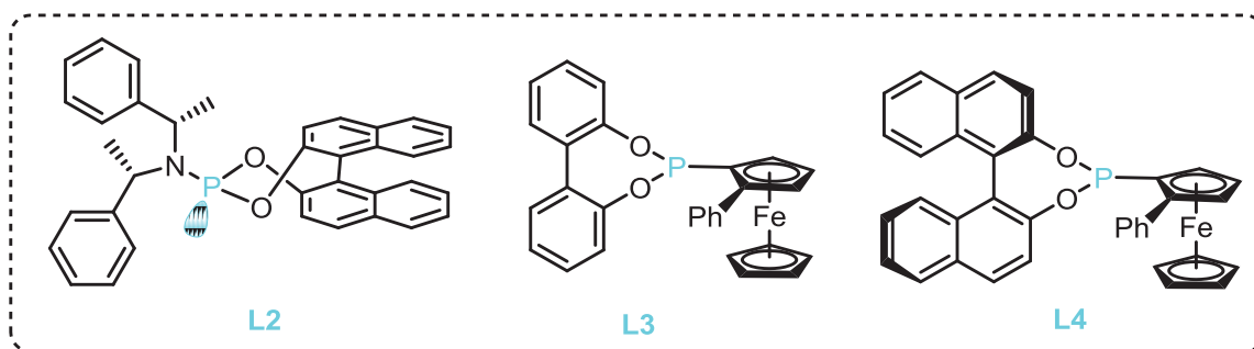
Schéma 167 : Utilisation du ligand phosphoramidite L2 et des ligands ferrophites L3 et L4 dans des réactions d'addition 1,2 de \text{AlMe}_3 sur le benzaldéhyde et 1,4 d'organo-alluminium sur la cyclohexènone.
