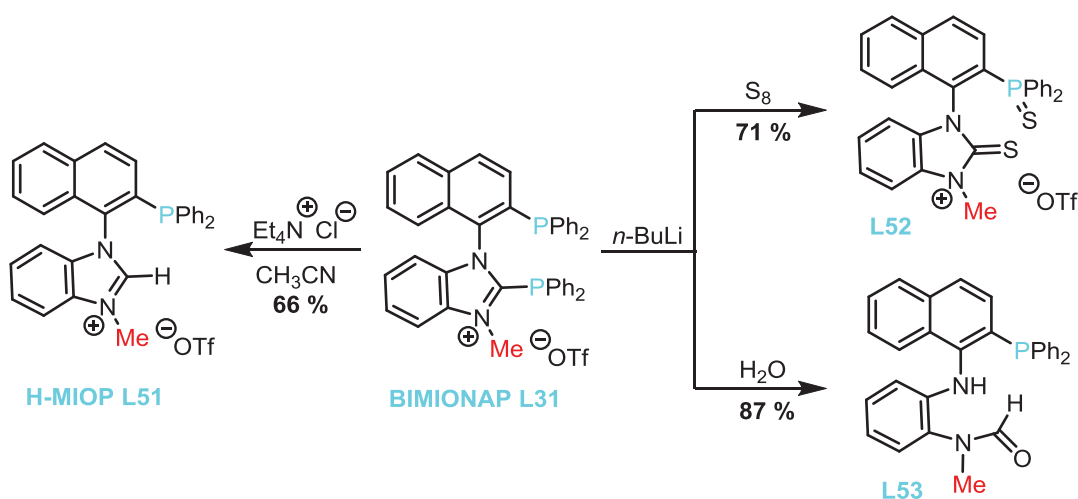
Schéma 188 : Coupure de la liaison N 2 C-P de la BIMIONAP par un anion chlorure ou butyle, suivie d'un traitement par une source protonique (CH 3 CN, H 2 O) ou par du soufre élémentaire.
