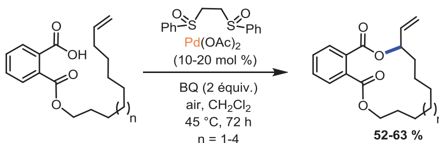
Schéma 47 : Synthèse des macrolactones par alcoxylation allylique CH oxydante directe.
