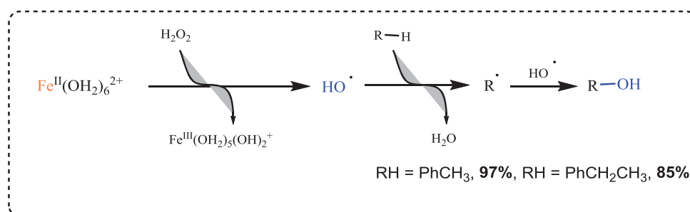
Schéma 11: Oxydation d'alcane par le réactif de Fenton (non organométallique).
