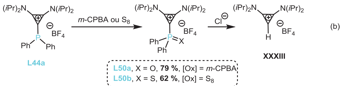
Schéma 187 : Synthèse des chalcogénoimidazoliophosphines L49a-b et chalcogénocyclopropéniophosphines L50a-b à partir des carbéniophosphines correspondantes.
