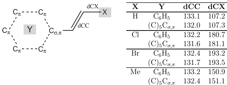
FIGURE 3.6 – Comparaison de distances (en pm) optimisées pour différents substituants (X=H, Cl, Br, Me) d’une double liaison liée à un système sans pseudo atome (Y=C 6 H 5 ) et un système avec pseudo atomes (Y=(C) 5 C \sigma,\pi ). La distance entre Y et la double liaison est fixée.
