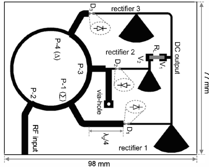
Figure II. 16. Schéma du convertisseur RF-DC double fréquences [II.23]
