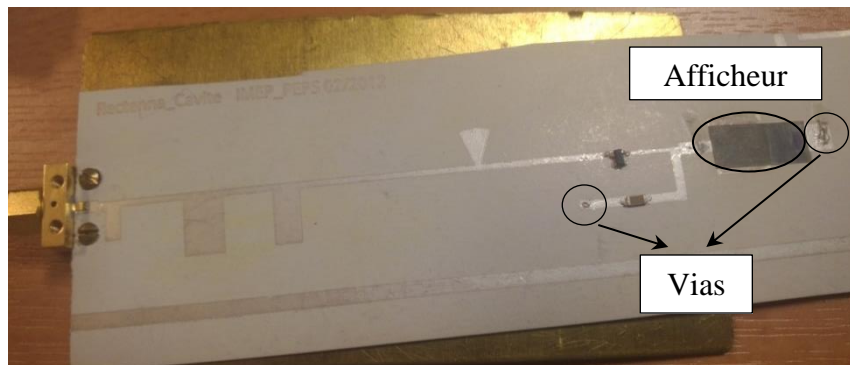
Figure IV. 19. Circuit de conversion RF-DC imprimé sur papier SP3
