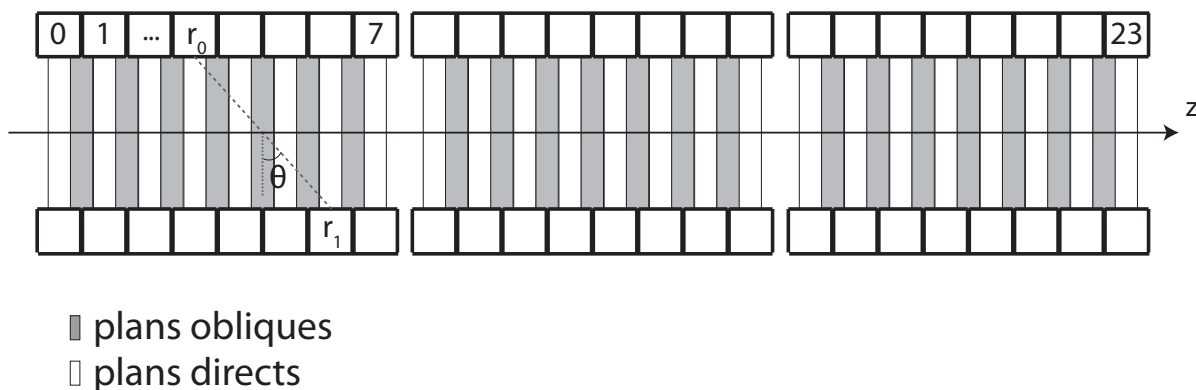
Figure 3.5 Représentation des coordonnées 4D décrivant un élément ou bin des sinogrammes 3D : s [-n_{\max}, +n_{\max}] , \theta [-23, +23] , \phi [0, 79] et z [0, 46] (Egger et al., 1998).
