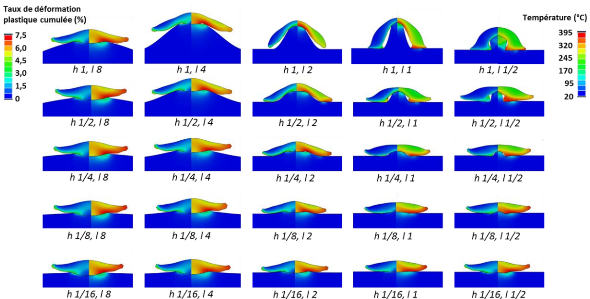
Figure 4-17 : Résultats de simulation d'impact (déformation plastique cumulée, à gauche, et température, à droite) d'aluminium pur 1050 sur substrat d'aluminium 2024-T3 pour une vitesse d'impact de 700 m.s^{-1} .
