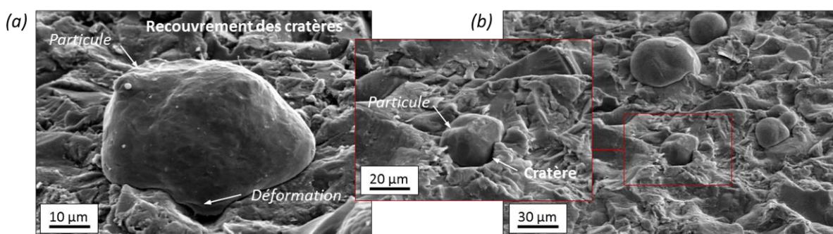
Figure 3-26 : Images MEB en électrons secondaires de particules d'aluminium pur 1050 (30 \mu\text{m} de diamètre moyen) déposées sur substrat d'aluminium 2024-T3 sablé : (a) finement et (b) grossièrement.
