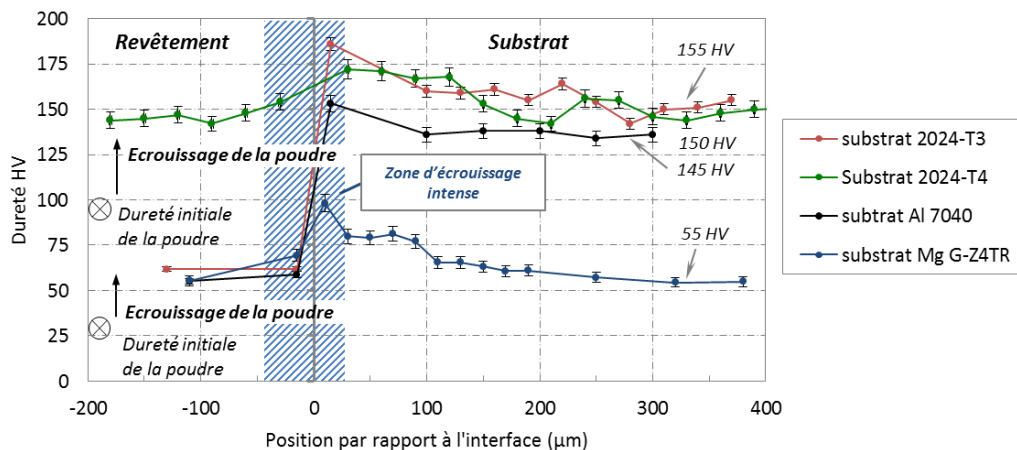
Figure 7-7 : Profils de dureté du système revêtement-substrat, depuis la surface du revêtement d'aluminium pur 1050 et d'aluminium 2024 jusque dans les substrats bruts d'aluminium 2024-T3, 2024-T4 et 7040-T6 et de magnésium G-Z4TR.
