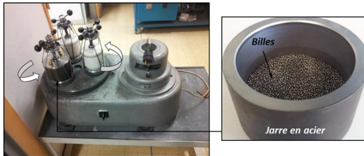
Figure A-2 : Broyeur pour la mécano-synthèse, équipement LIFCO Industries.
