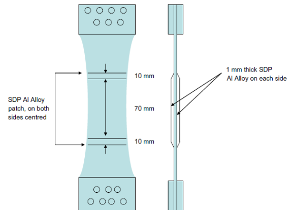
Figure 7-32 : Eprouvettes en aluminium 2024-T3 sollicitées en traction avec l'ajout d'un revêtement d'aluminium élaboré par cold spray [JON11].
