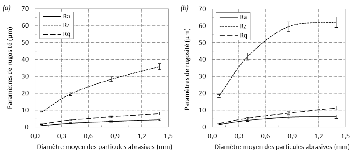
Figure 4-2 : Influence de la granulométrie moyenne des particules abrasives sur les paramètres de rugosité Ra, Rq et Rz dont les valeurs sont issues (a) du modèle empirique de Slatineanu [SLA11] et (b) de l'analyse profilométrique.
