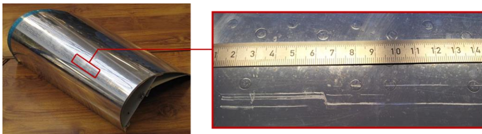
Figure 7-38 : Traces d'usure par impact en vol et au cours de la maintenance sur un bord d'attaque en aluminium 2024-T3 plaqué par de l'aluminium pur 1050, d'épaisseur 80-100 \mu m [CSA12].
