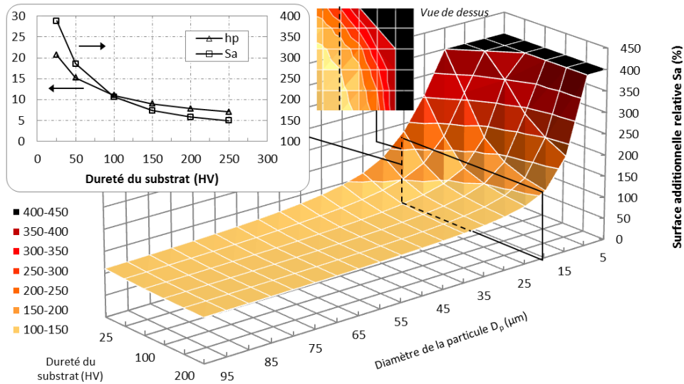
Figure 7-15 : Evolution de la surface additionnelle relative S_a en fonction du diamètre D_p de la particule (sphérique et indéformable) et de la dureté HV du substrat pour une vitesse de particule de 650 \text{ m}\cdot\text{s}^{-1} .
