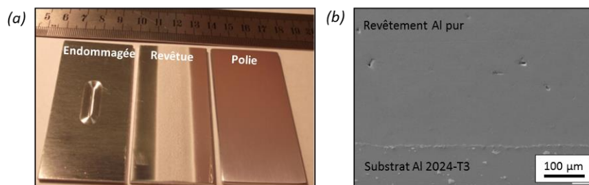
Figure 7-29 : (a) Étapes de réparation de l'éprouvette d'aluminium 2024-T3, endommagée, revêtue puis polie et (b) image MEB en coupe, en électrons secondaires, de l'interface d'aluminium pur et du substrat d'aluminium 2024-T3 [YAN14].
