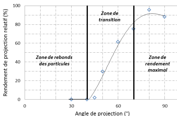
Figure 3-23 : Evolution du rendement relatif de revêtements d'aluminium pur 1050 déposés sur substrats d'aluminium 2024-T3 en fonction de l'angle de projection, cas d'un recouvrement de la surface du substrat.
