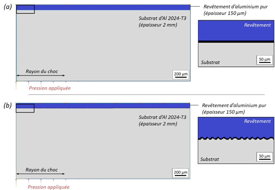
Figure 6-19: Modèles numériques 2D maillés du système revêtement d'aluminium pur 1050 sur substrat d'aluminium 2024-T3, cas d'une interface (a) plane et (b) rugueuse, utilisés pour la simulation de la propagation d'onde par choc laser.
