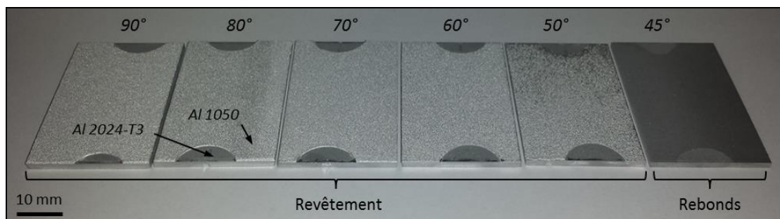
Figure 3-22 : Photographies des revêtements d'aluminium pur 1050 sur substrats d'aluminium 2024-T3 en fonction de l'angle de projection allant de 90° à 45°.
