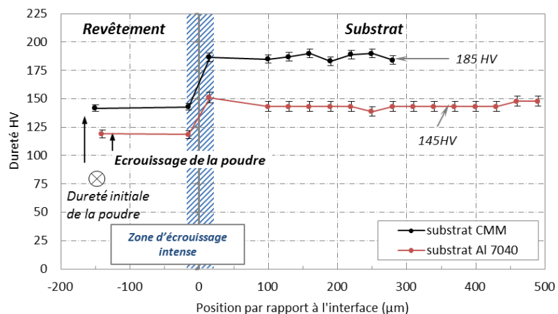
Figure 7-20 : Profils de dureté du système revêtement-substrat, depuis la surface des revêtements composites d'Al-SiC jusque dans les substrats bruts d'aluminium 7040 et de CMM.
