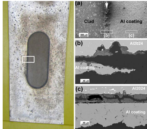
Figure 7-34 : Image de l'éprouvette réparée après une immersion pendant 480 h dans un bain corrosif, en vue de dessus (a gauche), (a) présence de corrosion par piqûre à la jonction revêtement/couche protectrice initiale, indiquée par la flèche blanche et (b et c) images MEB en coupe, en électrons secondaires, de cette jonction [YAN14].
