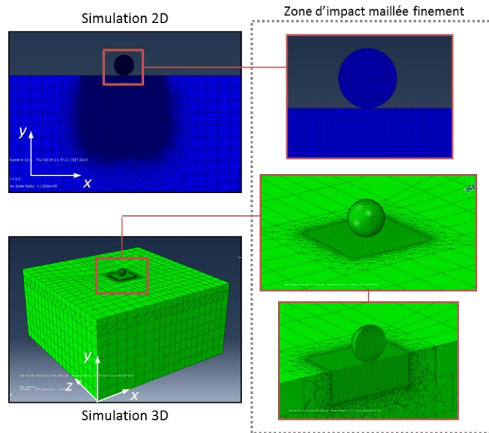
Figure 5-1 : Présentation du maillage utilisé pour les simulations 2D et 3D sur substrat plan.
