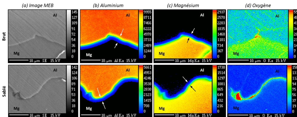
Figure 7-6 : Cartographies chimiques issues de l'analyse WDS de l'interface d'un revêtement d'aluminium pur 1050 sur un substrat de magnésium G-Z4TR, dont l'état de surface avant projection est brut (en haut) et sablé (en bas) : (a) image MEB, (b) teneur en Al, (c) teneur en Mg et (d) teneur en O.
