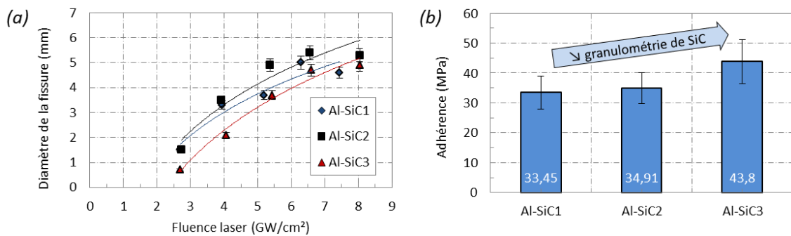
Figure 7-18 : Résultats d'adh rence des rev tements composites Al-SiC, d pos s sur un substrat d'aluminium 7040, en fonction de la granulom trie du SiC, mesur s (a) par choc laser et (b) par traction plots coll s.
