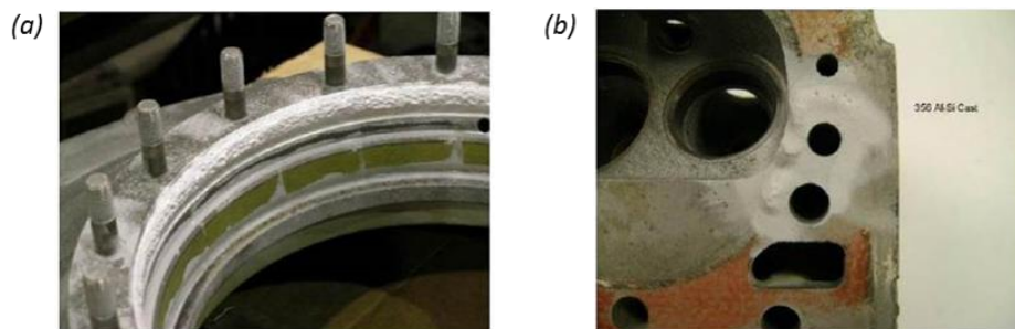
Figure 7-31 : Exemples de pièces réparées par cold spray : (a) revêtement de magnésium sur substrat de magnésium pour une pièce d'hélicoptère et (b) revêtement d'Al-Al 2 O 3 sur substrat d'Al-Si 356 constituant le bloc moteur [JON11].
