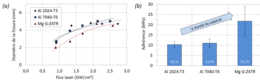
Figure 7-9 : Résultats d'adhérence déterminés (a) par choc laser et (b) par traction de plots collés, des revêtements d'aluminium pur 1050 déposés sur substrats bruts de magnésium G-Z4TR, d'aluminium 2024-T3 et 7040-T6, montrant l'influence de la dureté du substrat pour des paramètres de projection fixés.
