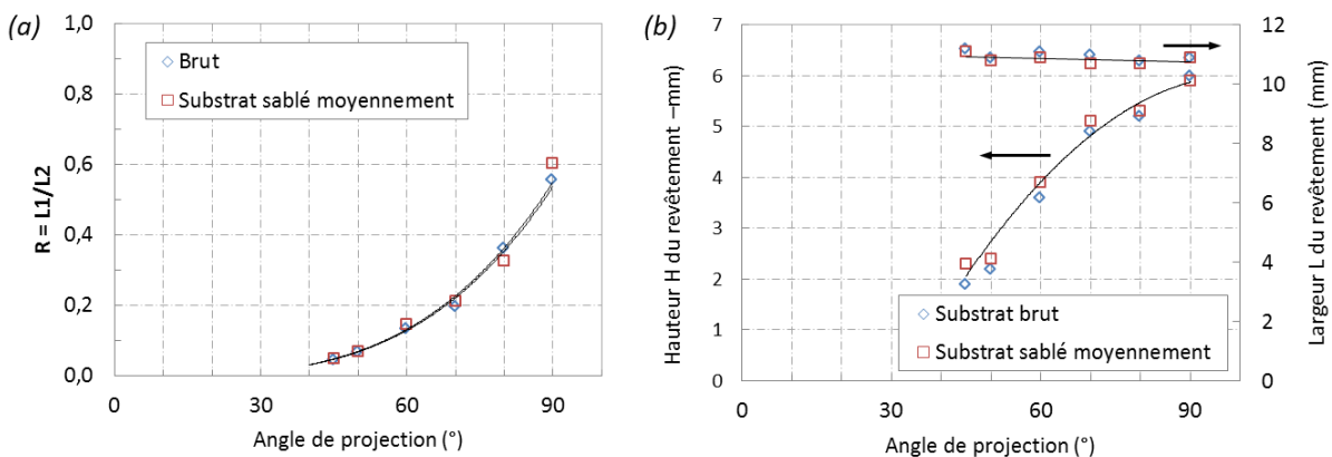
Figure B-3 : Evolution des dimensions géométriques du cordon de projection (a) du rapport R = L1/L2 et (b) de la hauteur L et de la hauteur H du cordon, en fonction de l'angle de projection.
