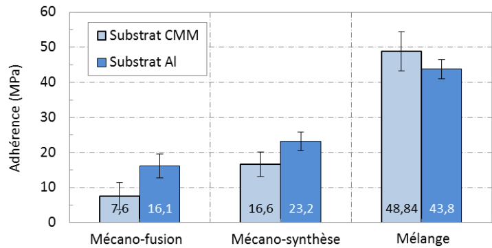
Figure 7-17 : Résultats d'adhérence mesurés par traction plots collés en fonction du procédé d'élaboration de la poudre CMM, pour deux types de substrats : CMM (aluminium 2009 + SiC) et aluminium 7040.
