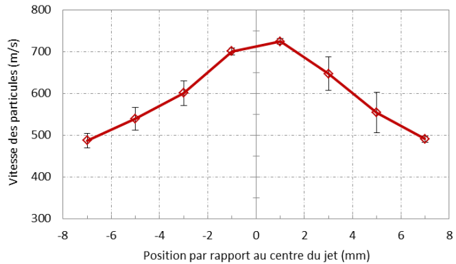
Figure 3-35 : Evolution de la vitesse des particules d'aluminium pur 1050 grossières et sphériques (30 \mu\text{m} ) dans le jet cold spray depuis le centre jusqu'en périphérie.
