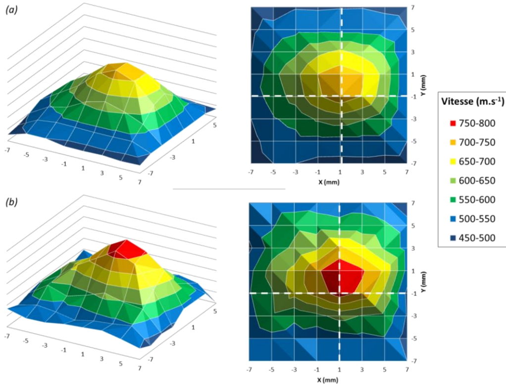
Figure 3-34 : Vue 3D et vue de dessus de la cartographie des vitesses des particules d'aluminium pur (a) 1050 grossières et sphériques (30 \mu\text{m} ) et (b) 1070 fines (10 \mu\text{m} ) dans un jet cold spray.
