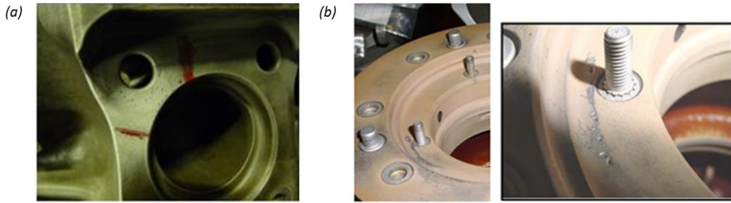
Figure 7-35 : (a) Cas 1, corrosion sur une zone d'attache d'une servocommande sur un carter en alliage de magnésium G-Z4TR et (b) Cas 2, carter en alliage de magnésium G-Z4TR avec la présence de traces de corrosion [CSA12].
