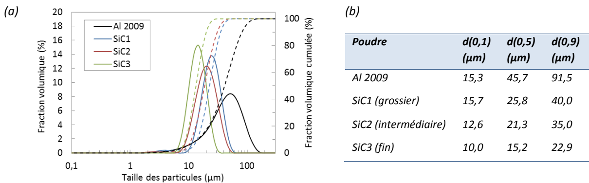
Figure 2-7 : (a) Répartition granulométrique en volume et (b) diamètres caractéristiques des poudres d'aluminium 2009 et de la poudre céramique SiC.
