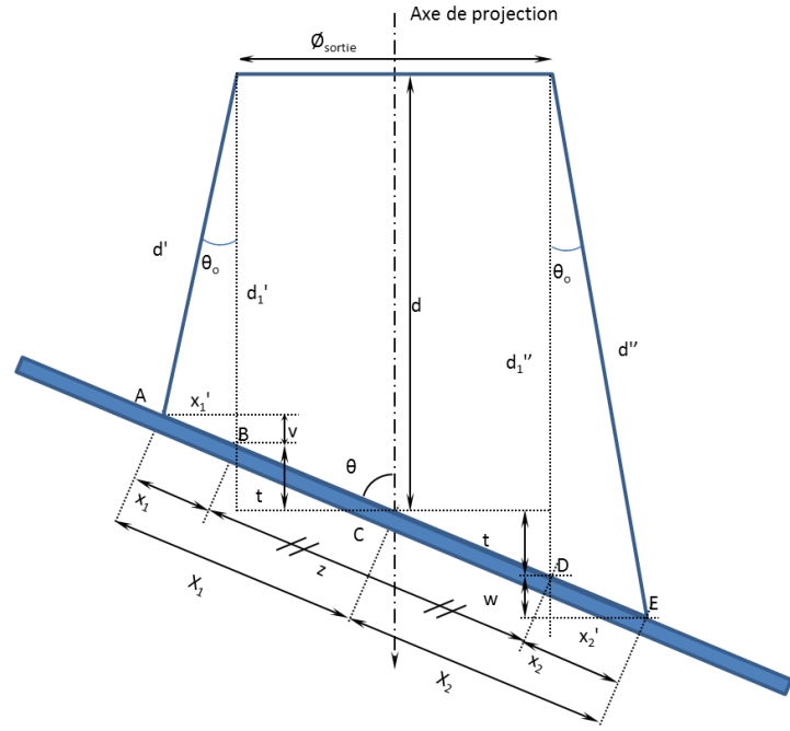
Figure C-2 : Schéma du flux de particules et de la zone d'impact du substrat générée par la buse, dimensions de la tache de projection.
