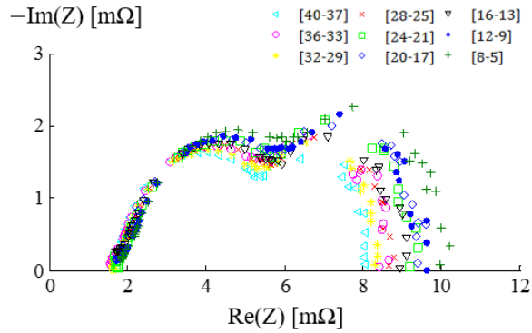
(a) cellules individuelles avant l'apparition du court-circuit
