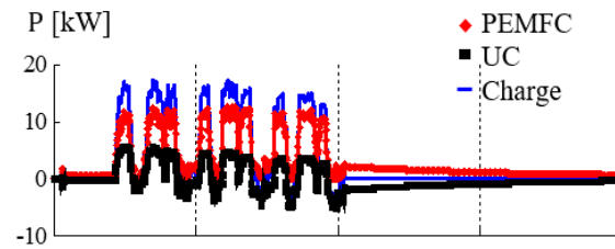
(a) Répartition de puissance
