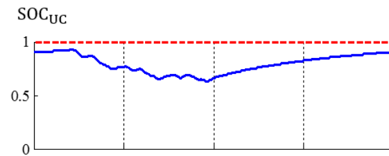
(b) UC état de charge
