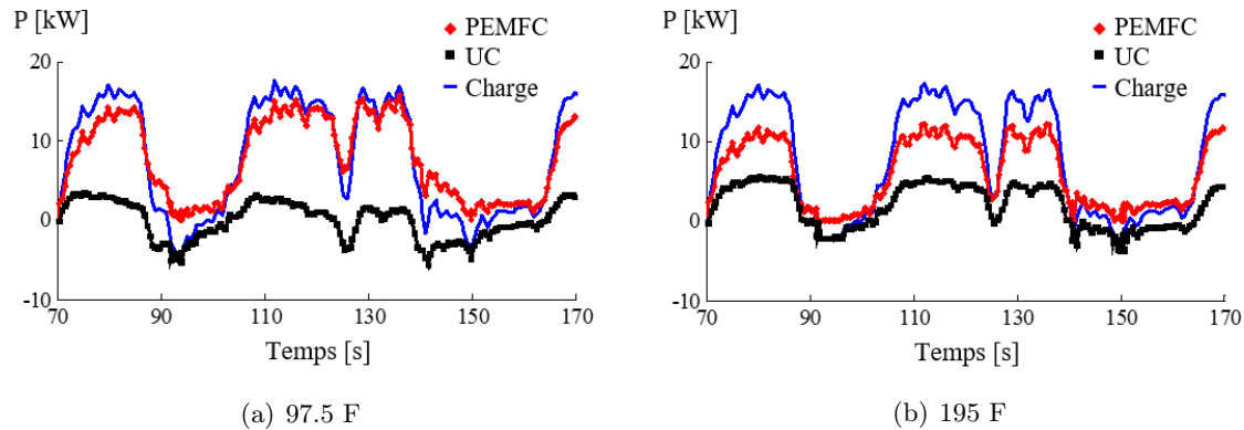
Figure 4.9 – Hybridation passive PEMFC/UC/Charge pour différents valeurs d'UCs
