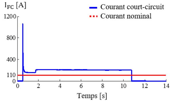
(a) Courant du stack
