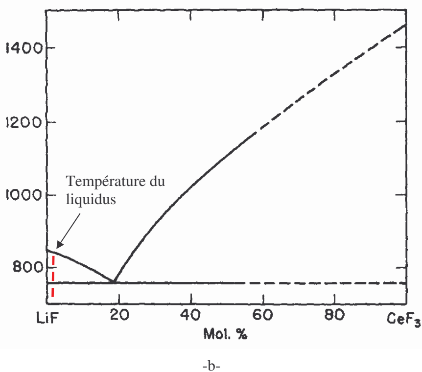
Figure 4.16 : Diagramme de phase des systèmes LiF-PbF 2 (cas -a-) et LiF-CeF 3 (cas -b-). D'après Roth et col. (1983) et Ernest et col. (1964).
