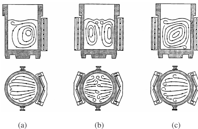
Figure 1.2 : Représentation de trois types de brasseur entourant une poche de traitement d'après Sundberg (1982).
