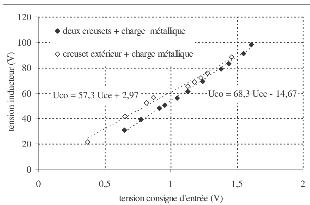
Figure 4.13 : Evolution de la tension efficace U_{co\text{eff}} aux bornes de l'inducteur en fonction de la tension de consigne d'entrée U_{ce} .
