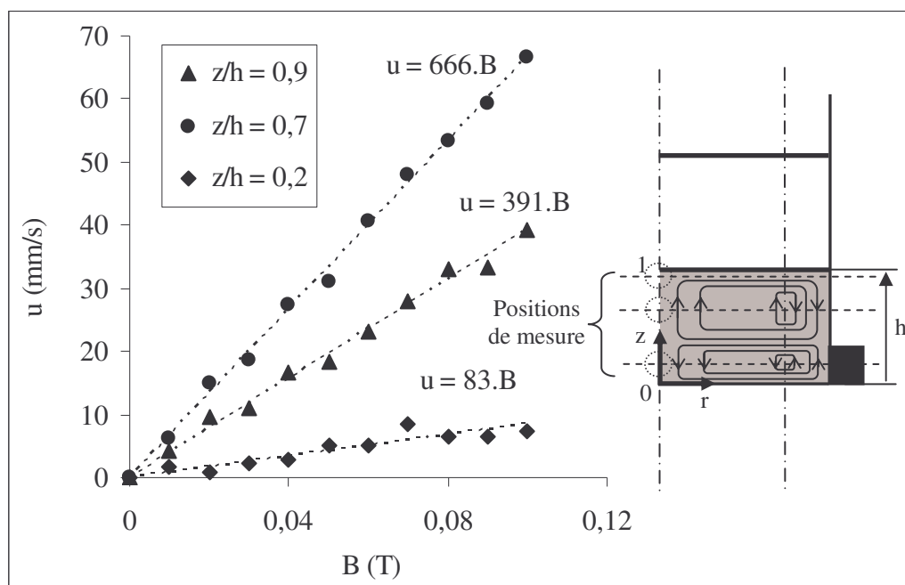
Figure 3.13: Variation des vitesses verticales moyennes locales en fonction de l'intensité du champ magnétique. f = 30 Hz. Les mesures sont réalisées sur l'axe de symétrie de la cuve pour trois points de mesure : z/h = 0,2, 0,7, 0,9 - mesure UDV.
