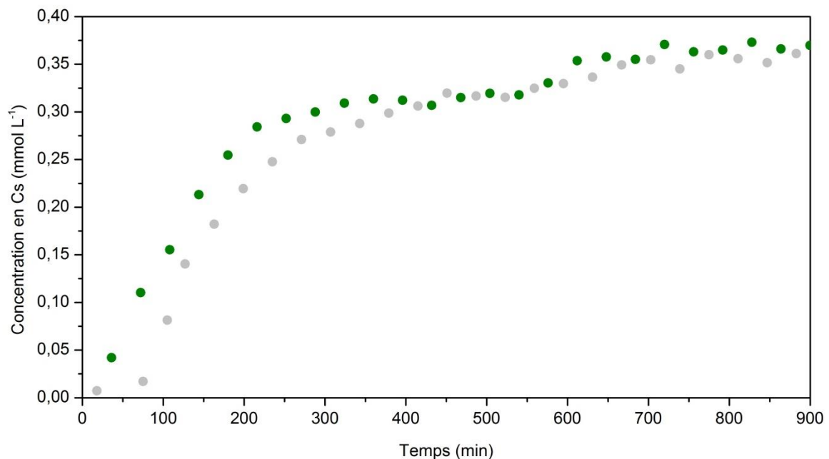
Figure 59 : Courbe de percée du césium (en gris) et du sodium (en vert). Conditions opératoires : T = 25 \text{ °C} ; 5,30 g de Biosorb ; [\text{Cs}^+]_0 et [\text{Na}^+]_0 = 3,76 \times 10^{-4} \text{ mol L}^{-1} ; débit = 1 \text{ mL min}^{-1} ; pH = 5,6.
