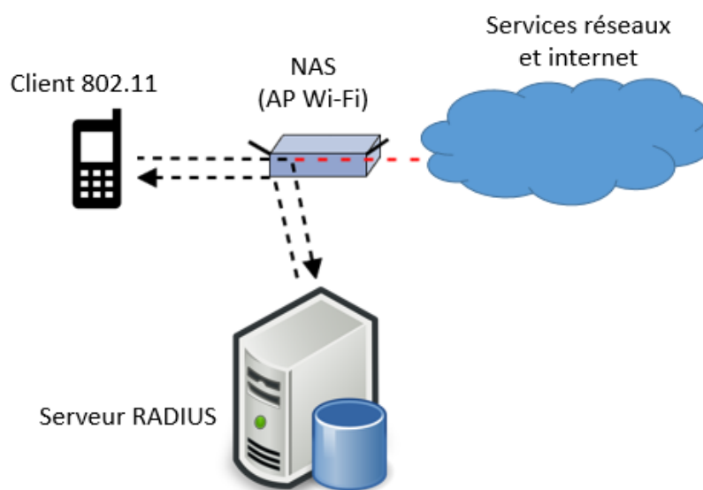
Figure 15 : Authentification avec un serveur RADIUS
