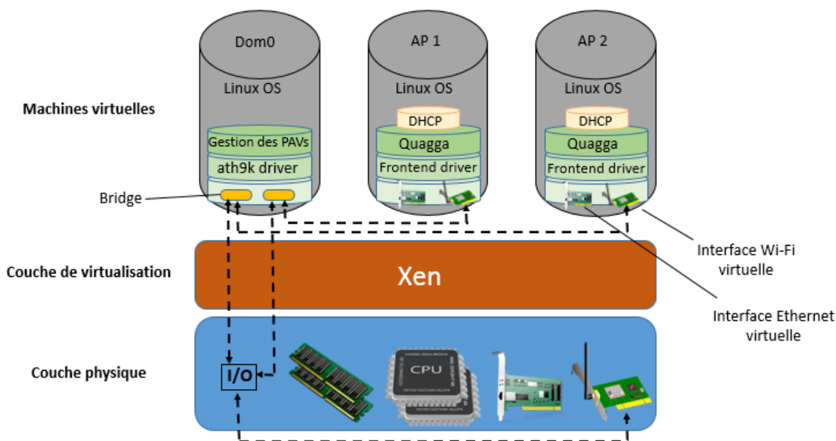
Figure 7: Architecture des points d'accès Wi-Fi virtuels
