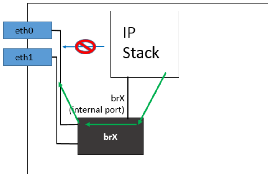
Figure 30 : Interfaces bridgées au bridge OVS
