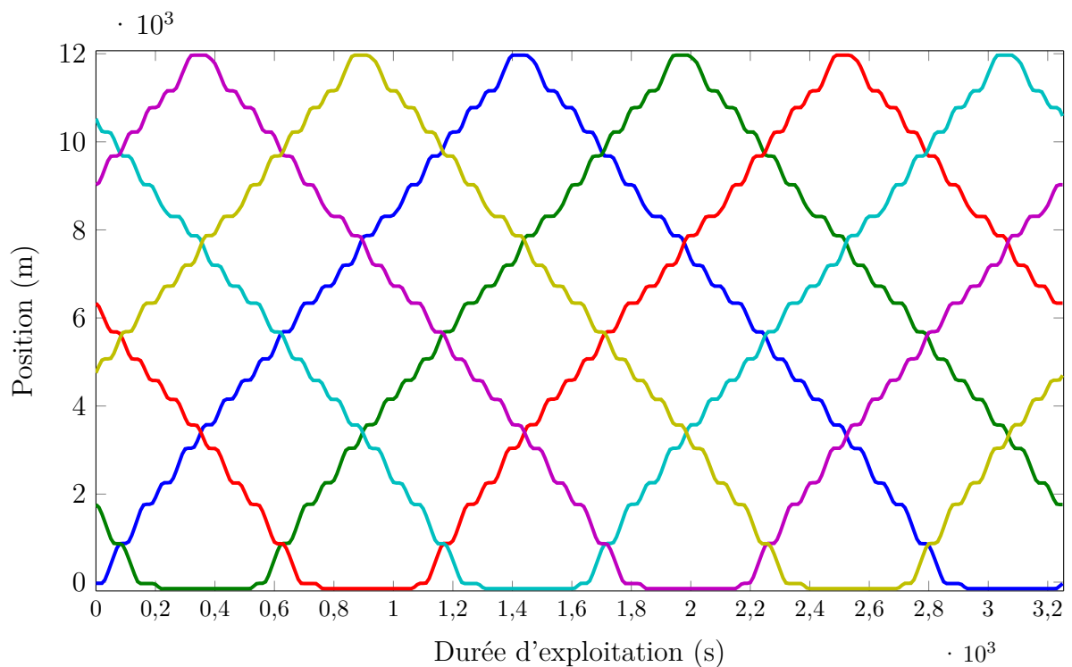
FIGURE 3.2 – Evolution de position d'un train sur un tour de boucle.
