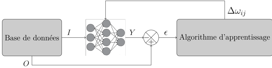
FIGURE 4.8 – Architecture simplifiée de la méthode d'apprentissage supervisé.
