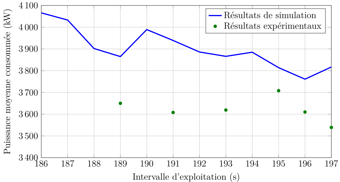
FIGURE 3.9 – Comparaison des résultats de simulation avec des mesures sur le site de Turin pour un carrousel composé de 16 trains
