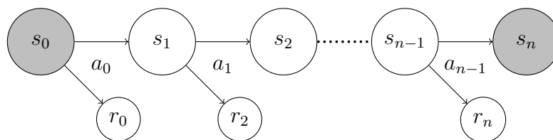
FIGURE 4.17 – Illustration d'un processus de décision markovien.
