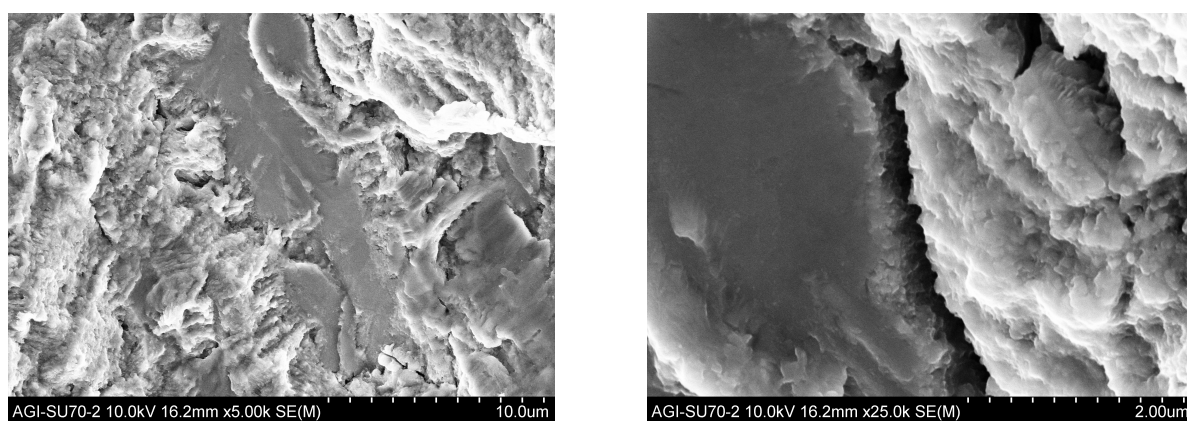
Figure 3.49 : Faciès de rupture obtenue pour le lot 1. La contrainte maximale pour chaque lot est \sigma_{max}^{imp} = 1200 \text{ MPa} et le nombre de cycles avant rupture est 9,22 \cdot 10^5 .
