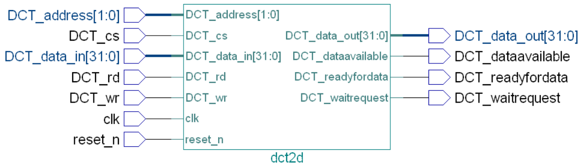
Figure 101. Entité du coprocesseur TCD/TCDI-2D
