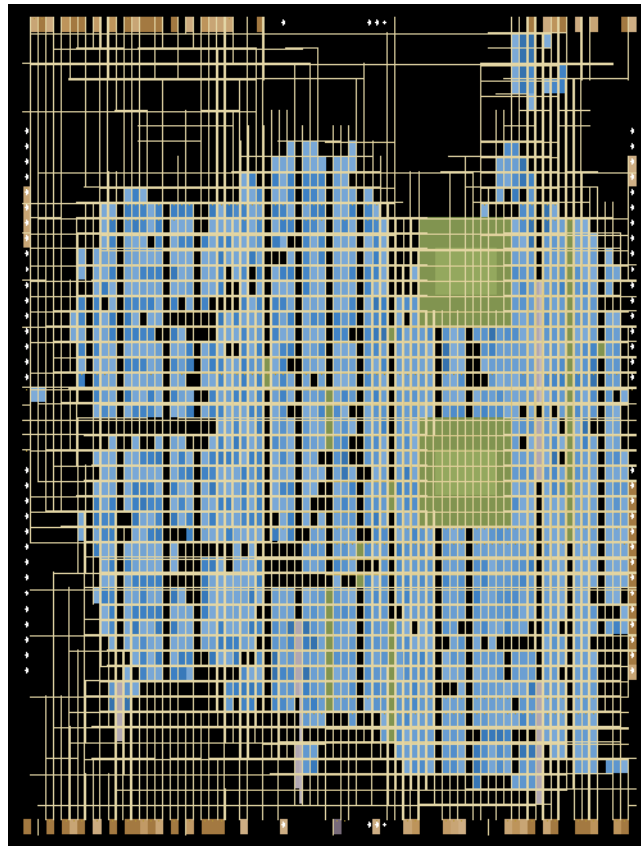
Figure 113. Placement et routage de notre système multimédia sur FPGA Stratix II
