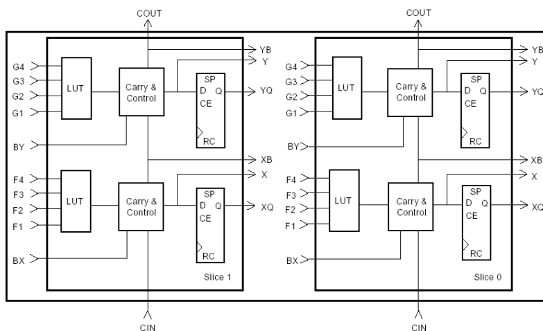
Figure 26. Structure de base d'un composant programmable
