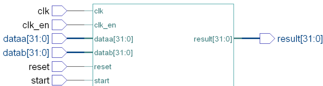
Figure 104. Interface de l'instruction pour Q/QI
