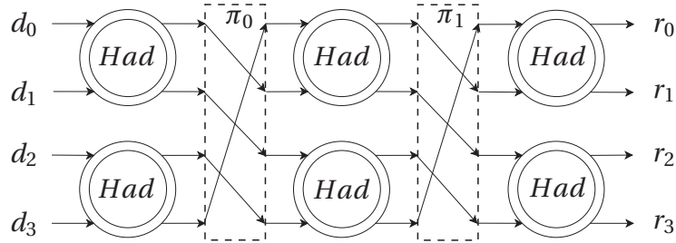
Figure 2.4. Code de Hamming(8,4,4) sous forme Cortex.
