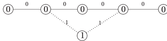
Figure 1.8. Treillis T_1 décrivant le sous-code \langle \mathbf{g}_1 \rangle .
