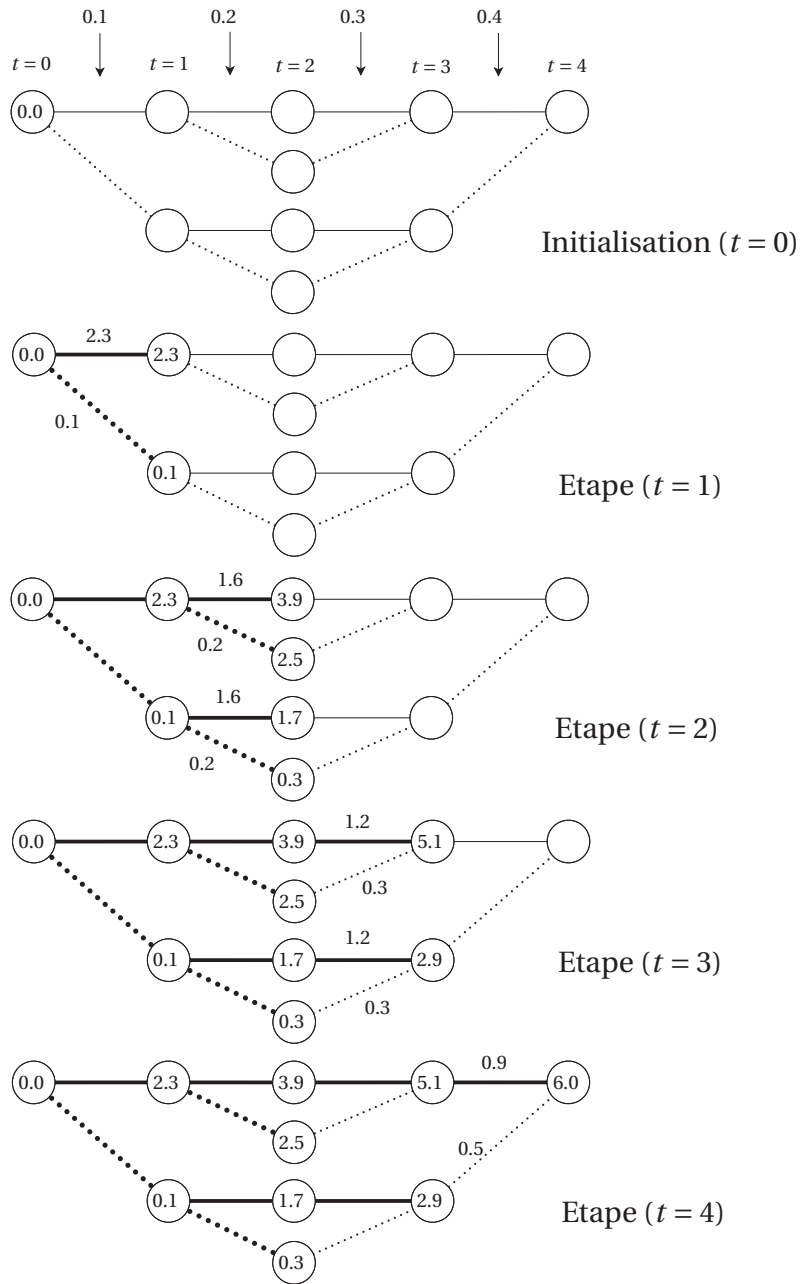
Figure 1.12. Exemple d'algorithme de Viterbi developp pour le code (4,2).
