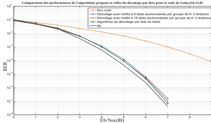
Figure 4.31. Comparaison de performances de l'algorithme proposé avec les deux configurations de dcodage ( n_L = 3, n_S = 6 ) et ( n_L = 4, n_S = 6 ) et celles du dcodage par liste [74] pour le code de Golay(24, 12, 8).
