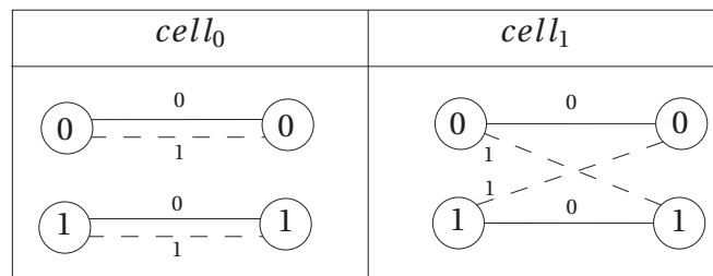
Figure 3.1. Structure des cellules cell_0 et cell_1
