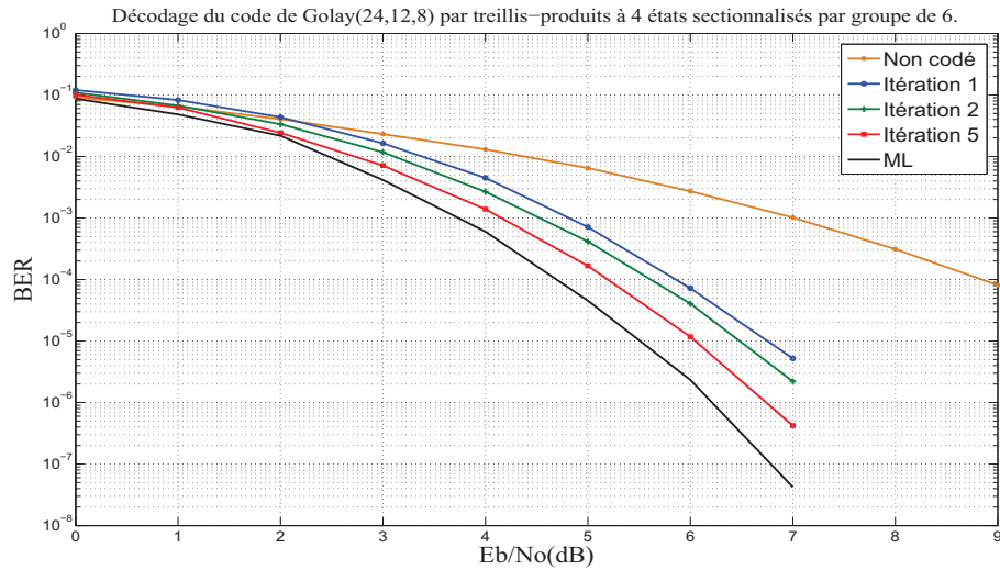
Figure 4.27. Performance de l'algorithme de décodage avec des treillis-produits à 4 états sectionnalisés par groupe de 6 pour le code de Golay(24, 12, 8).
