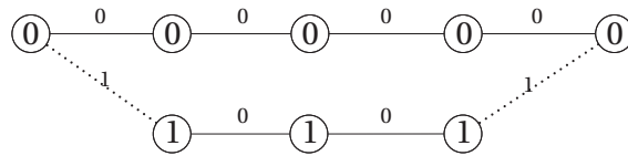
Figure 1.7. Treillis T_0 décrivant le sous-code \langle \mathbf{g}_0 \rangle .
