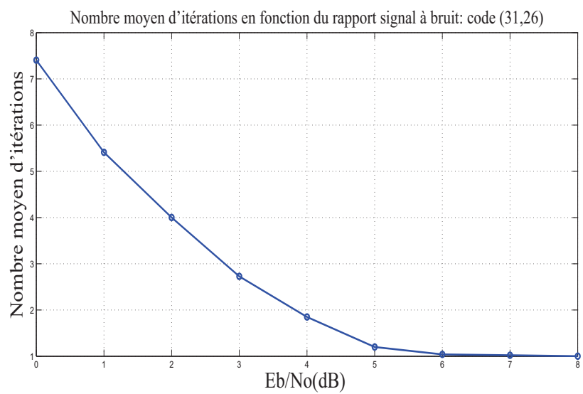
Figure 4.6. Nombre moyen d'itérations en fonction du SNR pour le code (31,26,3).
