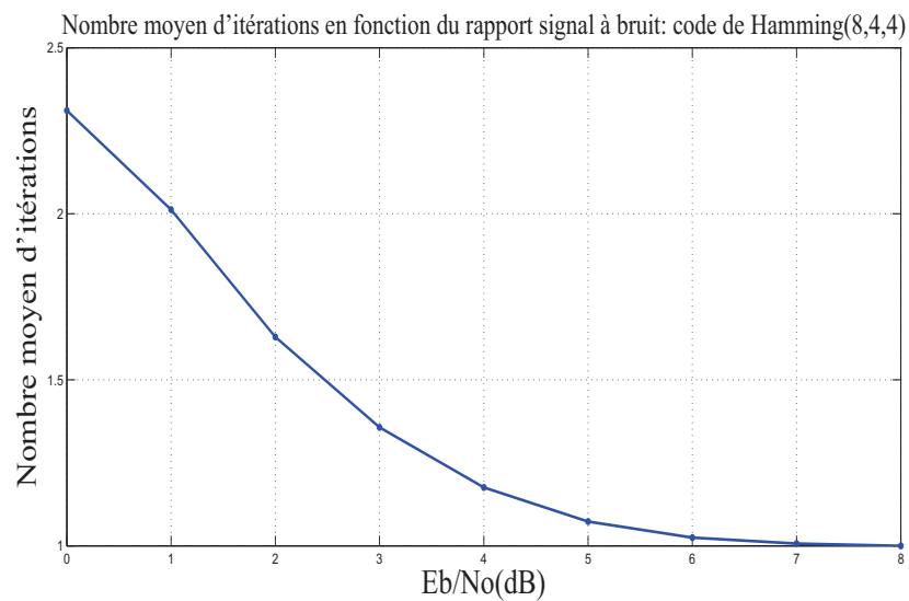
Figure 4.5. Nombre moyen d'itérations en fonction du SNR pour le code de Hamming(8,4,4).
