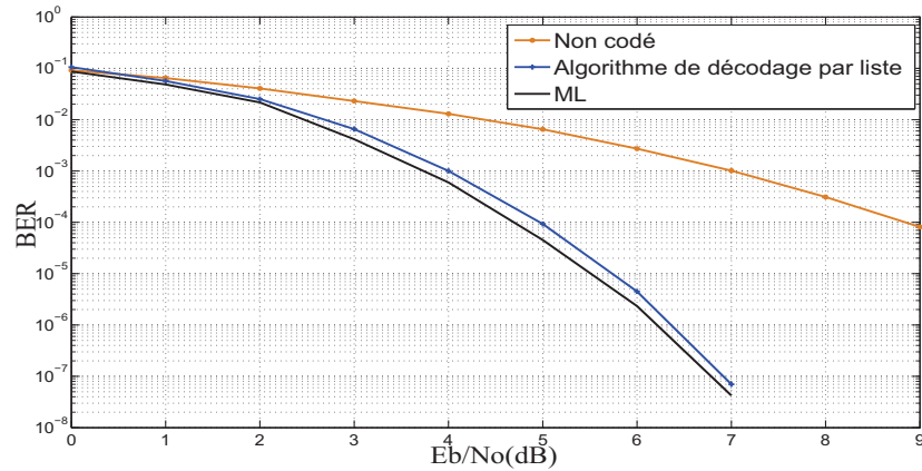
Figure 2.9. Performances de l'algorithme de décodage par liste.
