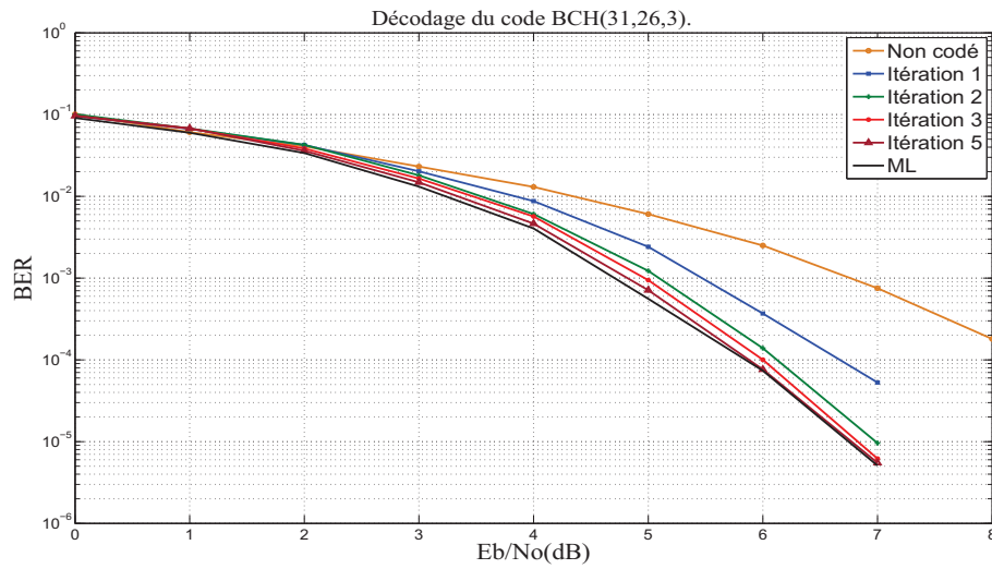
Figure 4.3. Performances de l'algorithme de décodage itératif driv de List-Viterbi pour le code (31,26,3).
