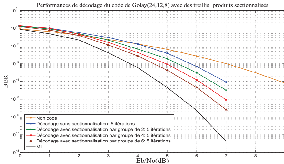
Figure 4.24. Performances de l'algorithme de dcodage avec des treillis-produits sectionnaliss pour le code de Golay(24,12,8).
