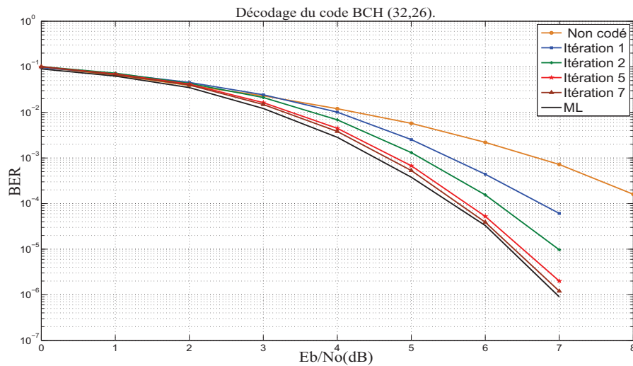
Figure 4.4. Performances de l'algorithme de décodage itératif driv de List-Viterbi pour le code (32,26,4).
