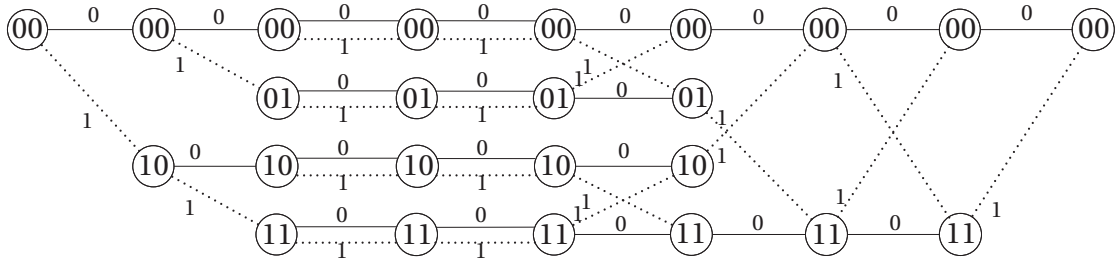
Figure 3.4. Treillis-produit T_0 \otimes T_1 .
