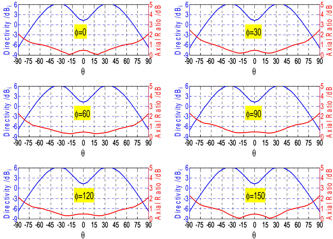
Figure III-14 : La directivité (bleu) et le taux d'ellipticité (rouge) synthétisés dans les plans \{\phi=0^\circ, 30^\circ, 60^\circ, 90^\circ, 120^\circ, 150^\circ\} pour la fréquence 8.2 GHz
