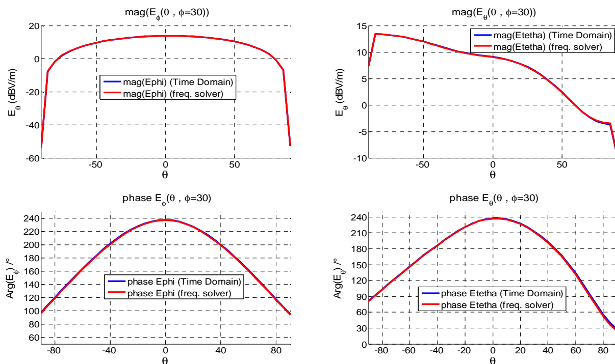
Figure A- 17: Comparaison de diagramme de rayonnements pour un maillage adaptative par solveur fréquentiel et le maillage définit en transitoire
