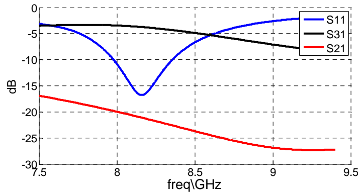
Figure III-41 : Paramètre[S] du patch sur chaque ligne d'excitation
