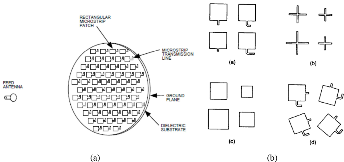
Figure I-27 : Panneau réflecteur d'une antenne de type reflectarray intégrant des charges réactives représentées par des Stubs en circuit-ouvert (a). Exemples de charges réactives pour la synthèse de phase par des modifications géométriques des motifs du panneau (b) [64].
