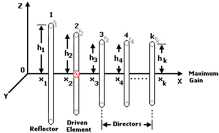
Figure I-2 : Illustration d'une antenne à éléments parasites (YAGI_UDA)
