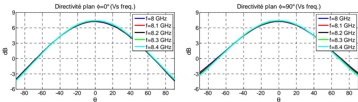
Figure A-4: Diagrammes de directivité de l'antenne dans les plans \Phi=0^\circ et \Phi=90^\circ sur la bande couvrant 8GHz à 8.4GHz.
