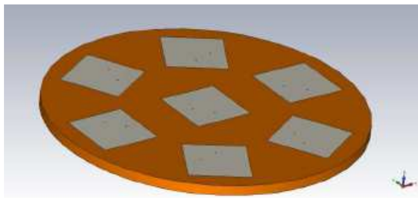
Figure A- 1: réseau patch de 7 éléments
