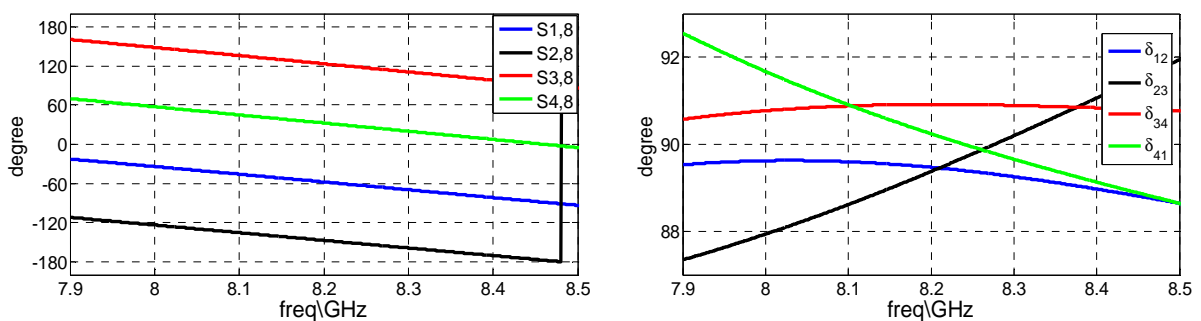
Figure IV-8 : Phases calculées à l'entrée de chaque ligne d'alimentation du patch. A droite les écarts de phase entre les lignes font apparaître une erreur inférieure à 3^\circ sur toute la bande
