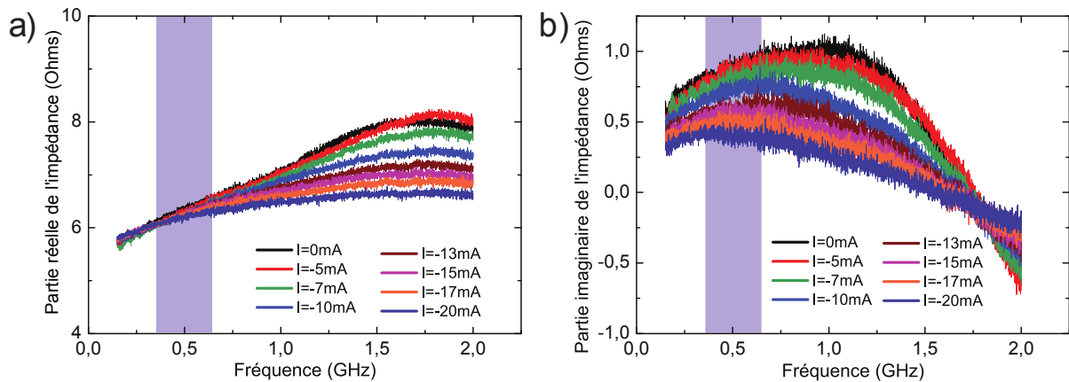
Figure II.13 – Partie réelle et imaginaire de l'impédance des échantillons mesurée avec un VNA. La zone bleue indique la plage de fréquence dans laquelle nous travaillerons principalement (autour de la fréquence naturelle de l'oscillateur à vortex).
