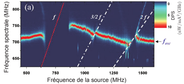
Figure III.10 – Adapté de [67]. Expérience réalisée sur un oscillateur à vortex nanopilier. Carte couleur de spectre en fonction de la fréquence de l'onde RF injectée. On peut voir 3 plages de synchronisation pour une fréquence de modulation proche de f_0 de 3/2f_0 et de 2f_0
