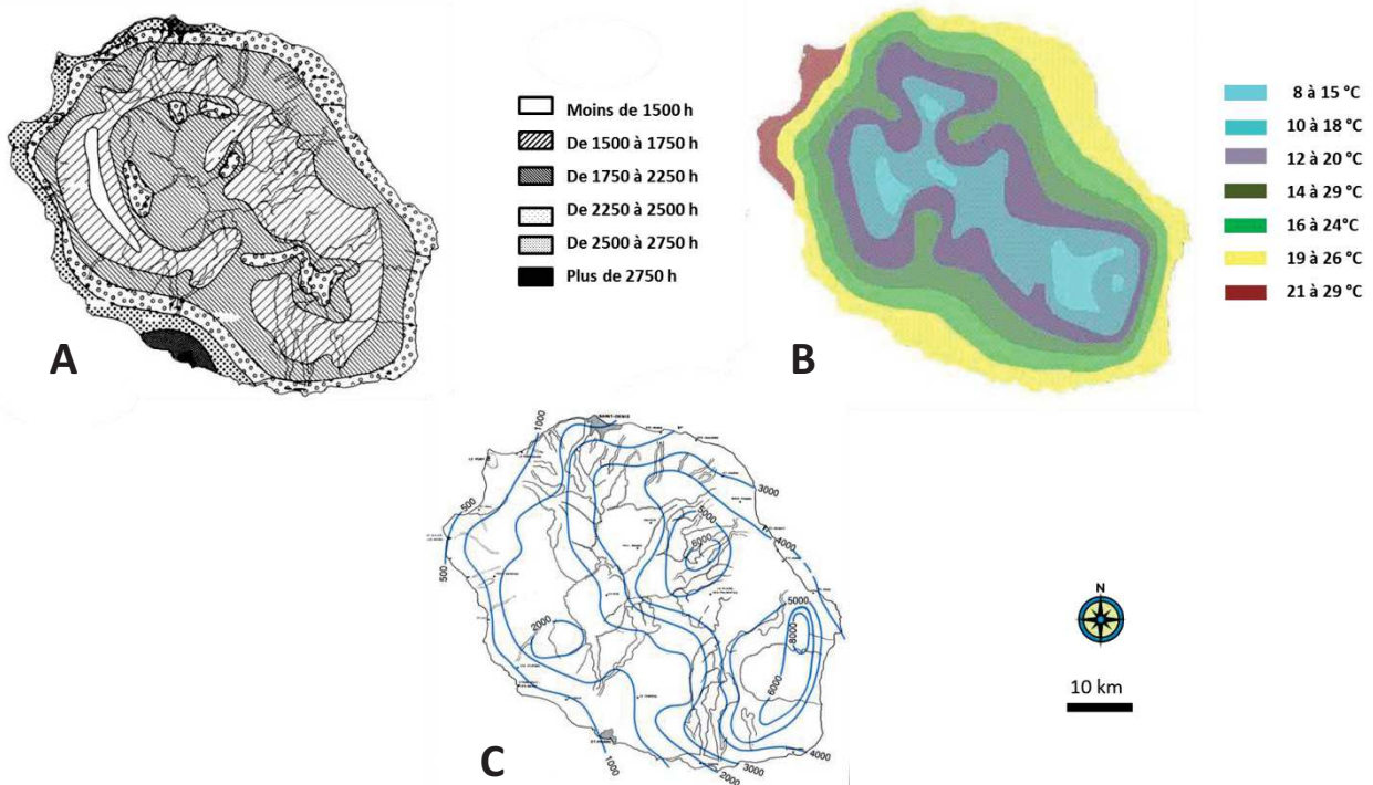
Figure I. 2. Cartes représentant (A) l'ensoleillement annuel moyen, (B) le gradient thermique annuel moyen, et (C) le gradient pluviométrique annuel moyen à la Réunion, adapté de Raunet (1991).
